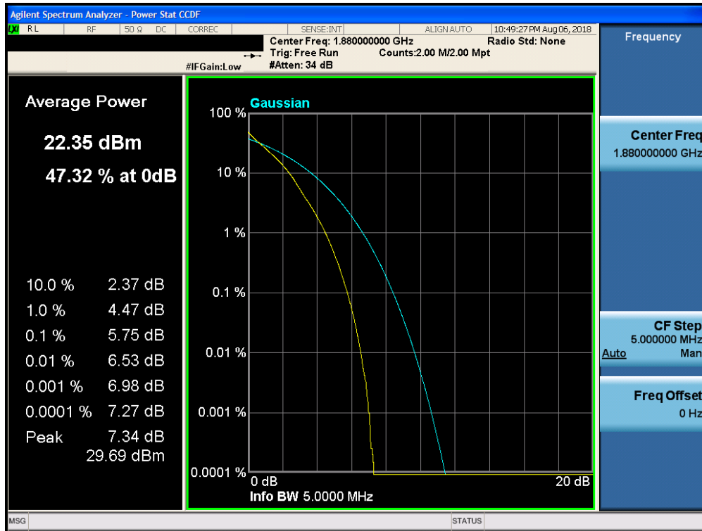
Plot 7-306. PAR Plot (Band 2 - 5.0MHz QPSK - Full RB Configuration)
