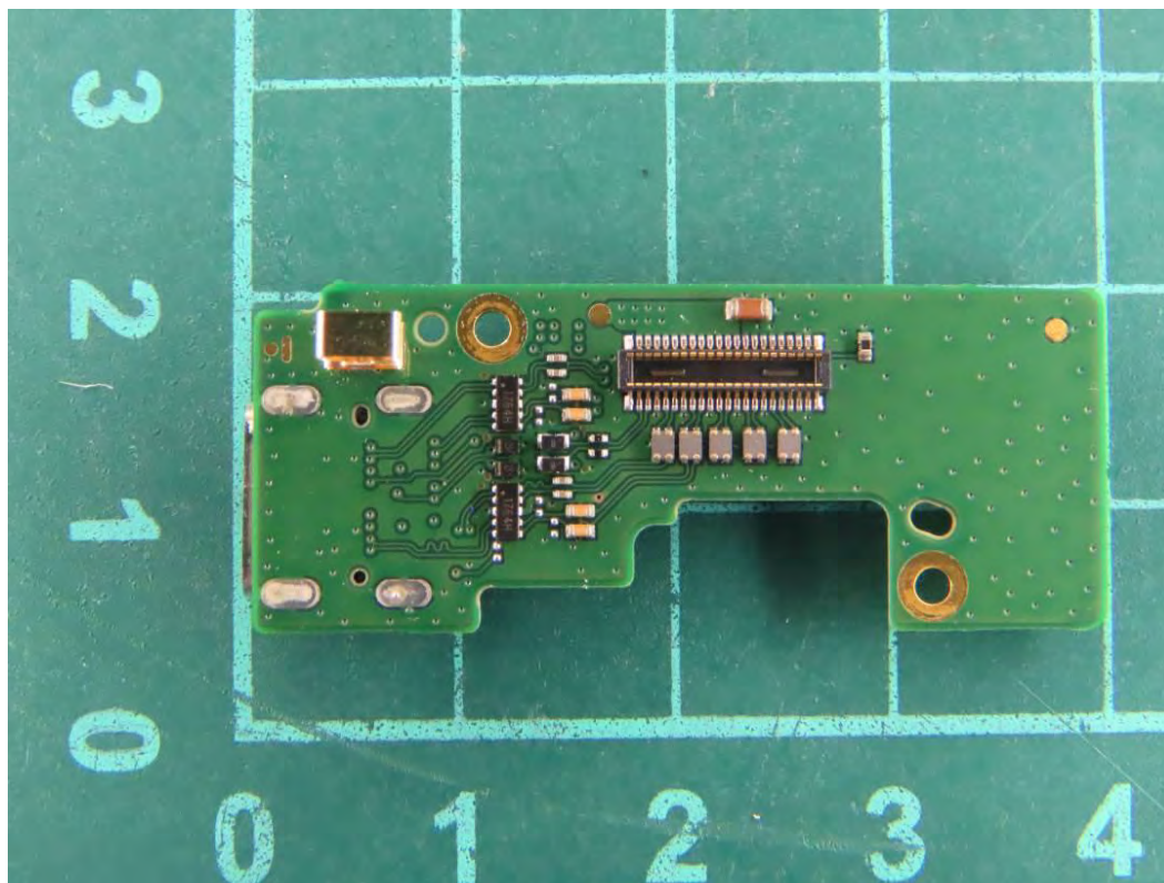
(44) EUT Photo
