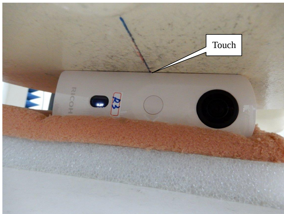
EUT Left-Side
