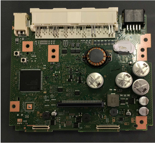
【Indicator Board】
