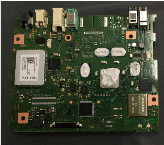
【CPU Board】
