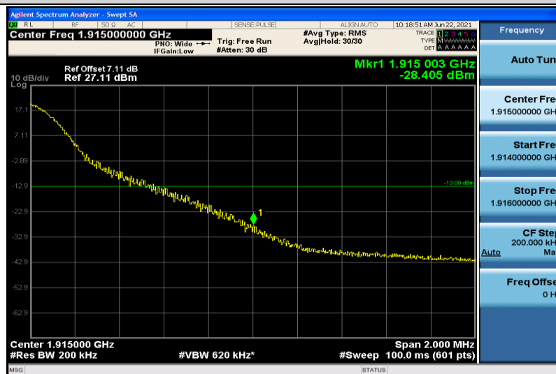
Band25-20MHz-16QAM-26590-1RB#99
