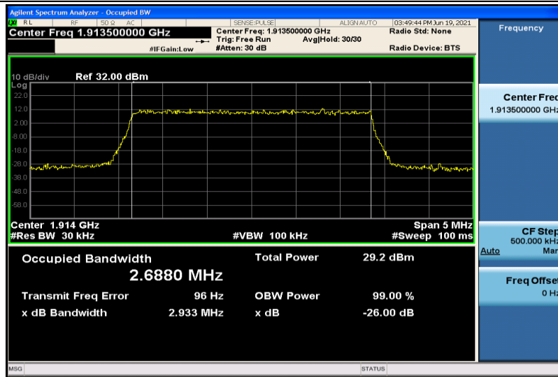
Band25-3MHz-QPSK-26675-15RB#0-2.6880
