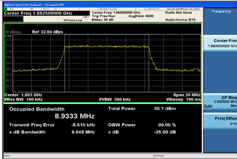
Band25-10MHz-QPSK-26365-50RB#0-8.9333
