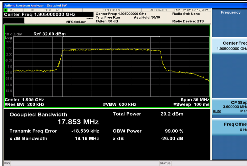
Band25-20MHz-QPSK-26590-100RB#0-17.853
