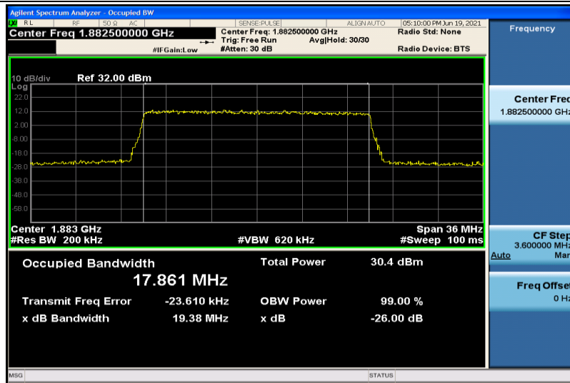
Band25-20MHz-QPSK-26365-100RB#0-17.861
