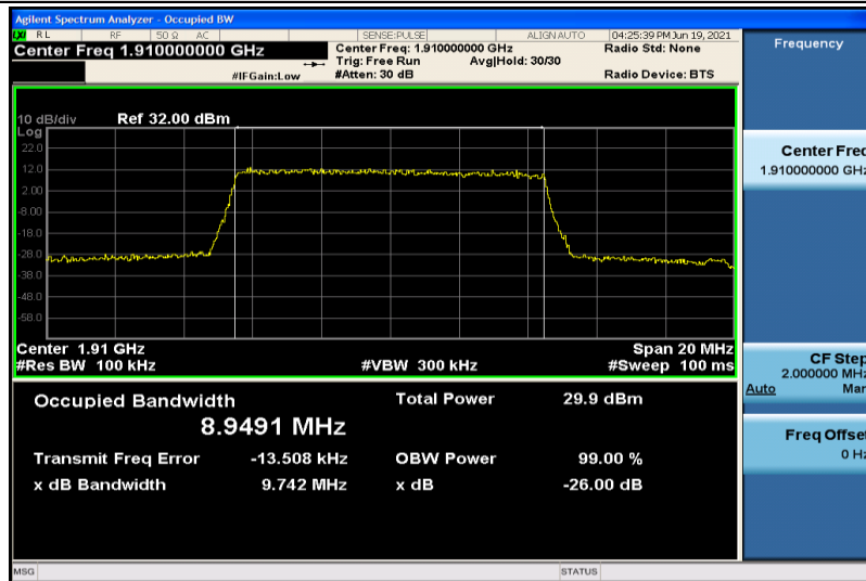
Band25-10MHz-QPSK-26640-50RB#0-8.9491
