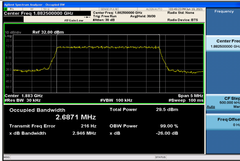
Band25-3MHz-QPSK-26365-15RB#0-2.6871
