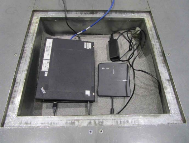
AE(Below 1 GHz)
