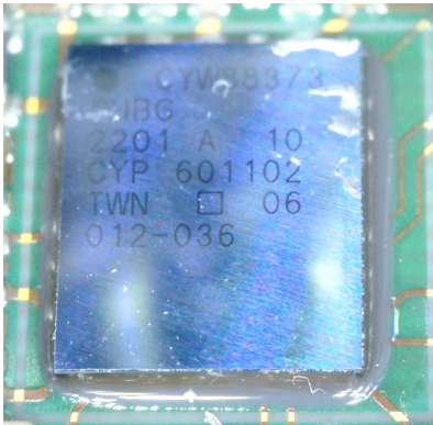
BT/WLAN Chip(CYW88373) ※Remove heat dissipation sheet
