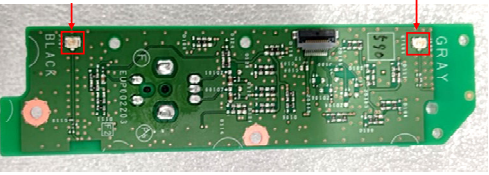
SW PCB F2 side
