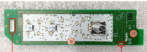
SW PCB F1 side
