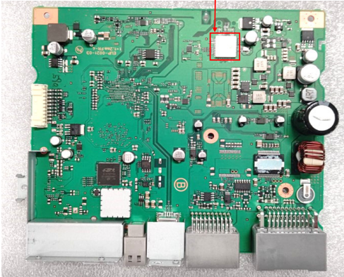
Main PCB F1 side
