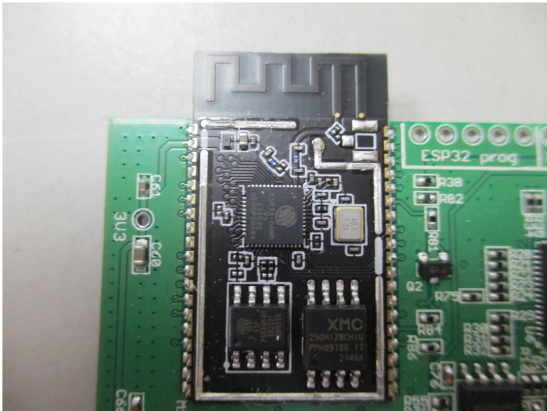
Wi-Fi & BLE Chain 1 IC
