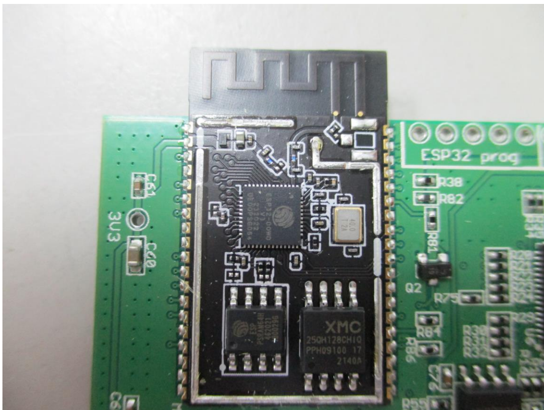
Wi-Fi &amp; BLE Chain 0
