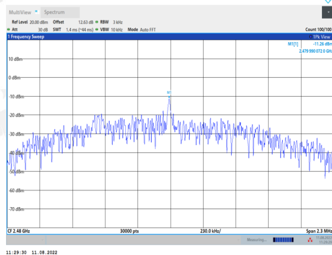
BLE_2M_Ant1_2480
