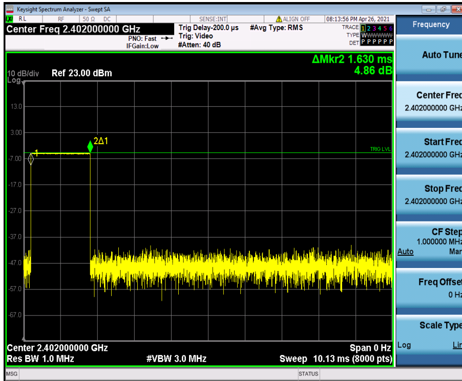
DH3_Ant1_Hop_2402
