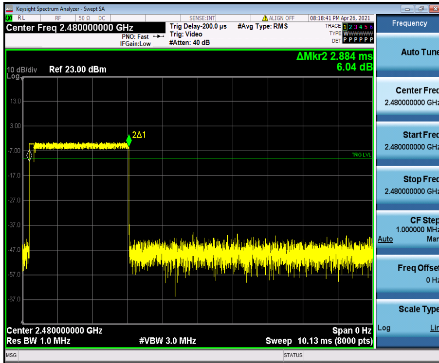
2DH5_Ant1_Hop_2480
