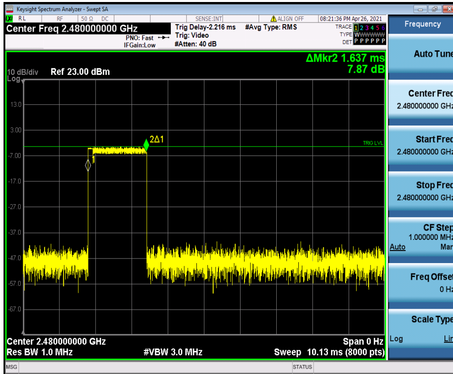
2DH3_Ant1_Hop_2480
