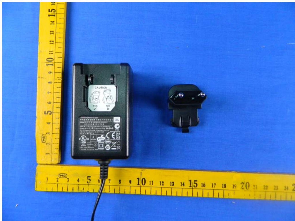
18) EUT Photo(Adapter 2#)
