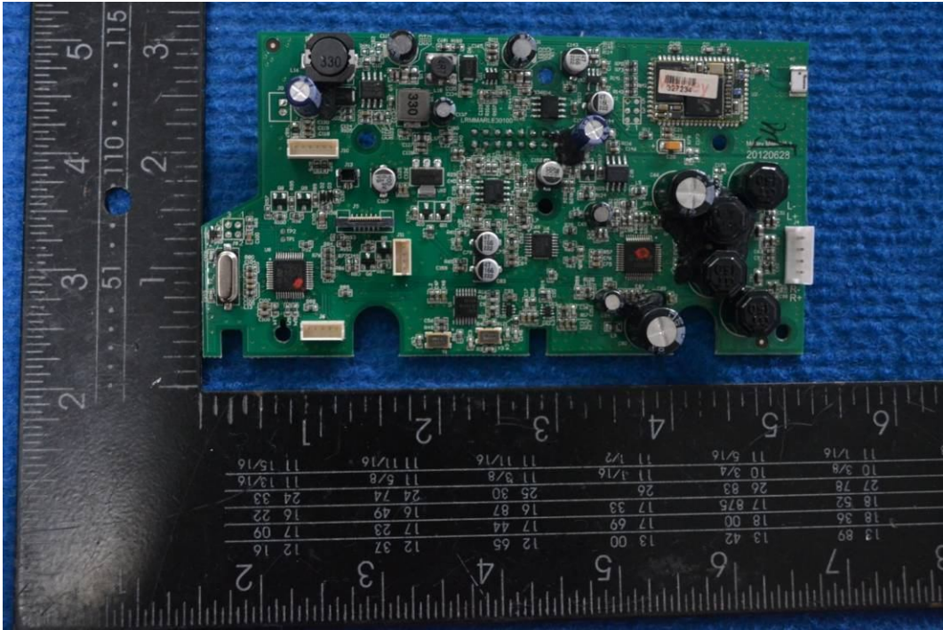
Bluetooth module
