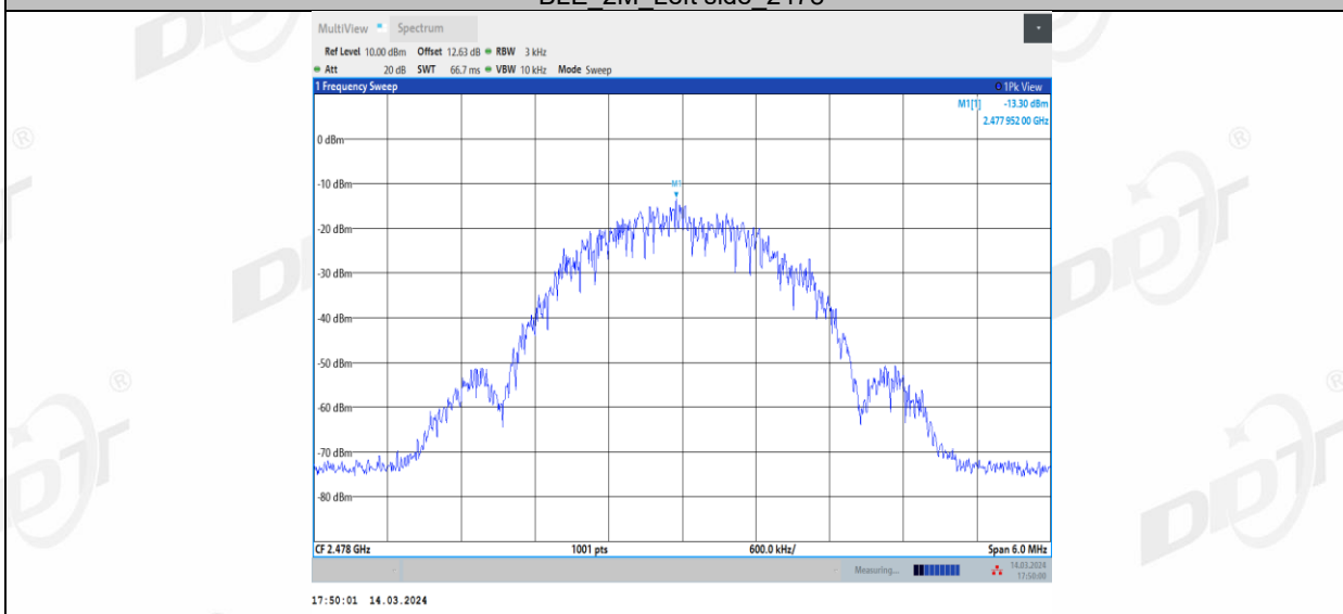
BLE_2M_Left side_2478
