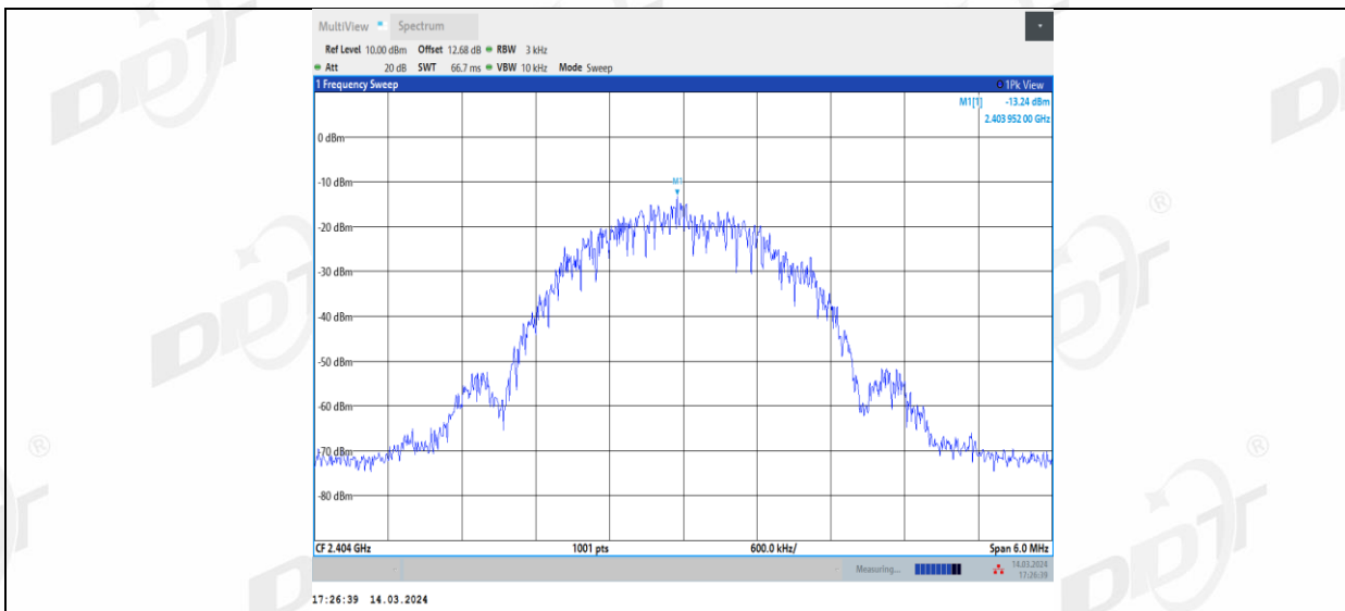
BLE_2M_Left side_2404
