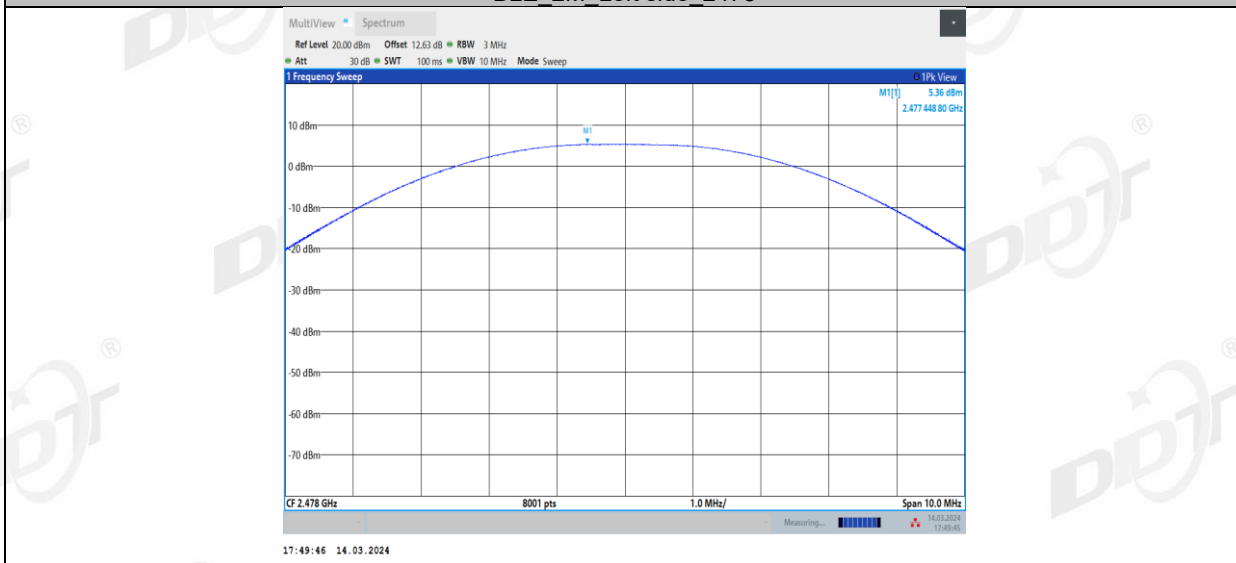
BLE_2M_Left side_2478
