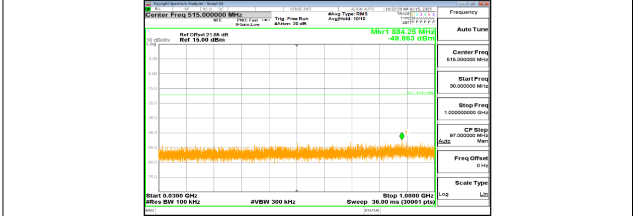
BLE 2M Ant1 2478 30~1000
