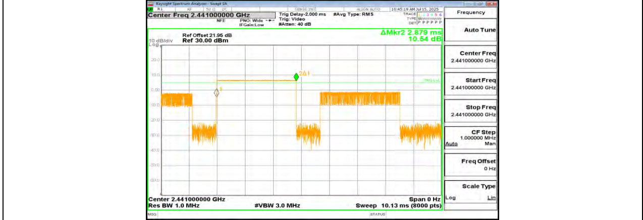
DH5_Ant1_Hop
