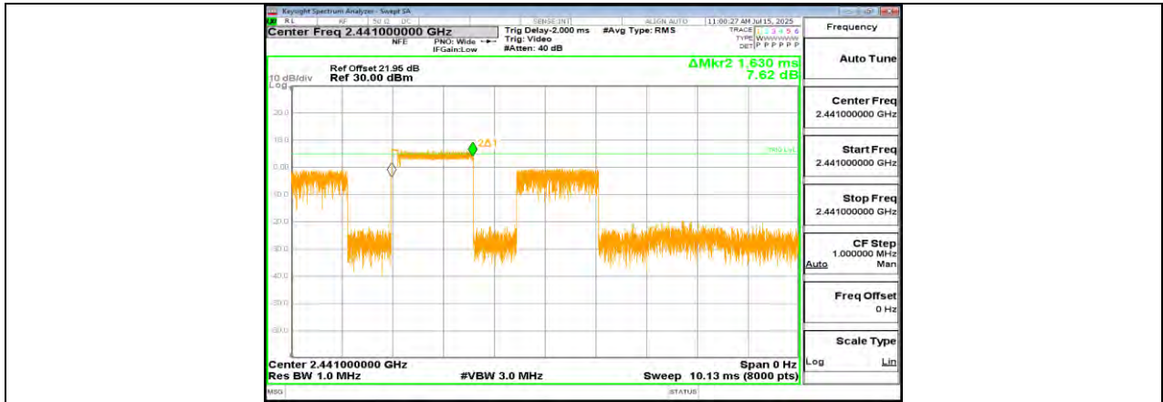
3DH3_Ant1_Hop
