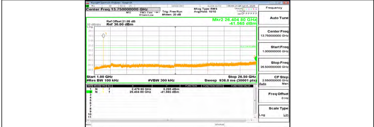
DH5_Ant1_2480_1000-26500
