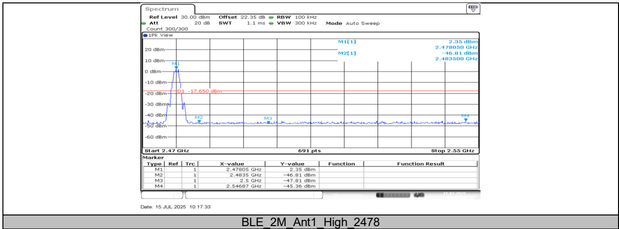
BLE 2M_Ant1_High_2478
