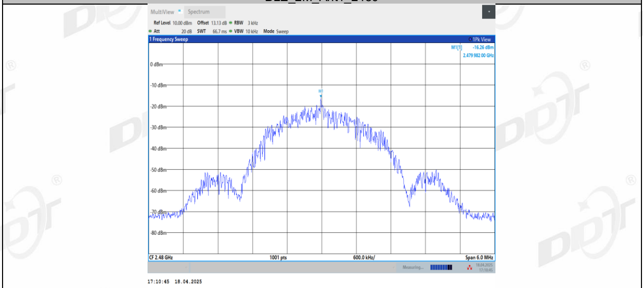
BLE_2M_Ant1_2480
