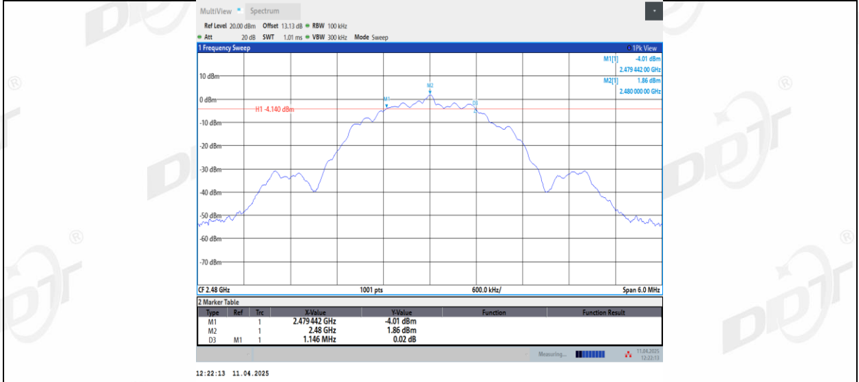
BLE_2M_Ant1_2480
