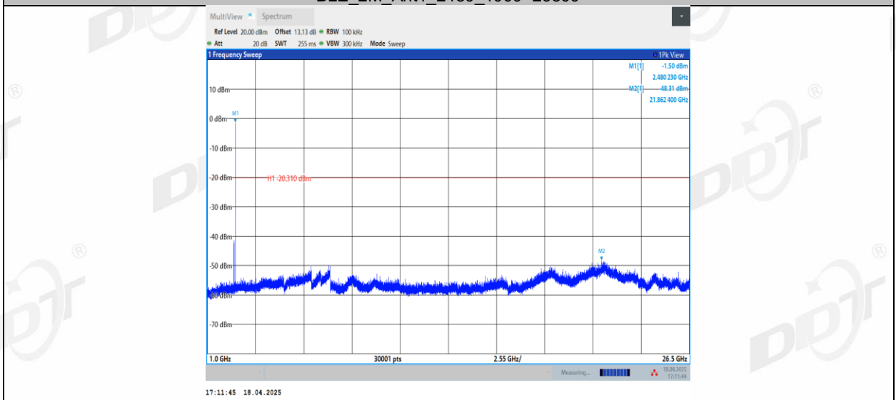
BLE_2M_Ant1_2480_1000~26500
