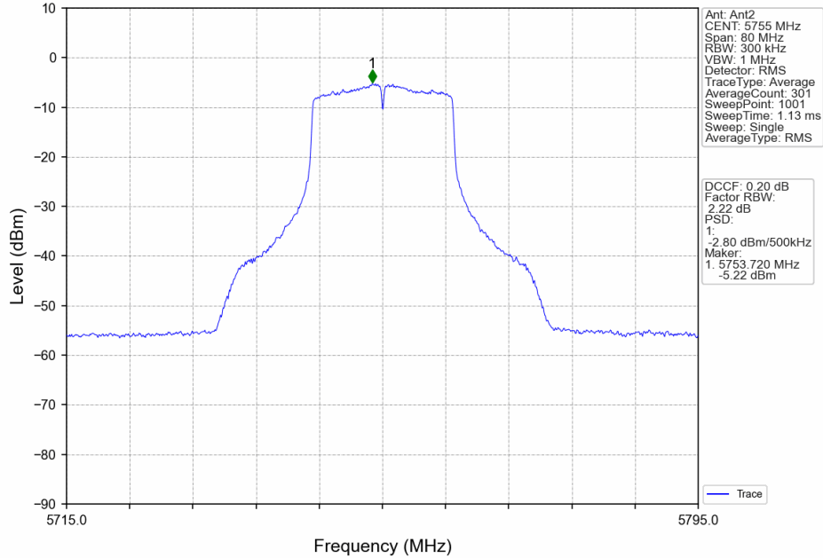
802.11ac(VHT40)_LCH_5755MHz_MIMO_NTNV
