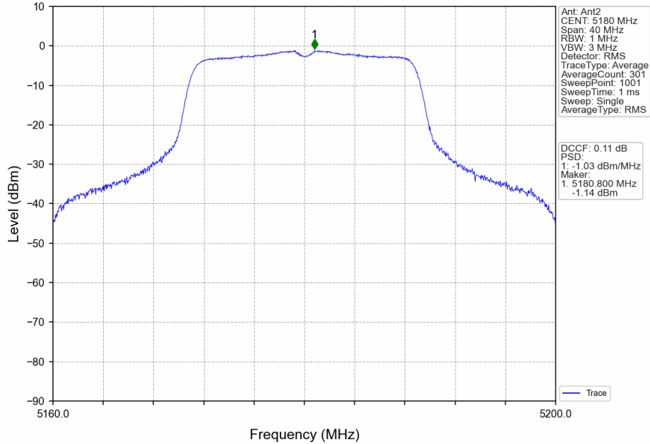
802.11n(HT20)_LCH_5180MHz_MIMO_NTNV
