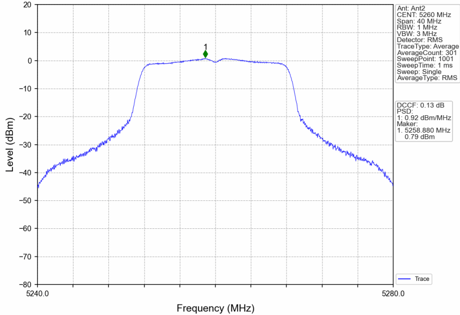
802.11a_LCH_5260MHz_MIMO_NTNV
