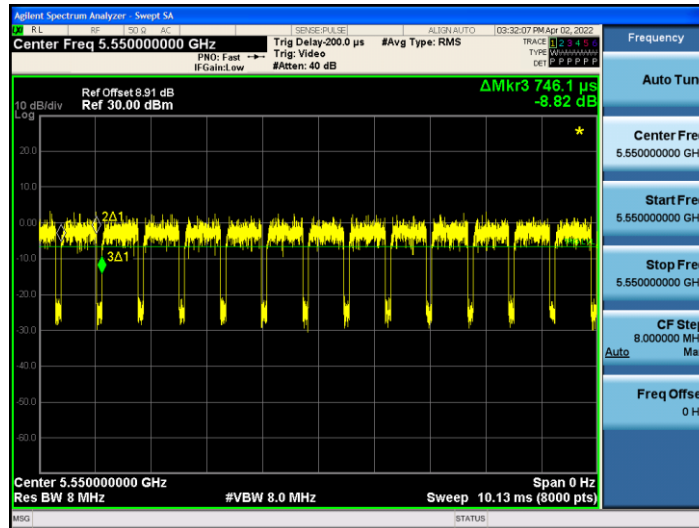
11N40MIMO_Ant2_5550
