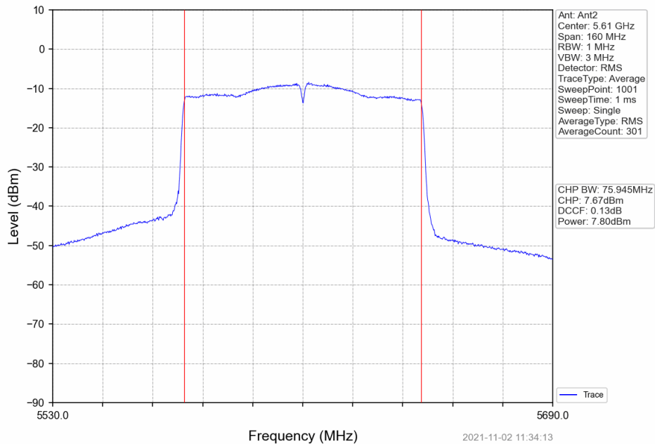
802.11ac(VHT80)_HCH_5610MHz_Ant2_NTNV
