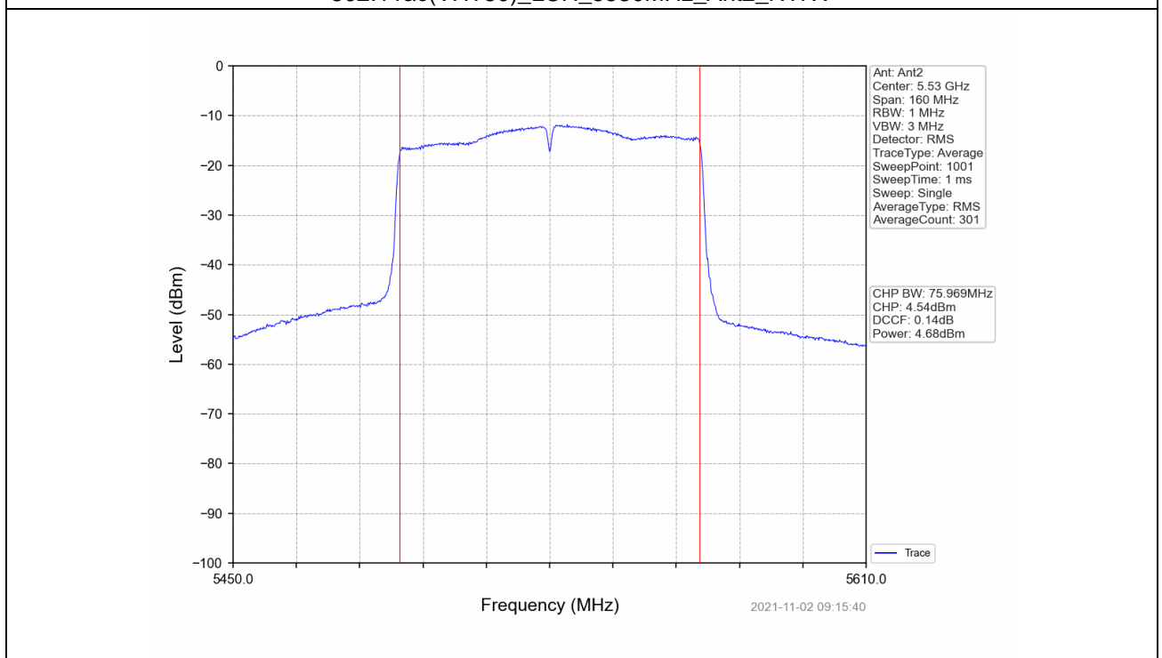
802.11ac(VHT80)_LCH_5530MHz_Ant2_NTNV
