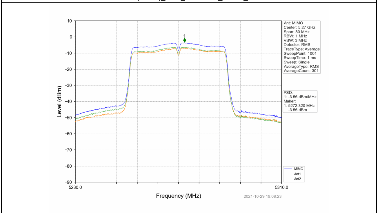
802.11n(HT40)_LCH_5270MHz_MIMO_NTNV
