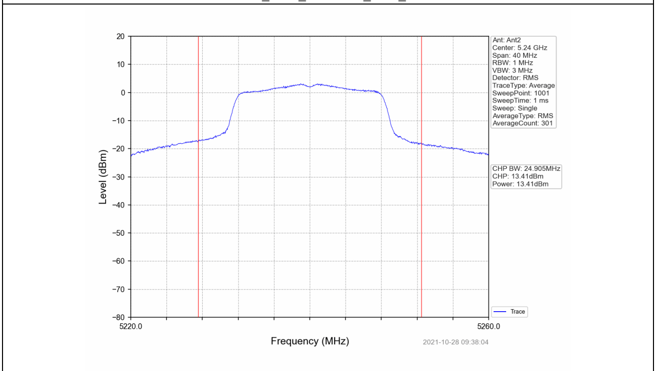
802.11a_HCH_5240MHz_Ant2_NTNV
