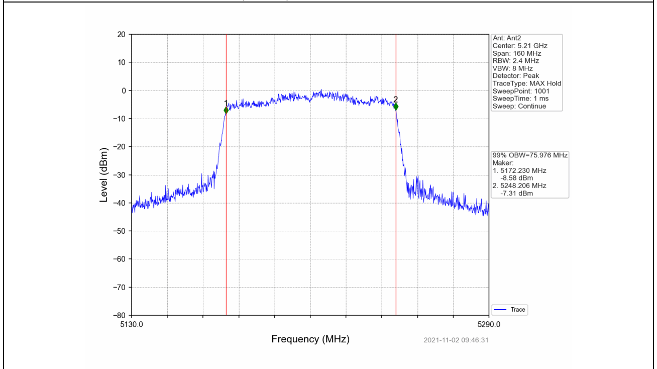
802.11ac(VHT80)_MCH_5210MHz_Ant2_NTNV
