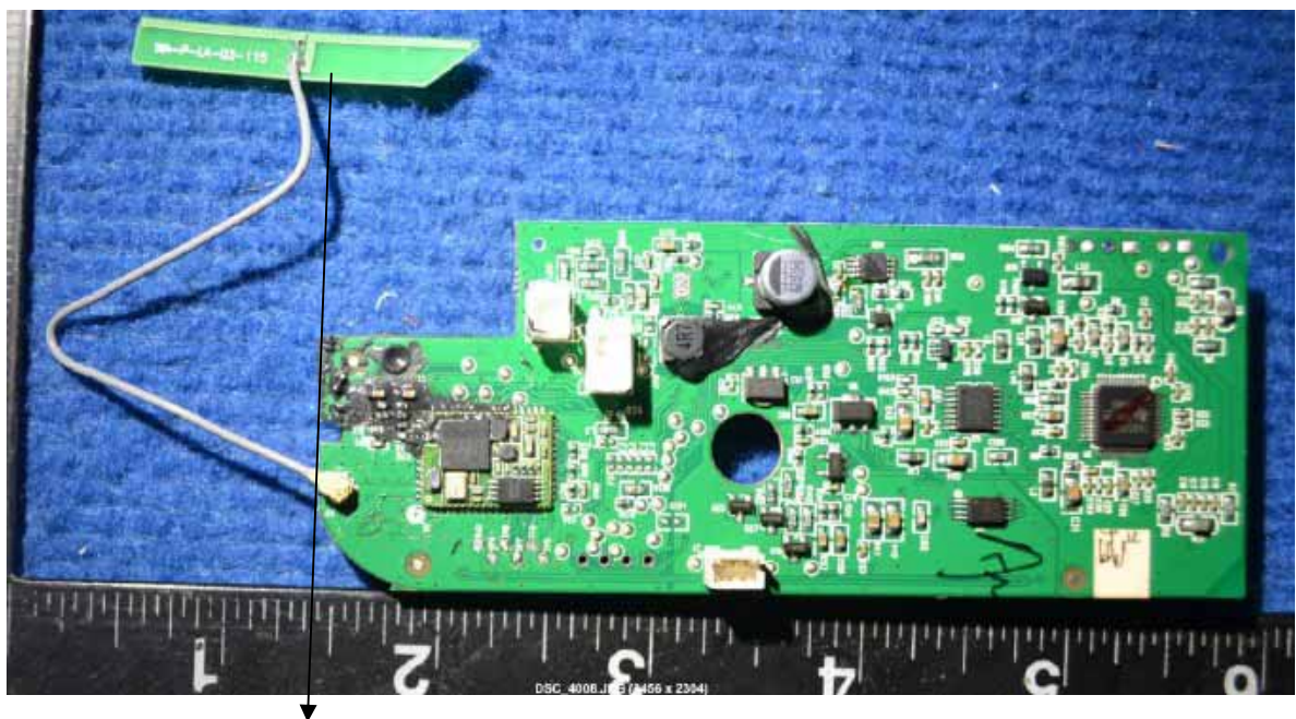
Antenna
