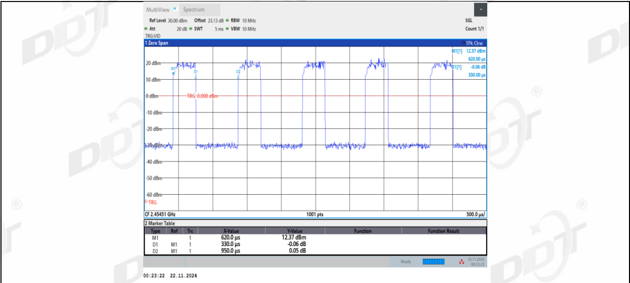
11AX20MIMO Ant2_2462_52Tone_RU38
