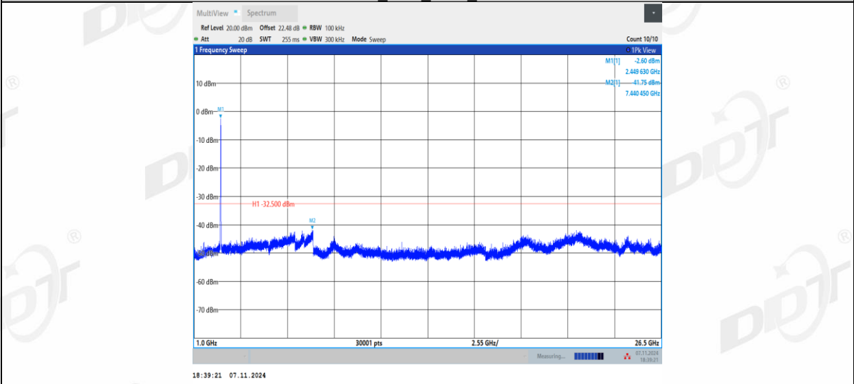
11AX20MIMO_Ant1_2412_0~Reference
