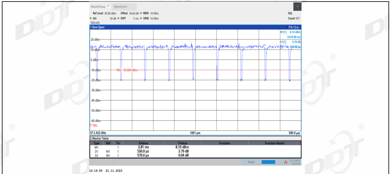
11AX40MIMO_Ant2_2422
