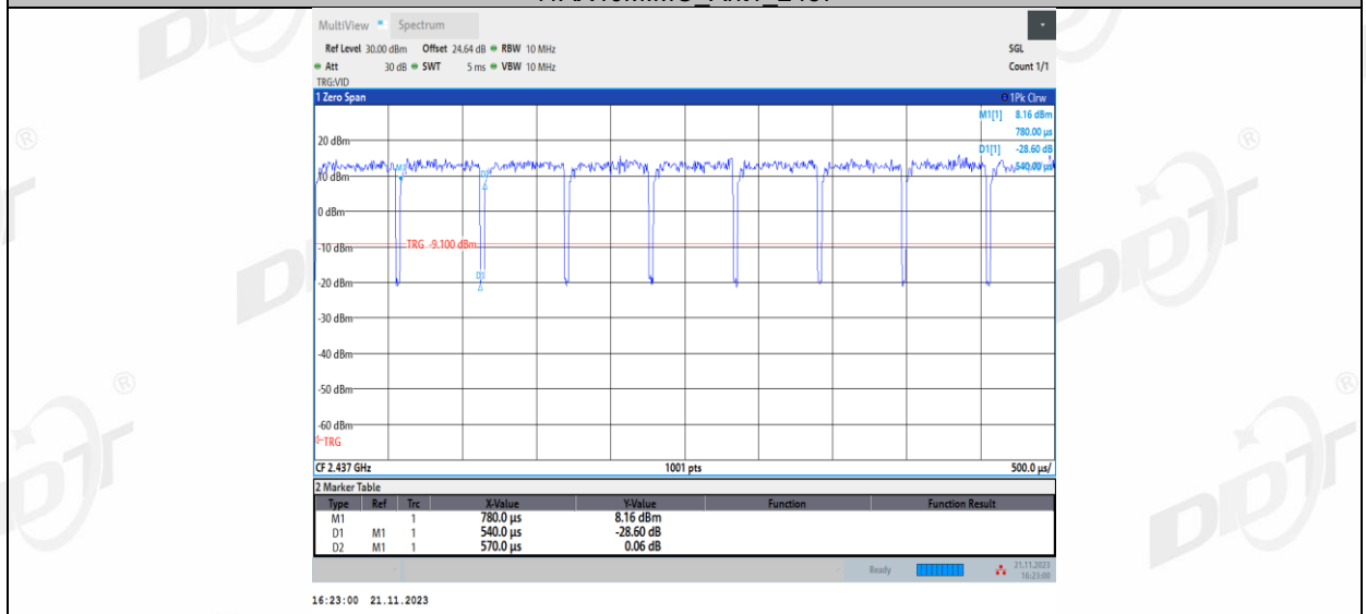
11AX40MIMO_Ant2_2437
