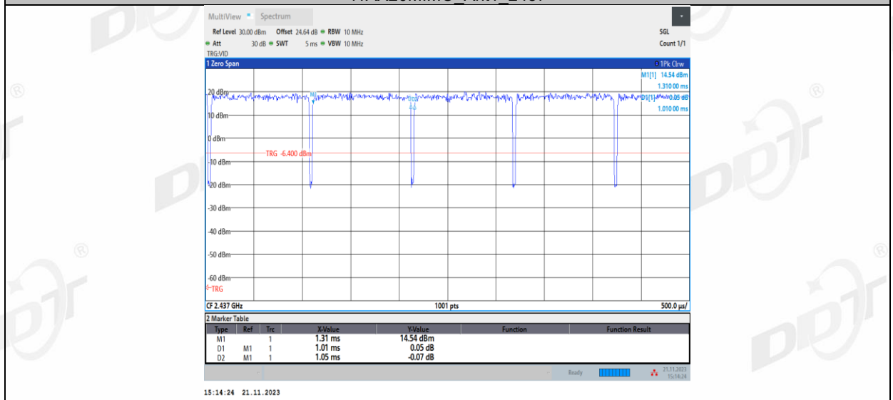
11AX20MIMO_Ant2_2437
