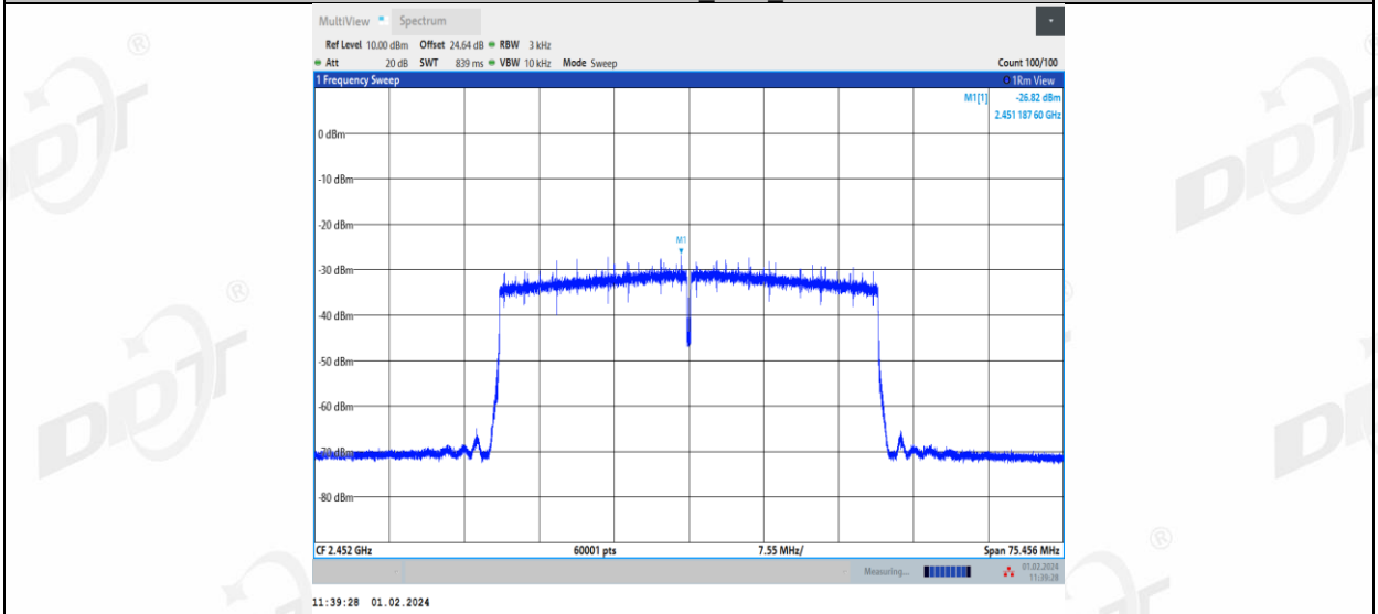
11AX40MIMO_Ant2_2452
