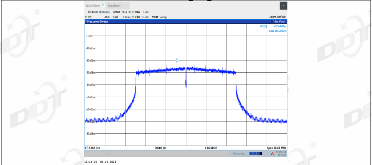
11AX20MIMO_Ant2_2462
