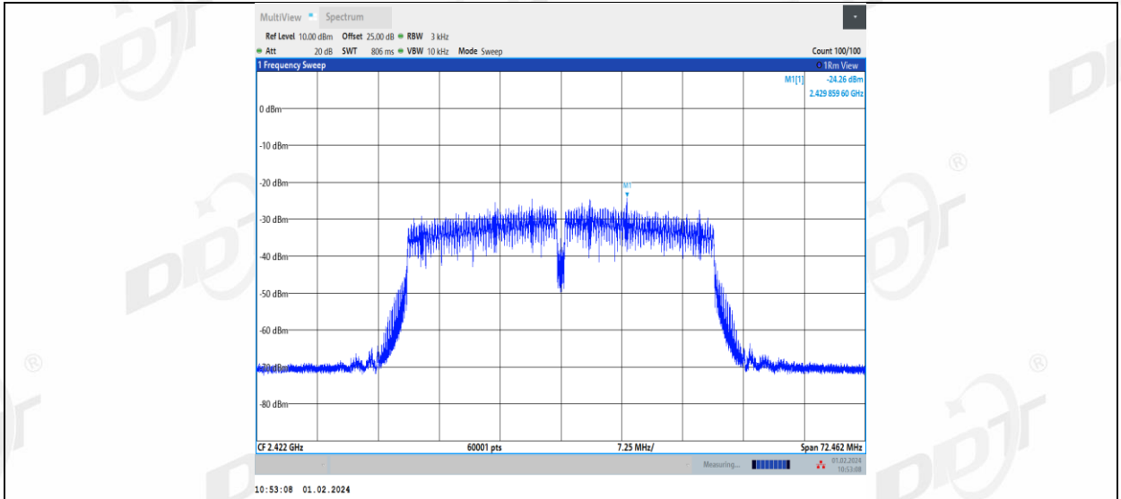
11N40MIMO_Ant2_2422
