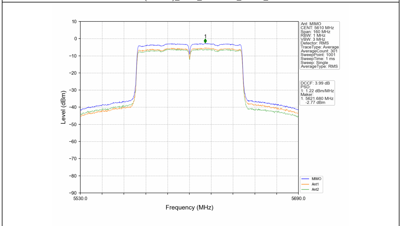
802.11ac(VHT80)_HCH_5610MHz_MIMO_NTNV
