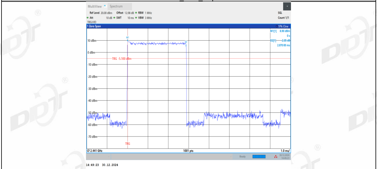
3DH5_Ant1_Hop
