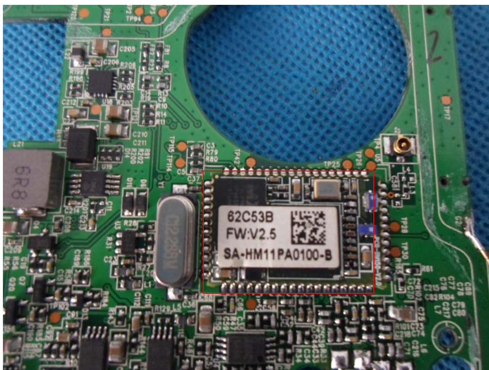
Photo 11 BT module
