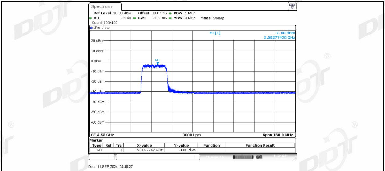
11AX80MIMO_Ant1_5530_242Tone_RU64
