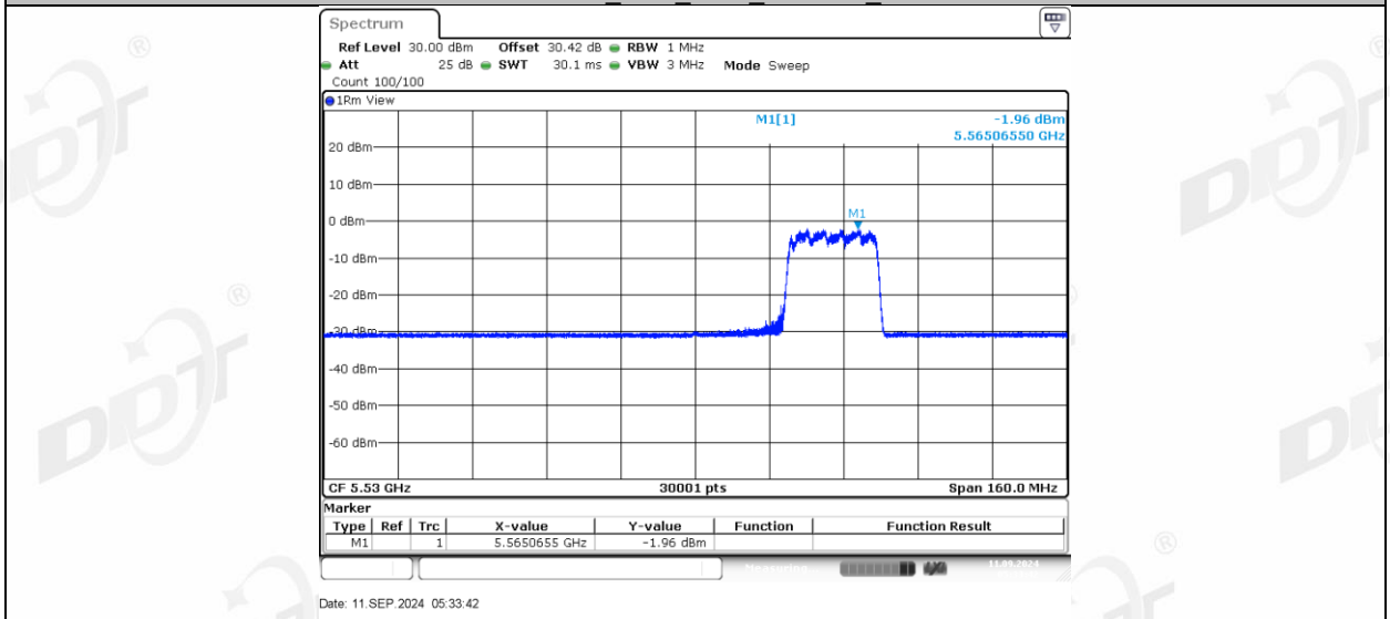
11AX80MIMO_Ant1_5530_484Tone_RU65
