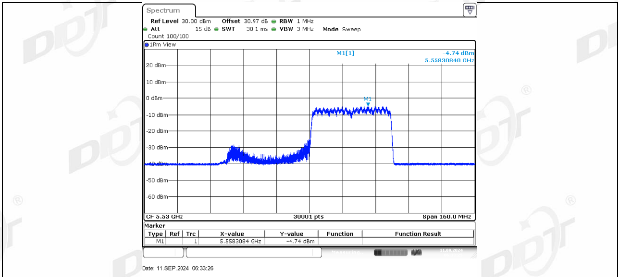
11AX80MIMO_Ant2_5530_242Tone_RU61
