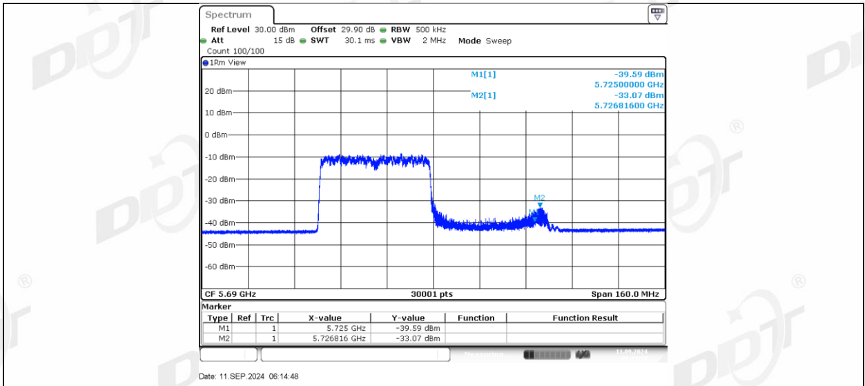
11AX80MIMO_Ant2_5690_UNII-3_484Tone_RU66
