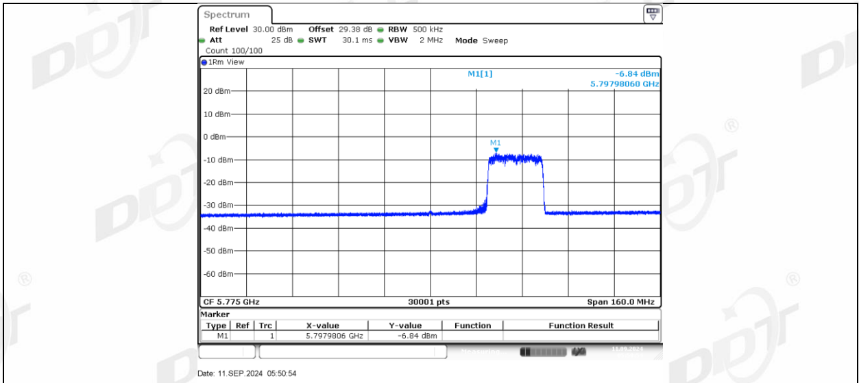
11AX80MIMO_Ant1_5775_484Tone_RU65
