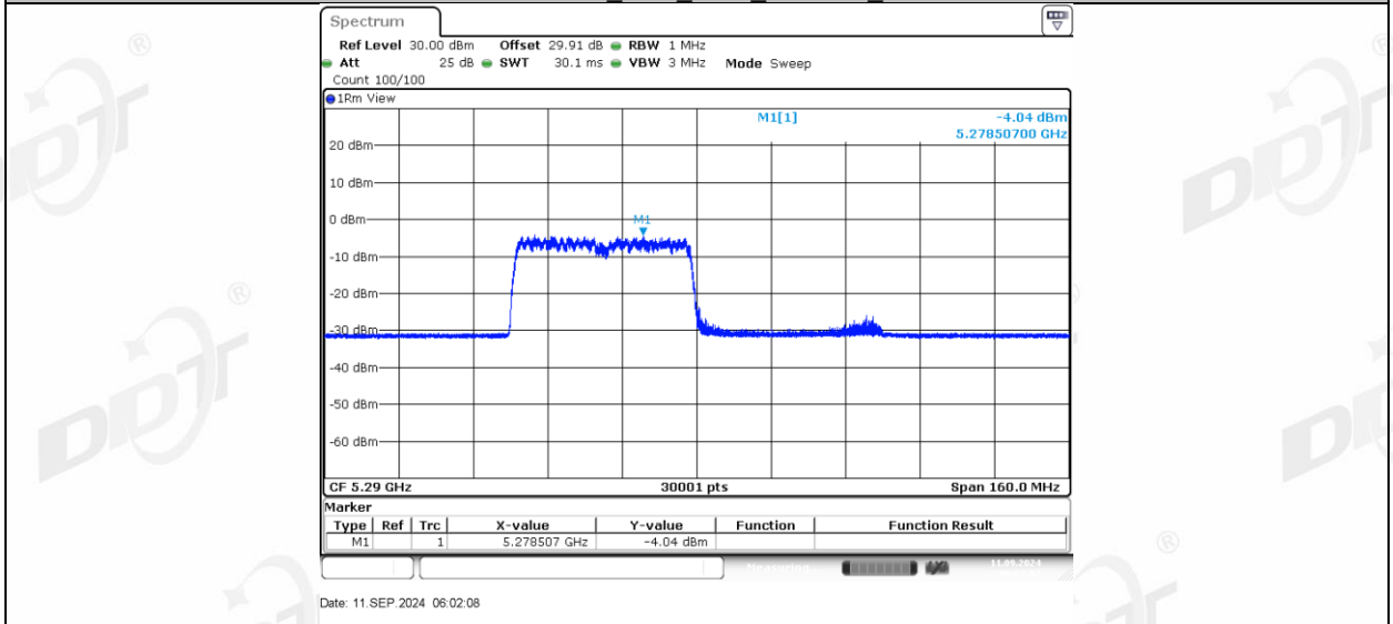
11AX80MIMO_Ant2_5290_484Tone_RU66
