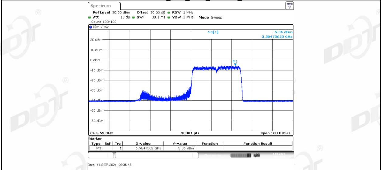
11AX80MIMO_Ant1_5610_242Tone_RU61
