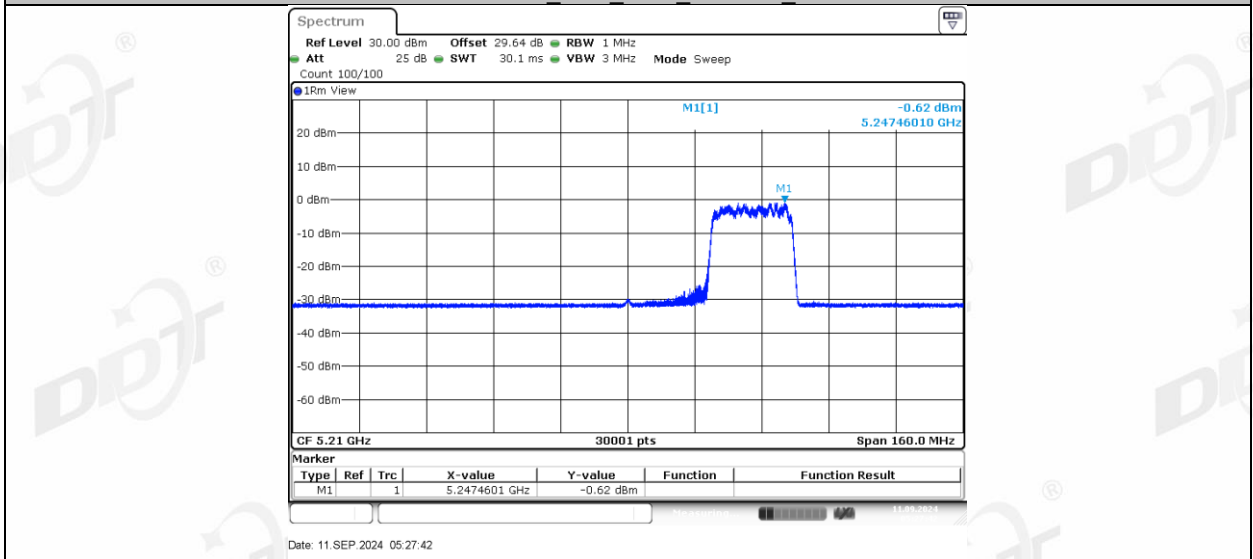
11AX80MIMO_Ant2_5210_484Tone_RU65
