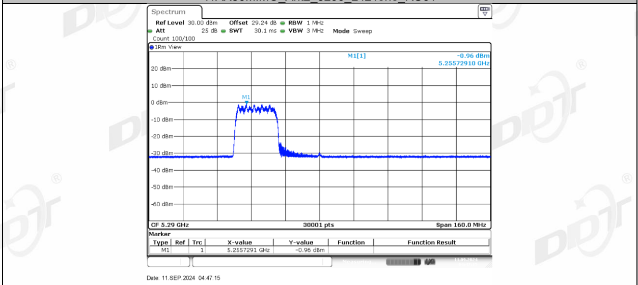
11AX80MIMO_Ant2_5290_242Tone_RU64
