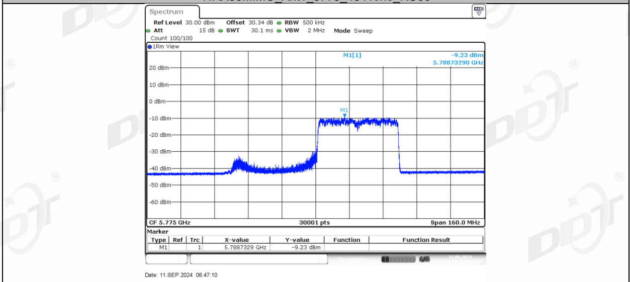
11AX80MIMO_Ant2_5775_242Tone_RU61
