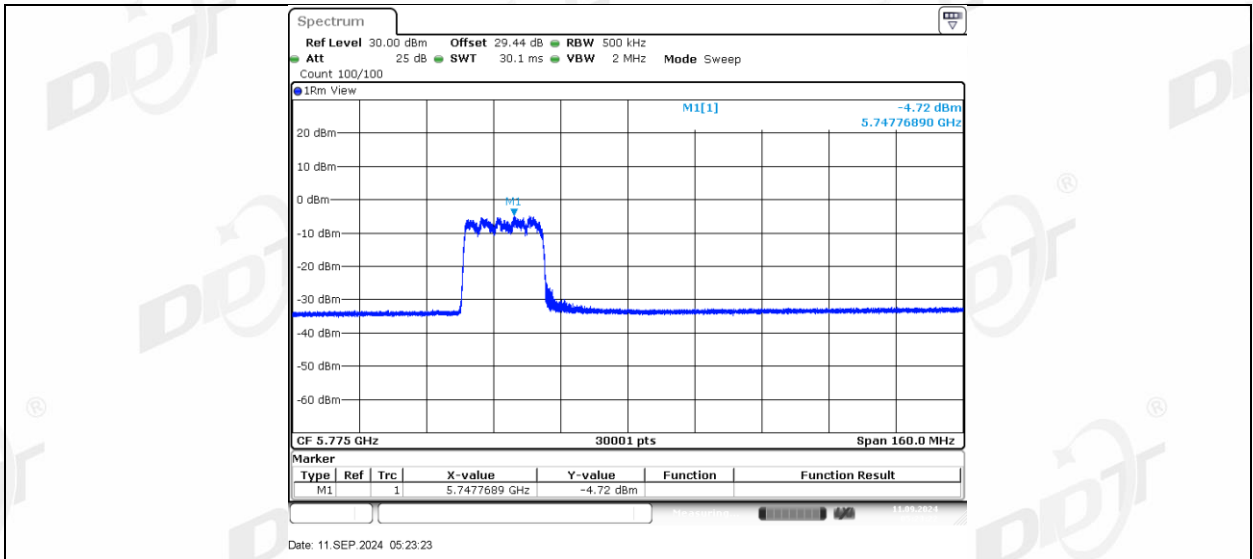
11AX80MIMO_Ant2_5775_242Tone_RU64
