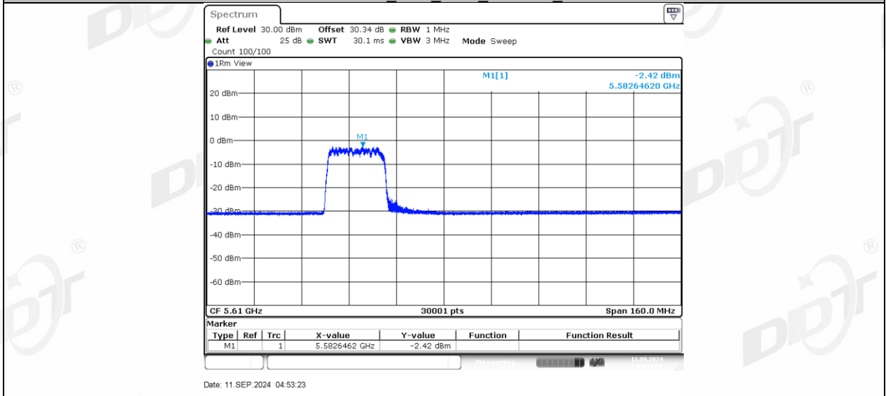
11AX80MIMO_Ant1_5610_242Tone_RU64
