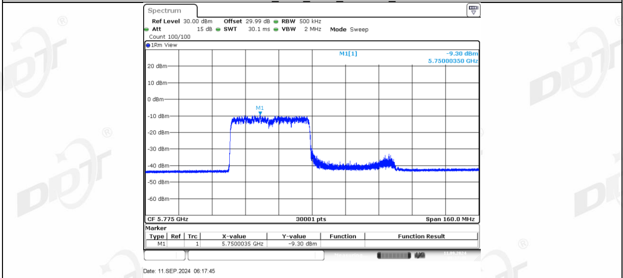
11AX80MIMO_Ant1_5775_484Tone_RU66
