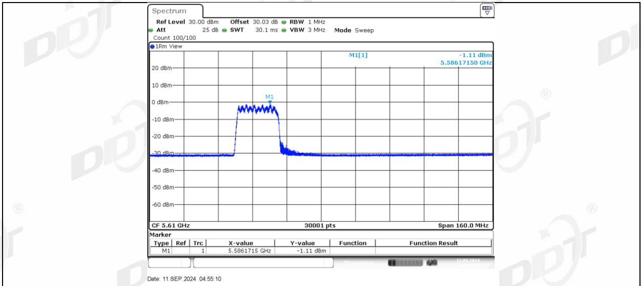
11AX80MIMO_Ant2_5610_242Tone_RU64
