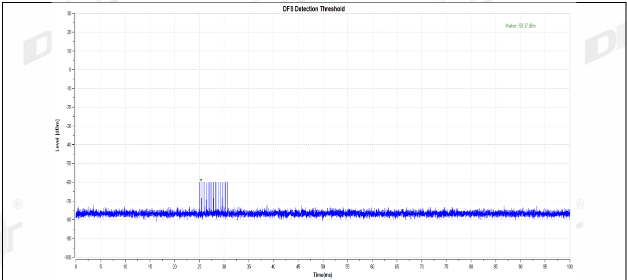
11AC80MIMO_5290_Type4
