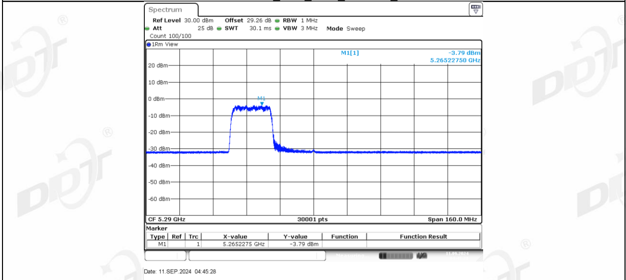
11AX80MIMO_Ant1_5290_242Tone_RU64
