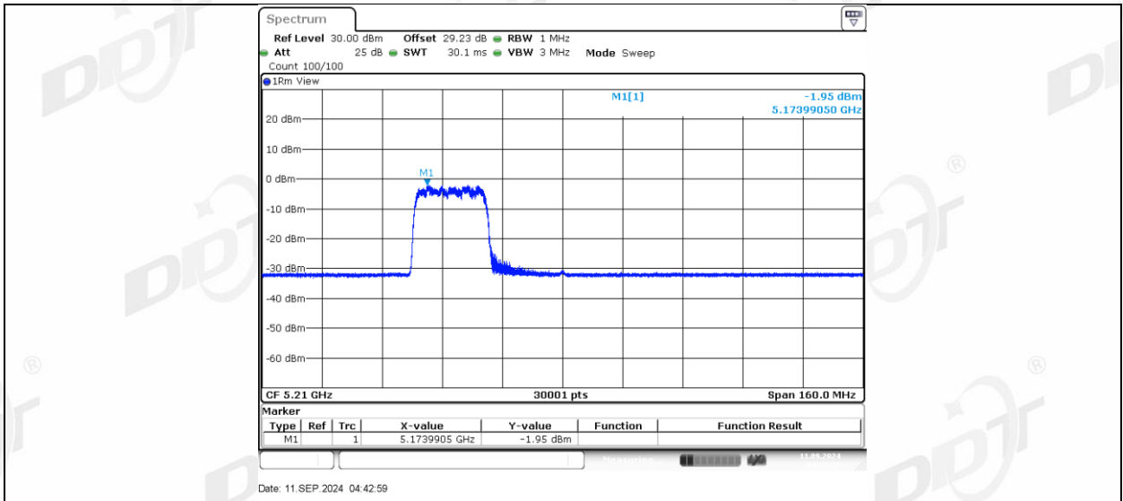
11AX80MIMO_Ant2_5210_242Tone_RU64
