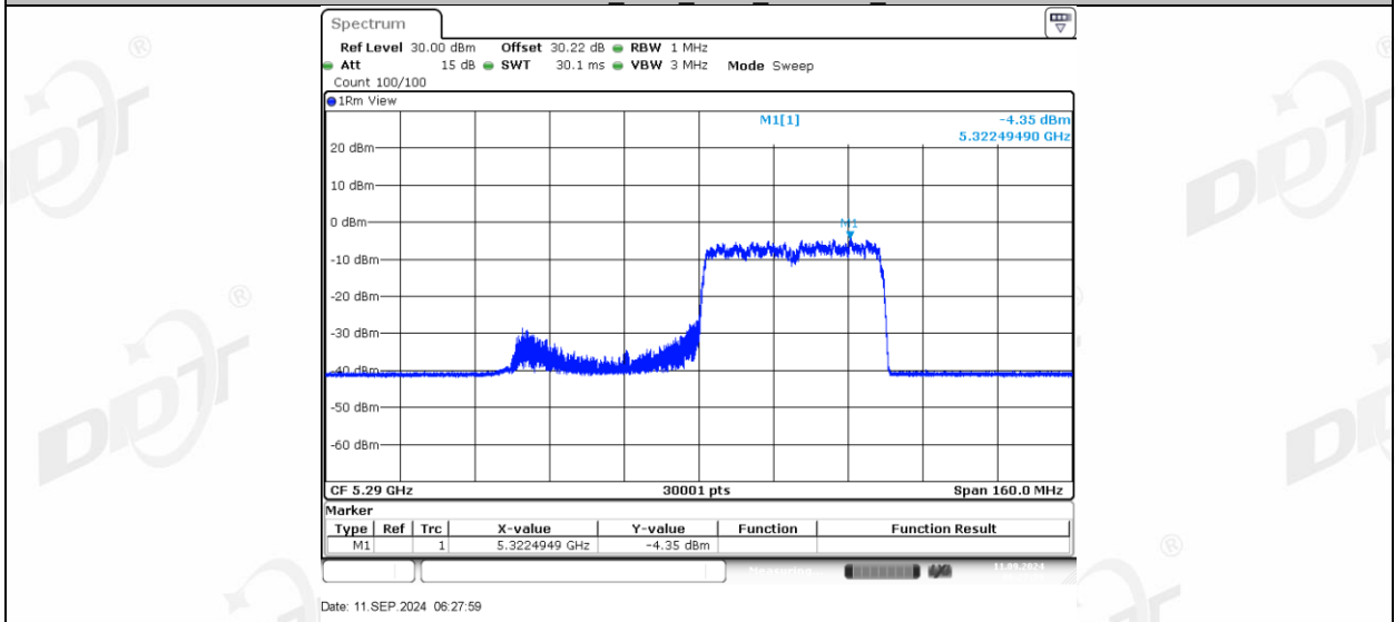
11AX80MIMO_Ant2_5290_242Tone_RU61
