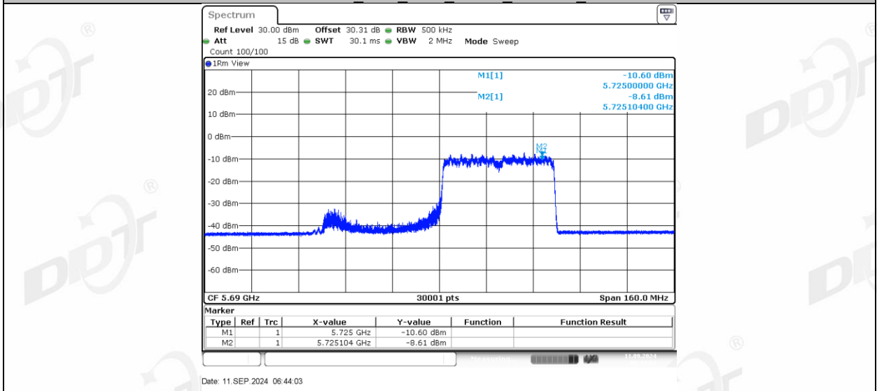
11AX80MIMO_Ant1_5775_242Tone_RU61
