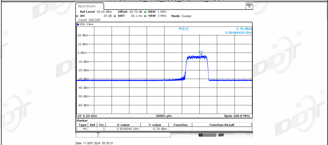
11AX80MIMO_Ant2_5530_484Tone_RU65
