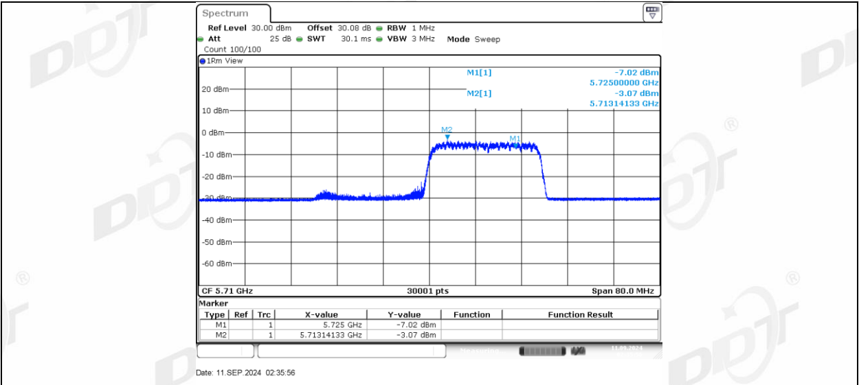
11AX40MIMO_Ant2_5710_UNII-2C_106Tone_RU53
