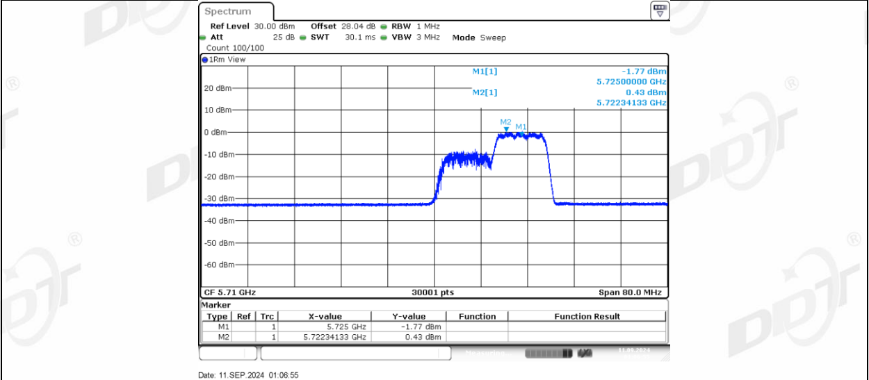
11AX40MIMO_Ant2_5710_UNII-2C_242Tone_RU61
