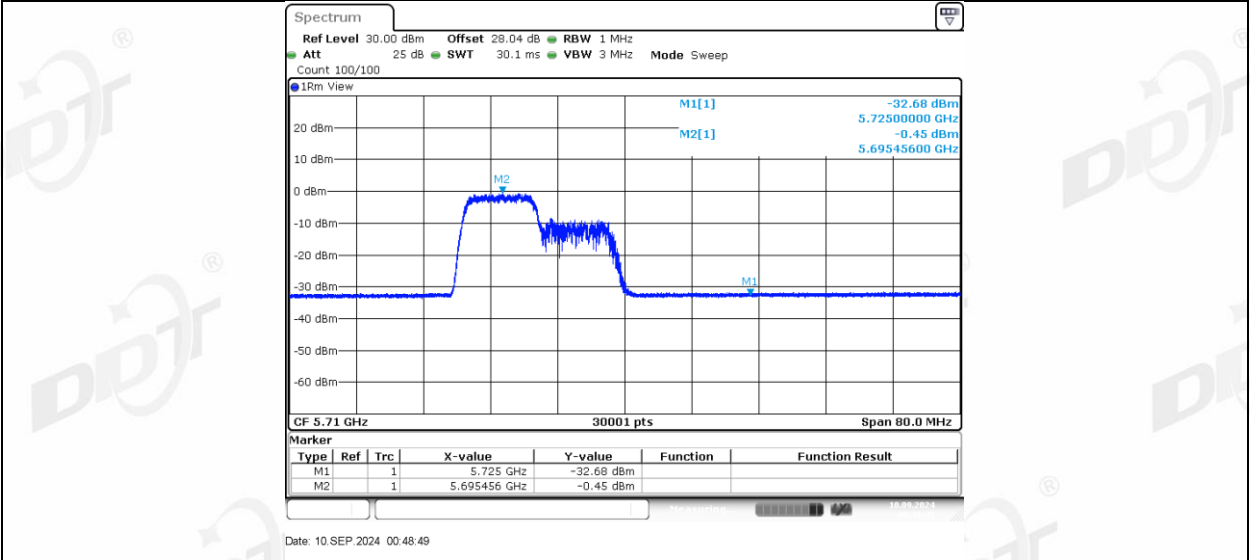
11AX40MIMO_Ant2_5710_UNII-2C_106Tone_RU56
