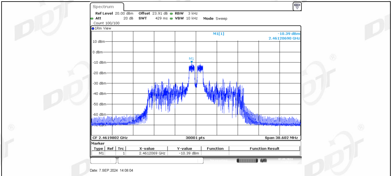
11AX20MIMO_Ant1_2462_26Tone_RU8
