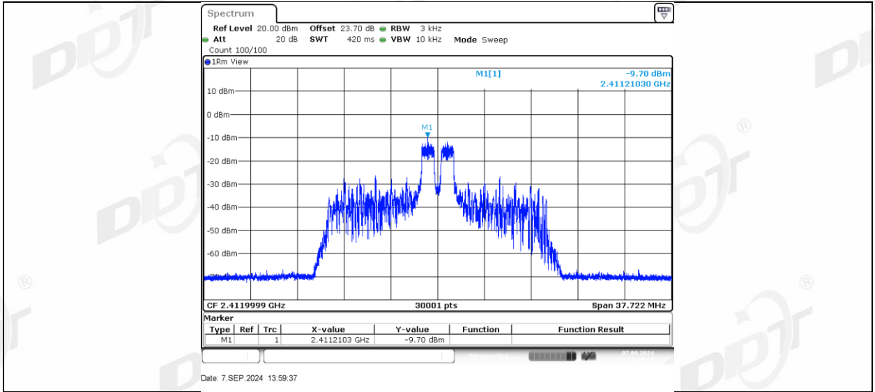
11AX20MIMO_Ant2_2412_26Tone_RU8
