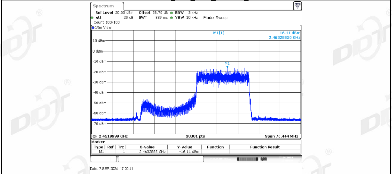
11AX40MIMO_Ant2_2452_106Tone_RU53
