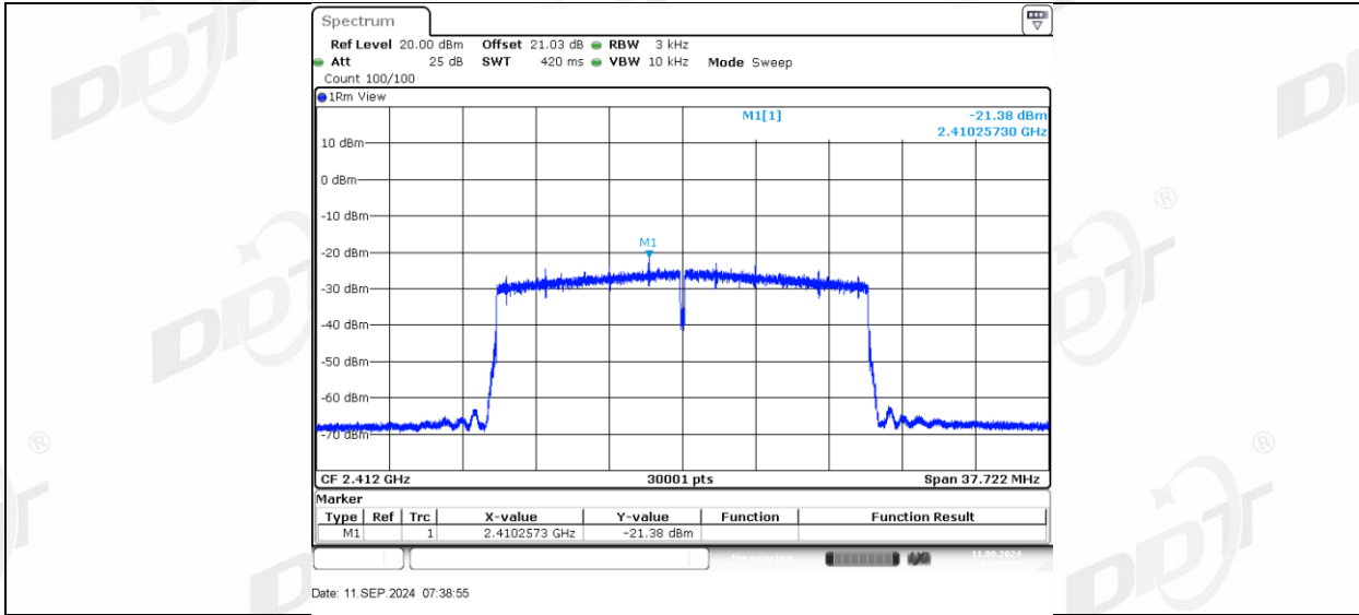
11AX20MIMO_Ant2_2412
