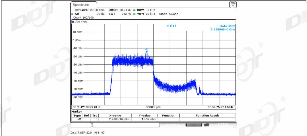
11AX40MIMO_Ant2_2422_242Tone_RU62
