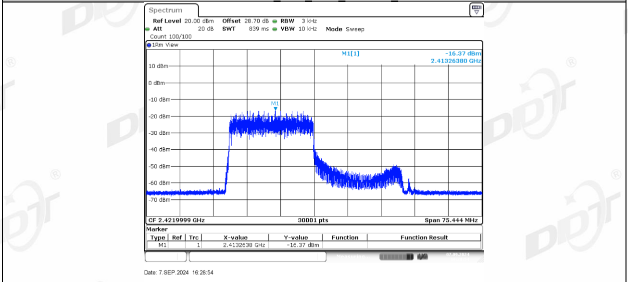
11AX40MIMO_Ant1_2422_242Tone_RU62
