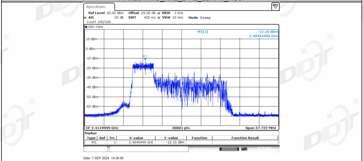
11AX20MIMO_Ant2_2412_52Tone_RU39
