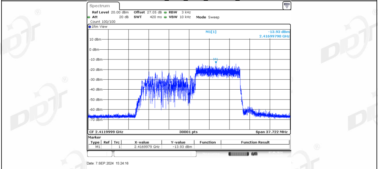
11AX20MIMO_Ant2_2412_26Tone_RU0
