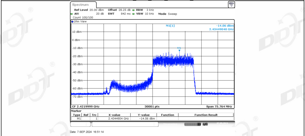
11AX40MIMO_Ant1_2437_106Tone_RU53
