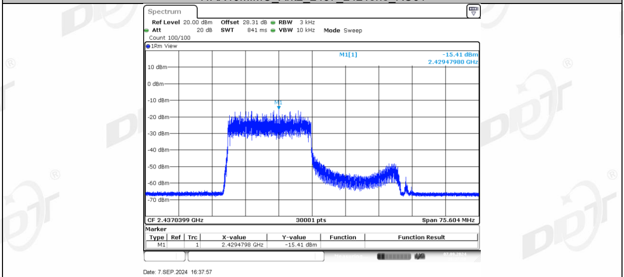
11AX40MIMO_Ant2_2437_242Tone_RU62
