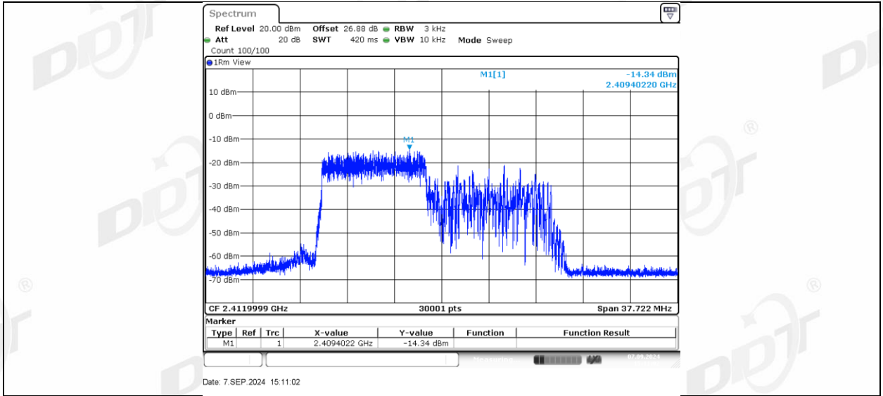
11AX20MIMO_Ant1_2412_106Tone_RU54
