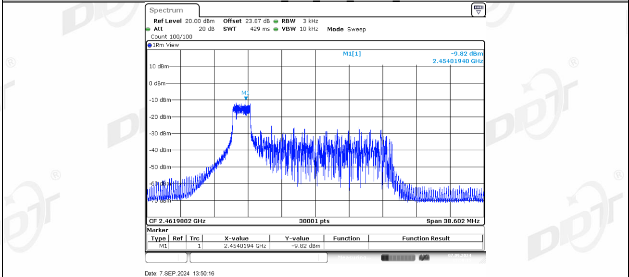
11AX20MIMO_Ant1_2462_26Tone_RU4
