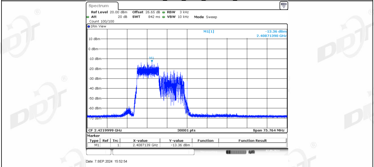
11AX40MIMO_Ant2_2422_106Tone_RU56
