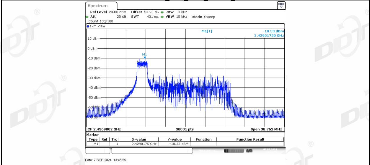
11AX20MIMO_Ant1_2437_26Tone_RU4
