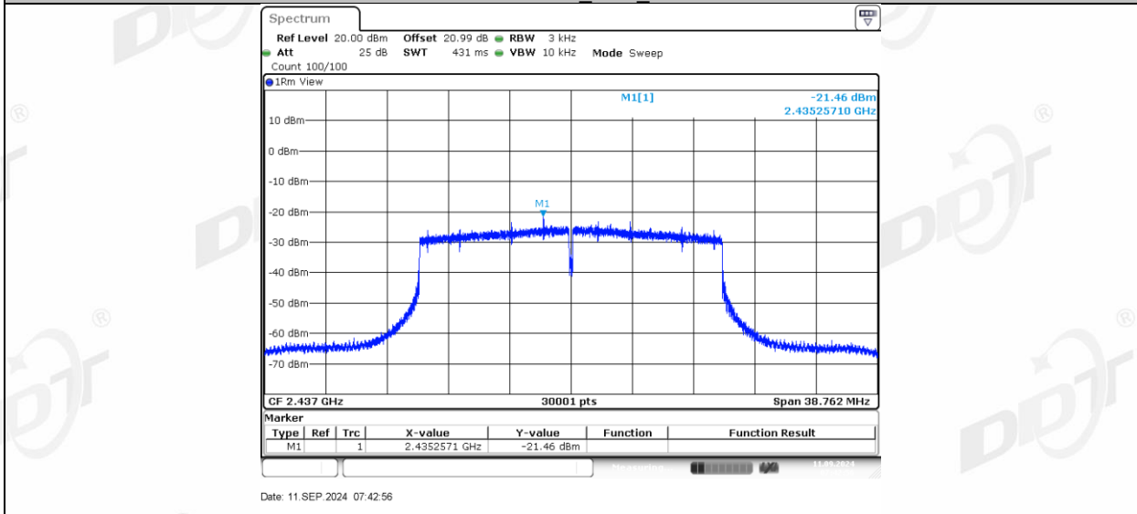
11AX20MIMO_Ant2_2437
