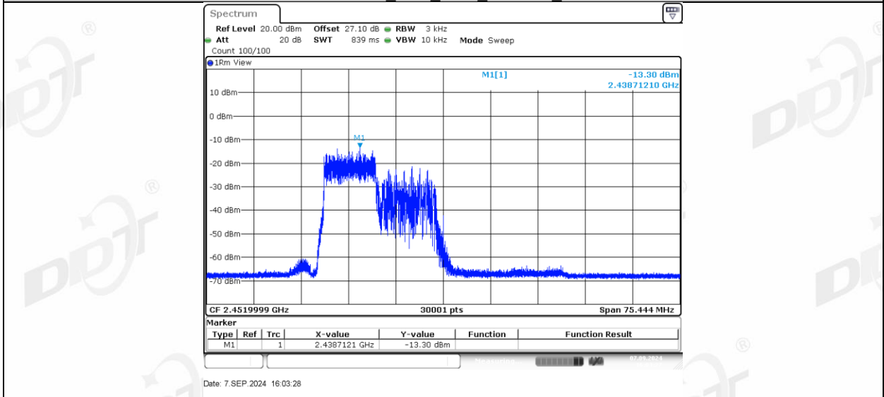
11AX40MIMO_Ant1_2452_106Tone_RU56
