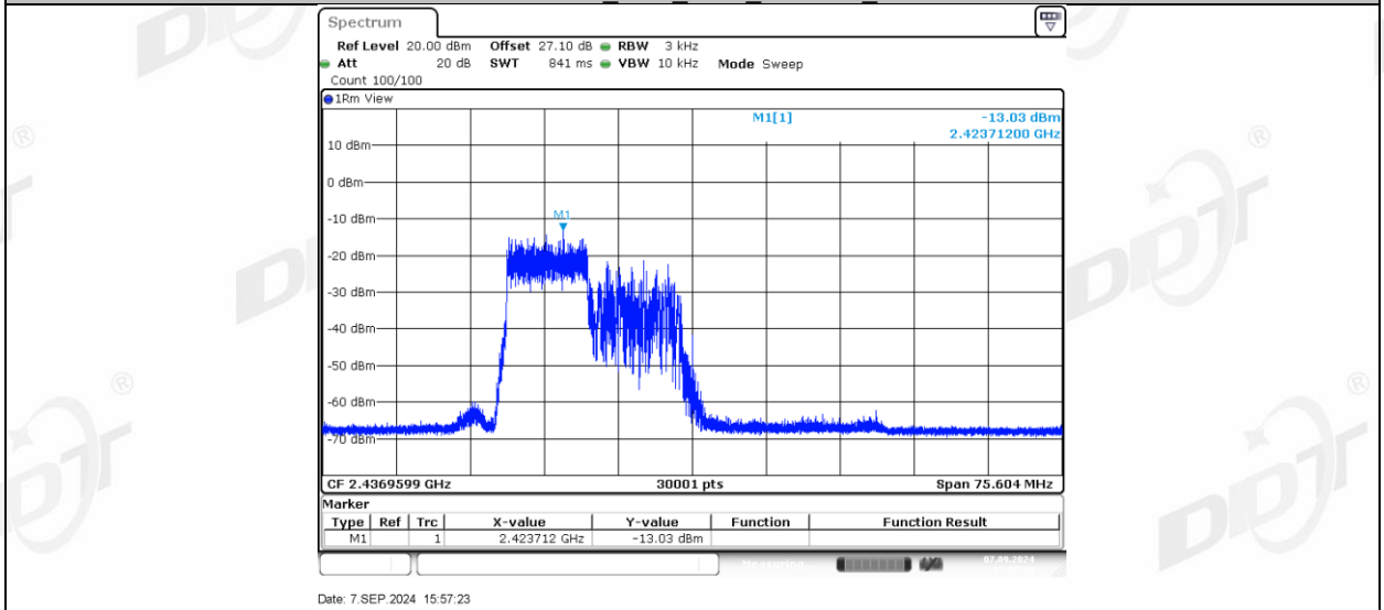
11AX40MIMO_Ant1_2437_106Tone_RU56
