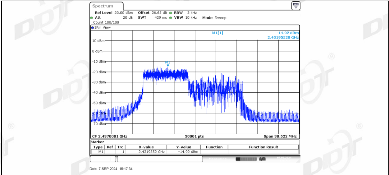
11AX20MIMO_Ant2_2437_106Tone_RU54
