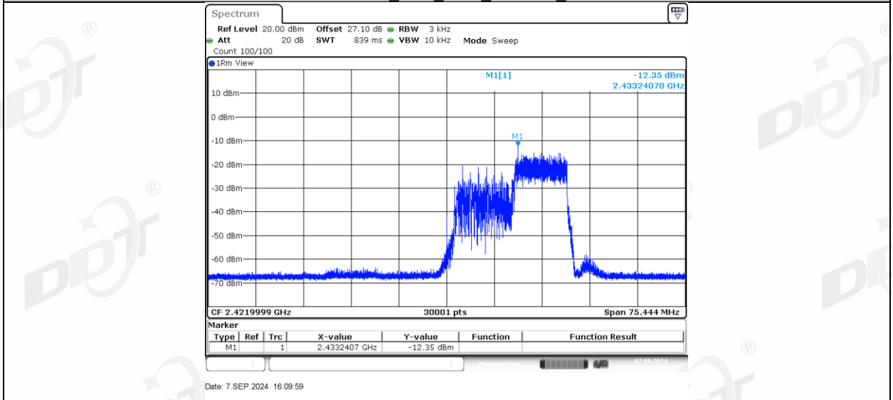
11AX40MIMO_Ant1_2422_242Tone_RU61
