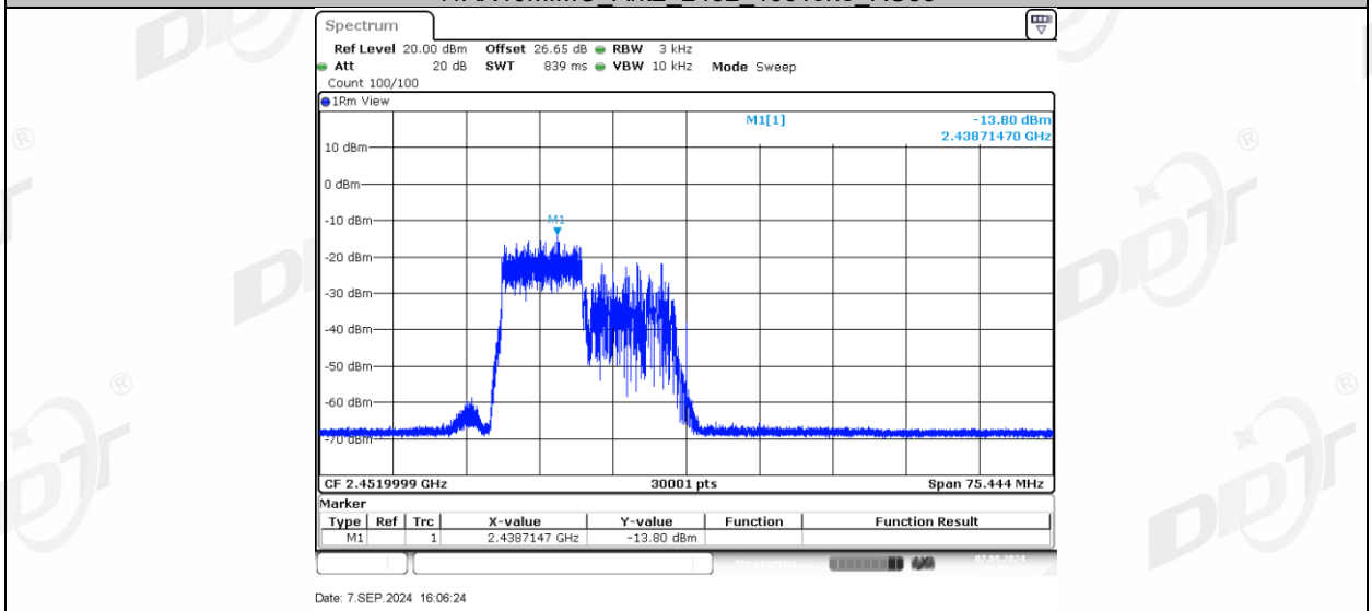
11AX40MIMO_Ant2_2452_106Tone_RU56
