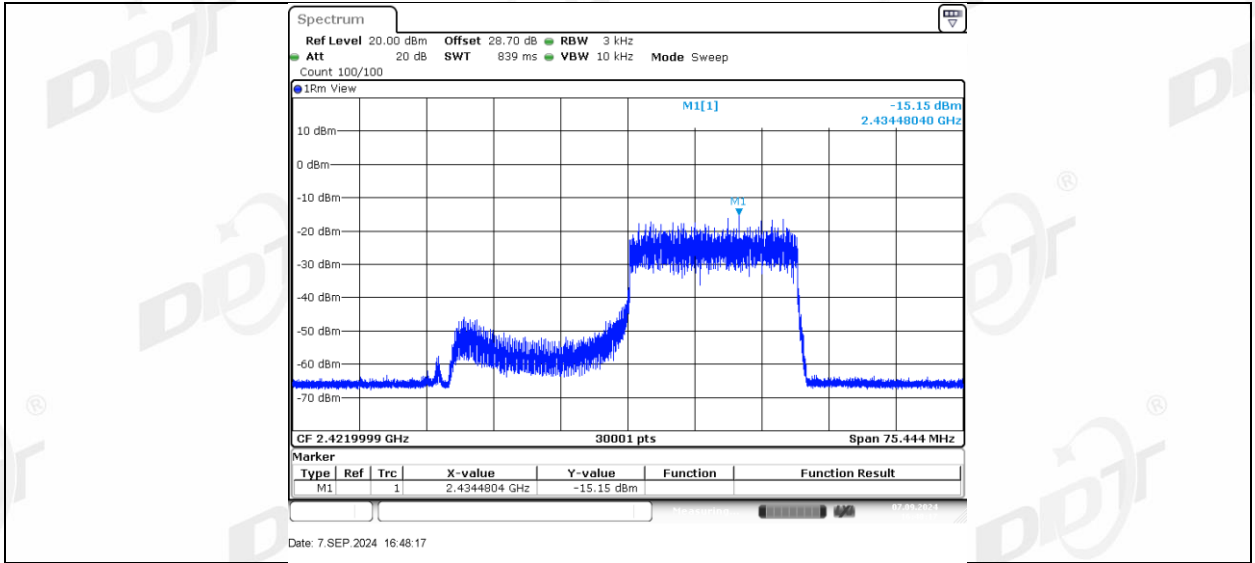
11AX40MIMO_Ant2_2422_106Tone_RU53
