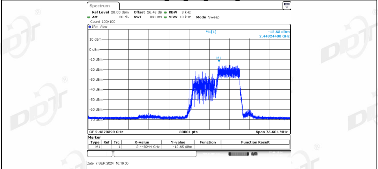
11AX40MIMO_Ant2_2437_242Tone_RU61
