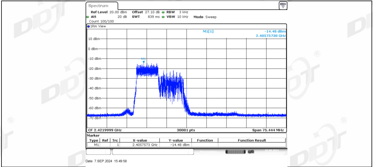
11AX40MIMO_Ant1_2422_106Tone_RU56
