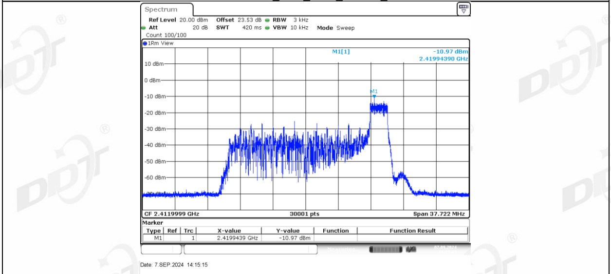
11AX20MIMO_Ant2_2412_52Tone_RU37
