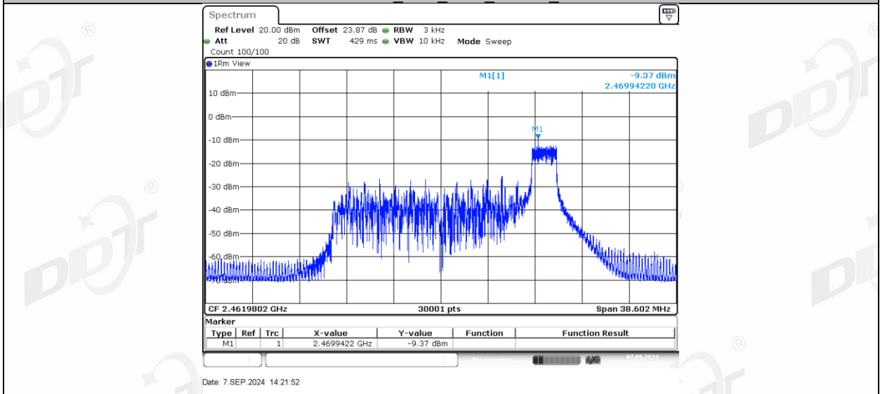
11AX20MIMO_Ant1_2462_52Tone_RU37
