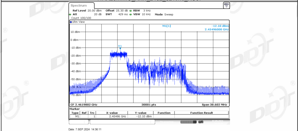
11AX20MIMO_Ant1_2462_52Tone_RU39
