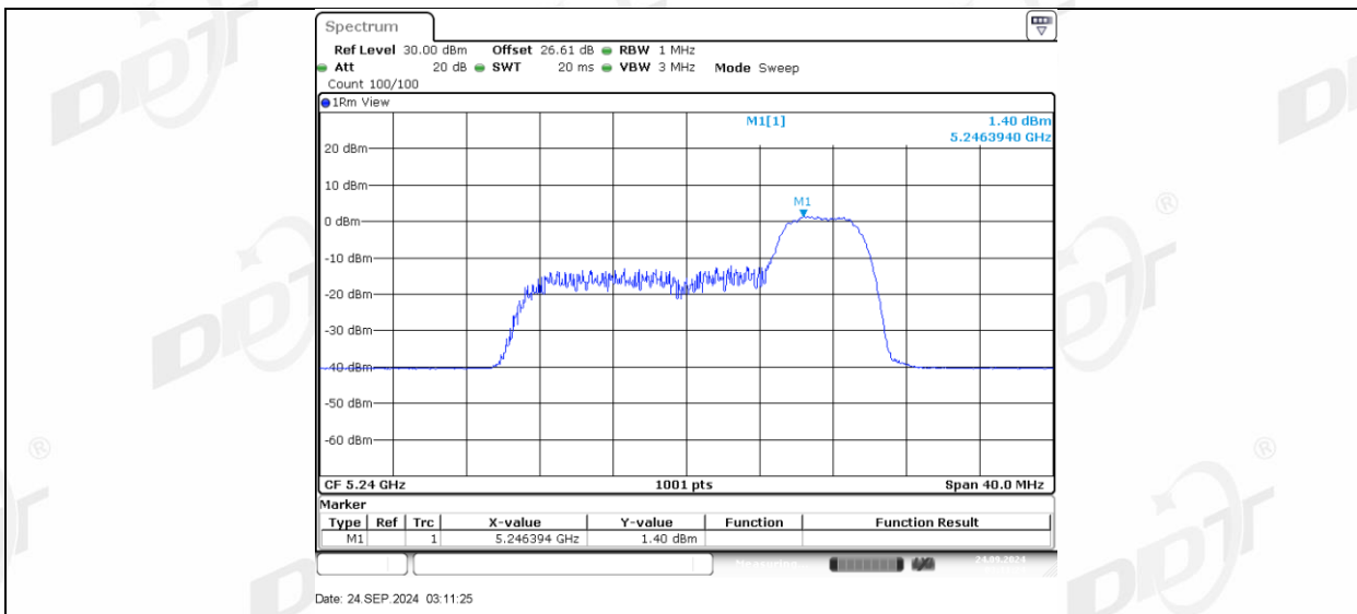
11AX20MIMO_Ant1_5240_106Tone_RU53
