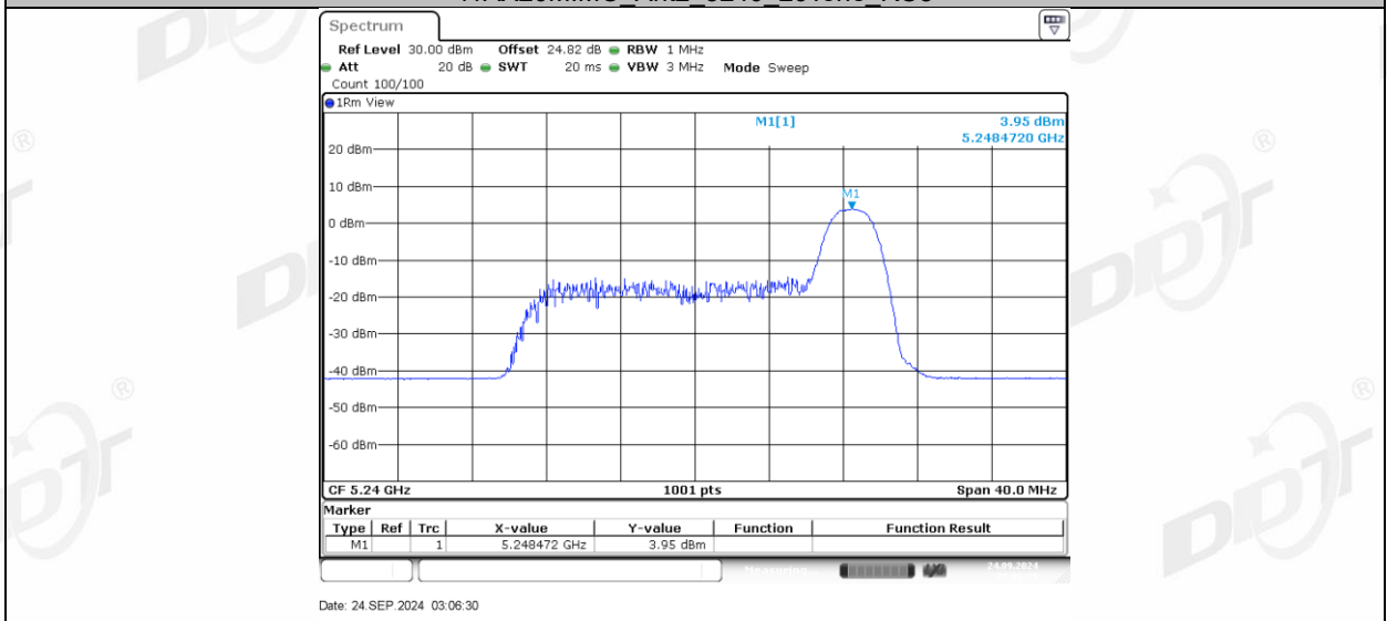
11AX20MIMO_Ant2_5240_52Tone_RU37
