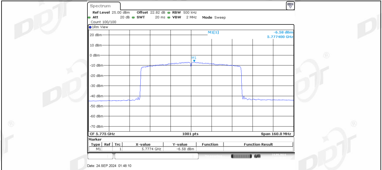
11AX80MIMO_Ant2_5775
