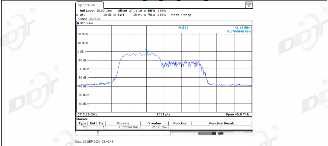
11AX20MIMO_Ant2_5180_106Tone_RU54
