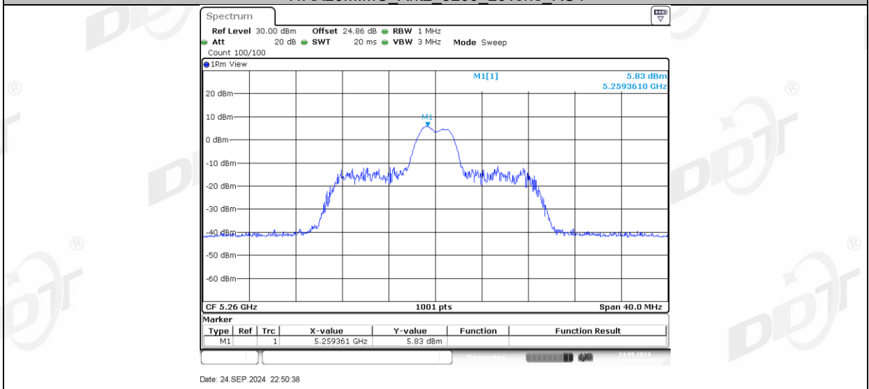
11AX20MIMO_Ant2_5260_26Tone_RU8
