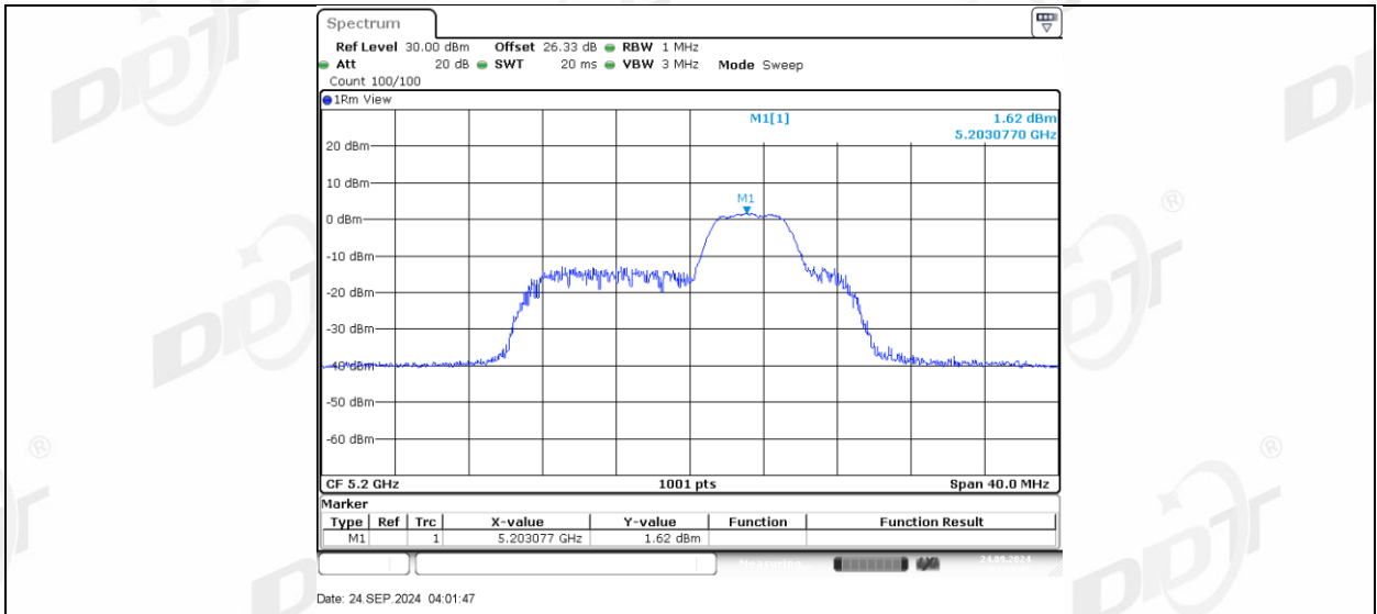
11AX20MIMO_Ant2_5200_52Tone_RU40
