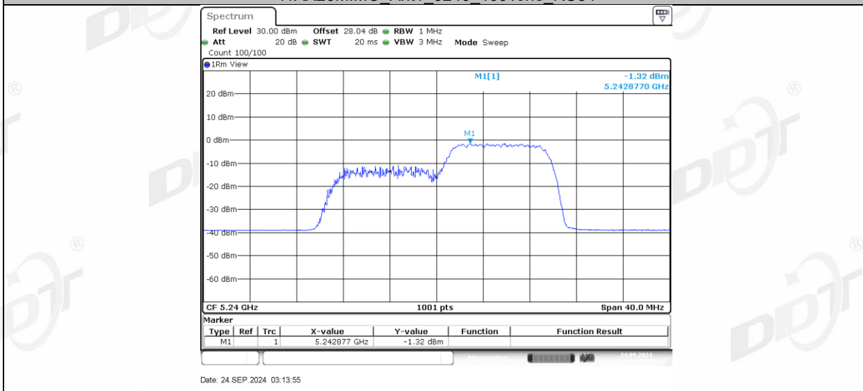
11AX20MIMO_Ant2_5240_26Tone_RU0
