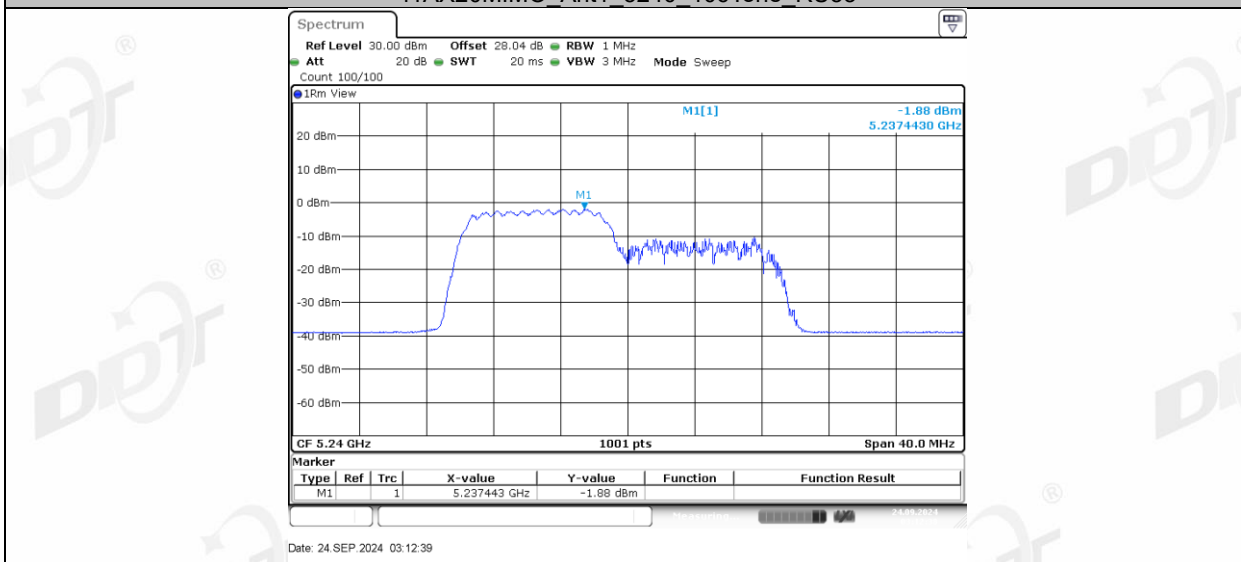
11AX20MIMO_Ant1_5240_106Tone_RU54
