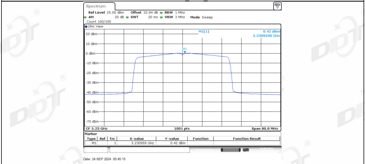
11AX40MIMO_Ant2_5230
