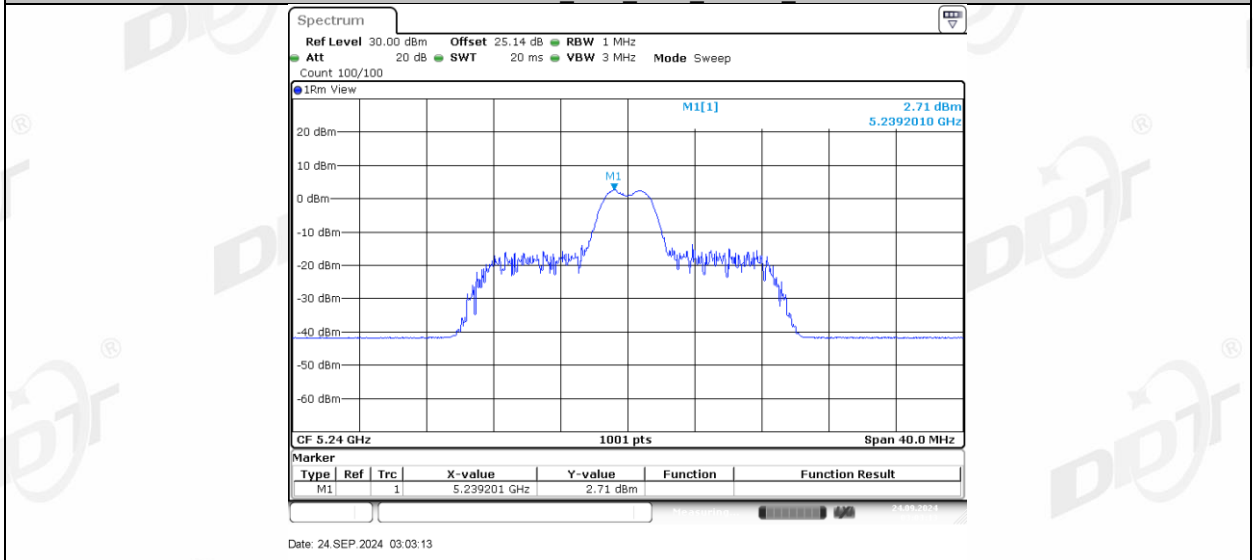
11AX20MIMO_Ant1_5240_26Tone_RU8
