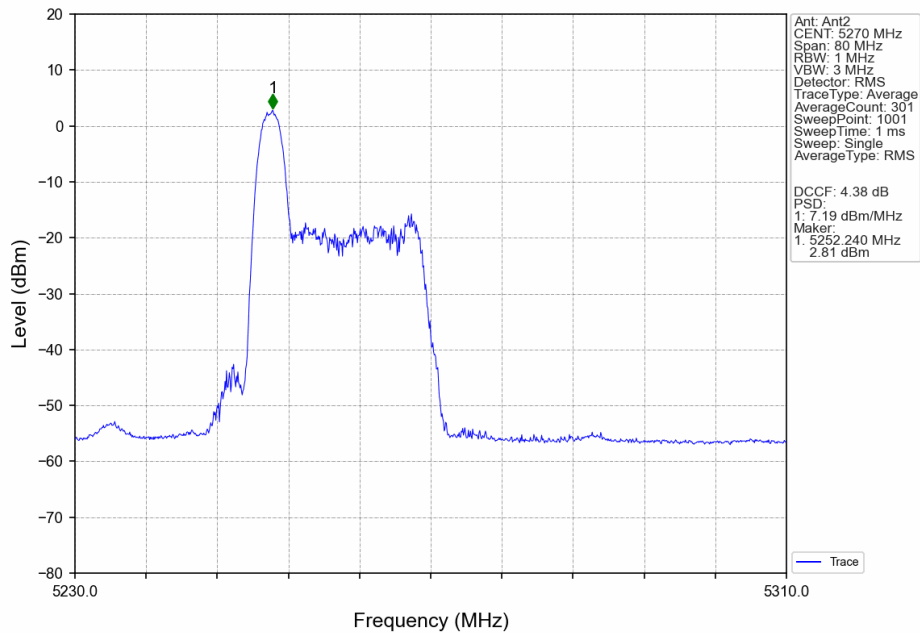
802.11ax(HEW40)_LCH_5270MHz_RU26_Left_Ant2_NTNV
