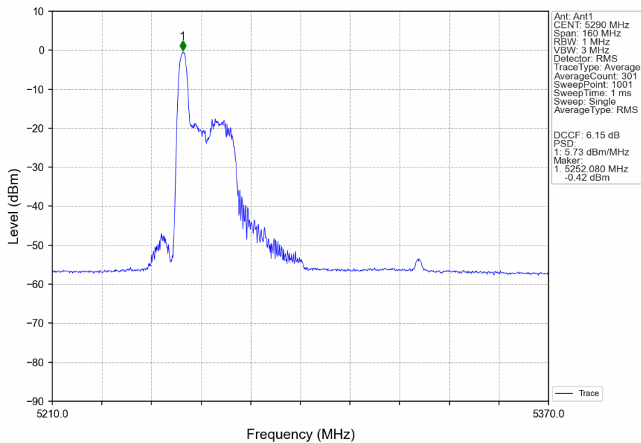
802.11ax(HEW80)_MCH_5290MHz_RU26_Left_Ant1_NTNV
