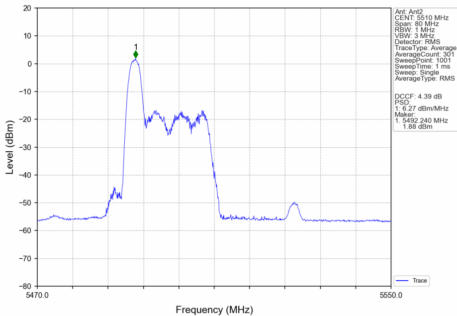
802.11ax(HEW40)_LCH_5510MHz_RU26_Left_Ant2_NTNV
