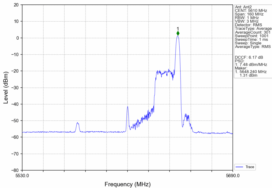
802.11ax(HEW80)_HCH_5610MHz_RU26_Right_Ant2_NTNV
