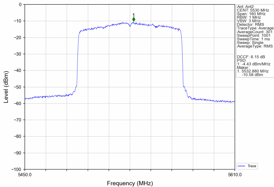
802.11ax(HEW80)_LCH_5530MHz_RU996_Left_MIMO_NTNV
