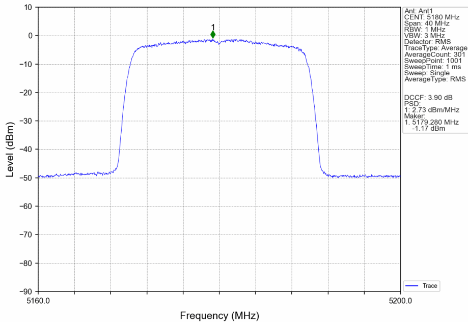
802.11ax(HEW20)_LCH_5180MHz_RU242_Left_Ant1_NTNV
