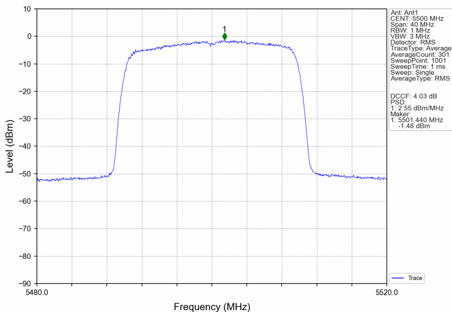
802.11ax(HEW20)_LCH_5500MHz_RU242_Left_Ant1_NTNV
