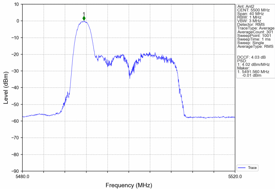
802.11ax(HEW20)_LCH_5500MHz_RU26_Left_Ant2_NTNV
