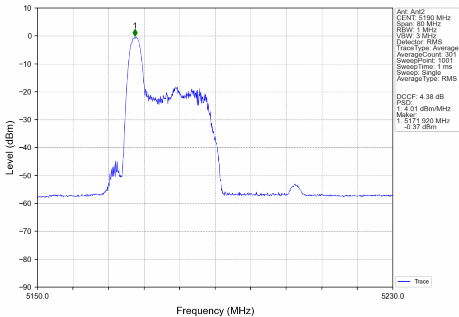
802.11ax(HEW40)_LCH_5190MHz_RU26_Left_Ant2_NTNV
