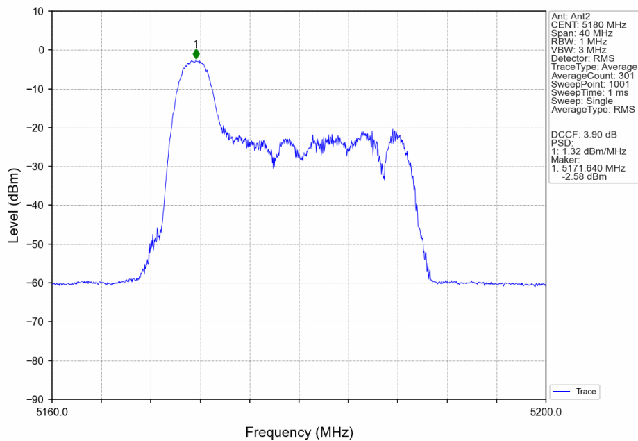
802.11ax(HEW20)_LCH_5180MHz_RU26_Left_Ant2_NTNV
