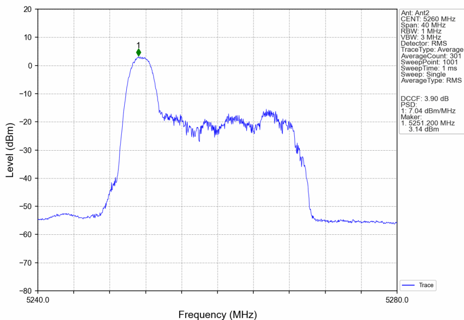
802.11ax(HEW20)_LCH_5260MHz_RU26_Left_Ant2_NTNV
