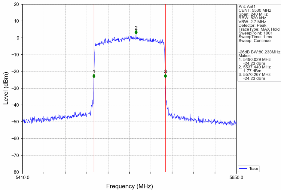
802.11ax(HEW80)_LCH_5530MHz_RU996_Left_Ant1_NTNV
