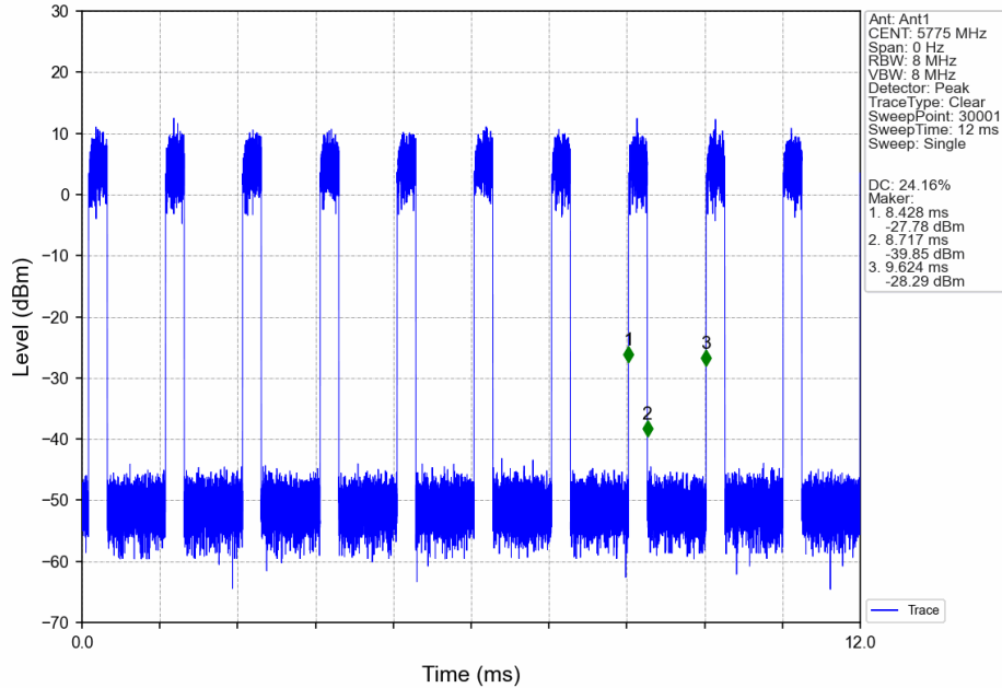
802.11ax(HEW80)_MCH_5775MHz_RU996_Left_Ant1_NTNV
