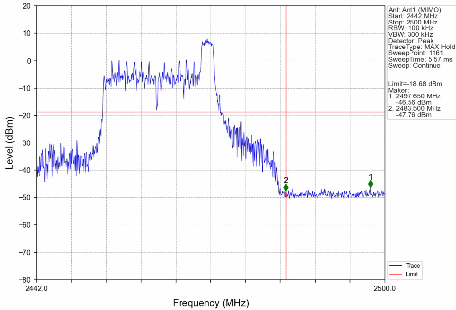
802.11ax(HEW20)_HCH_2462MHz_RU26_Right_Ant1 (MIMO)_NTNV
