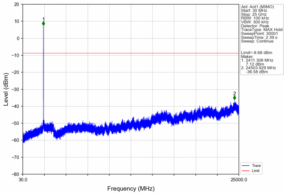
802.11ax(HEW20)_LCH_2412MHz_RU26_Mid_Ant1 (MIMO)_NTNV
