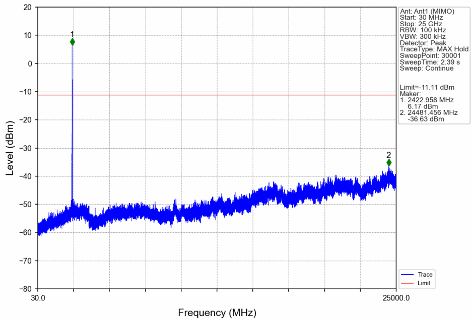
802.11ax(HEW40)_LCH_2422MHz_RU26_Mid_Ant1 (MIMO)_NTNV
