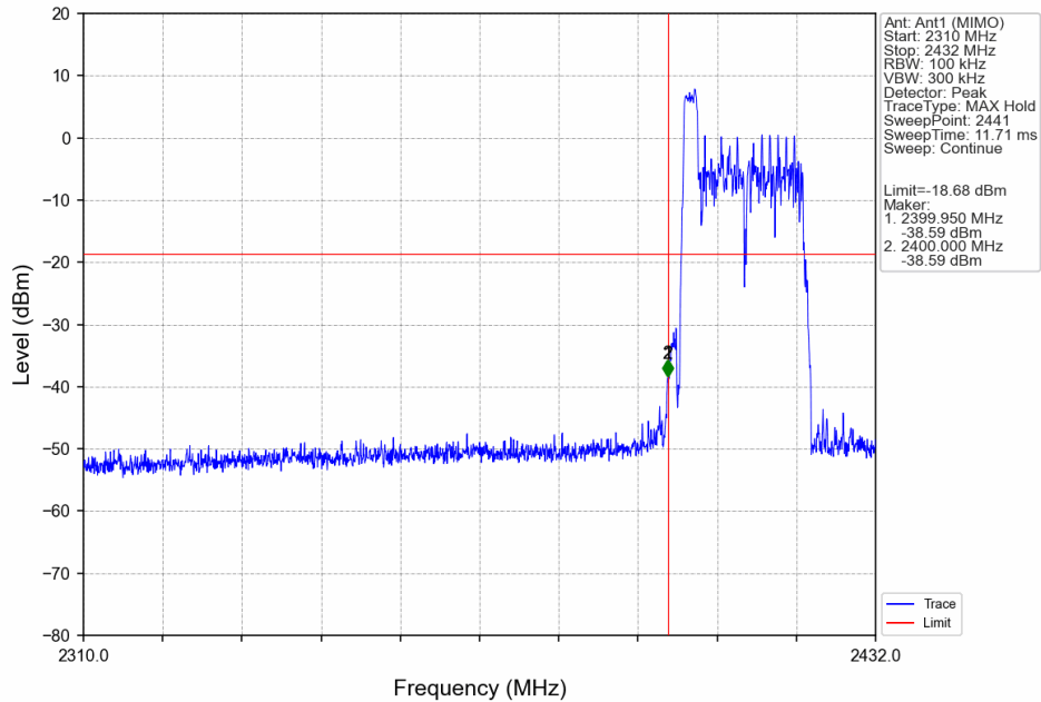
802.11ax(HEW20)_LCH_2412MHz_RU26_Left_Ant1 (MIMO)_NTNV
