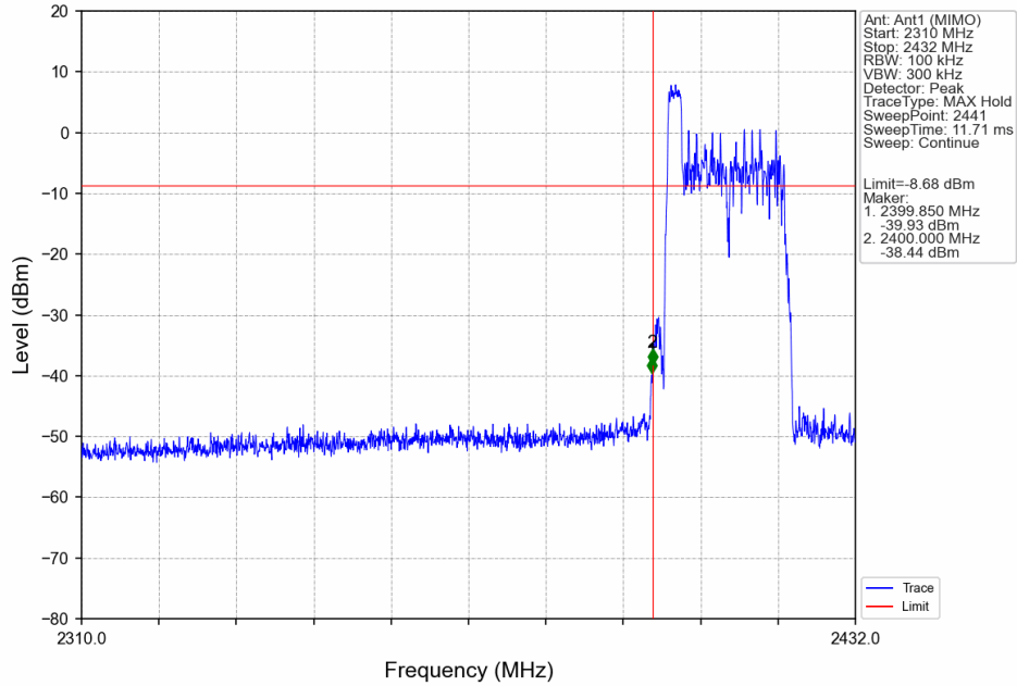
802.11ax(HEW20)_LCH_2412MHz_RU26_Mid_Ant1 (MIMO)_NTNV
