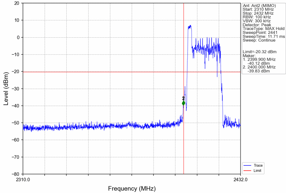
802.11ax(HEW20)_LCH_2412MHz_RU26_Left_Ant2 (MIMO)_NTNV
