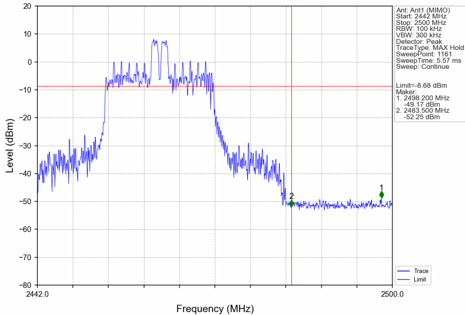
802.11ax(HEW20)_HCH_2462MHz_RU26_Mid_Ant1 (MIMO)_NTNV
