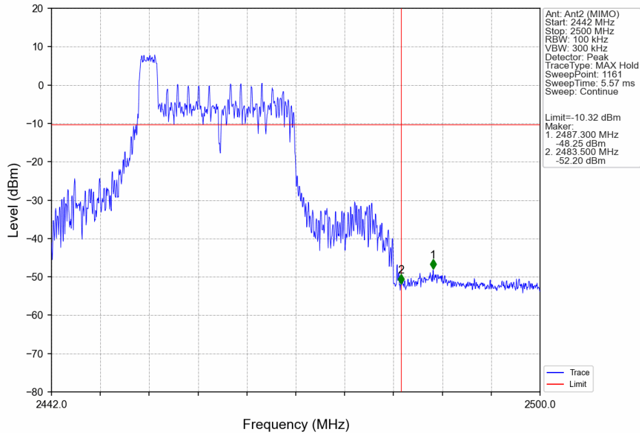
802.11ax(HEW20)_HCH_2462MHz_RU26_Left_Ant2 (MIMO)_NTNV
