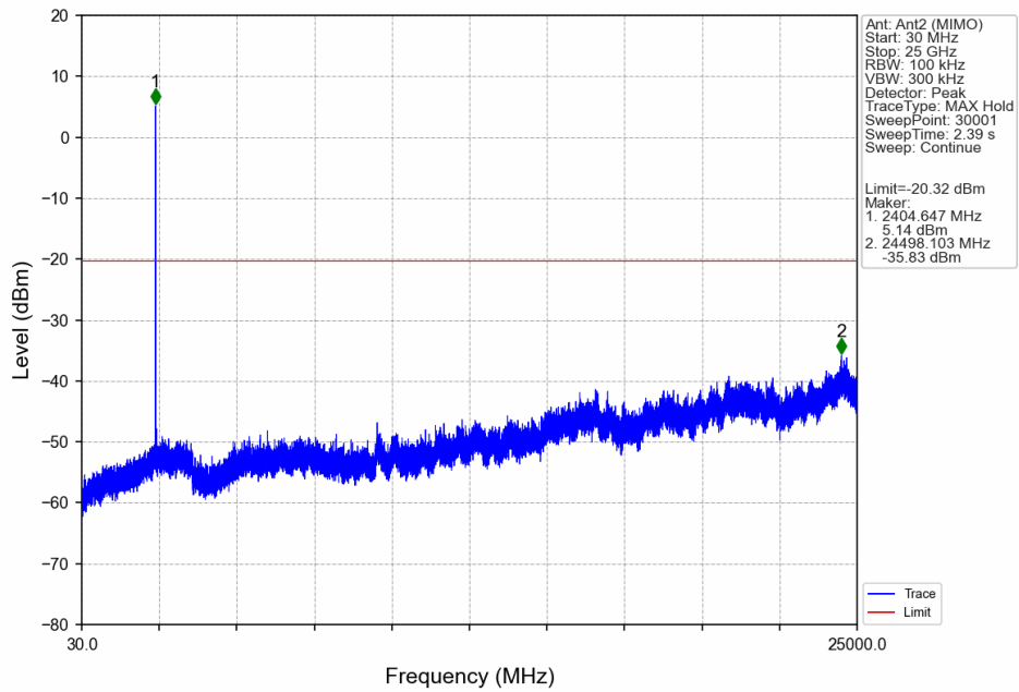
802.11ax(HEW20)_LCH_2412MHz_RU26_Left_Ant2 (MIMO)_NTNV
