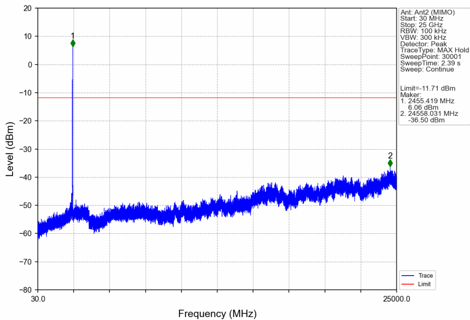
802.11ax(HEW40)_MCH_2437MHz_RU26_Right_Ant2 (MIMO)_NTNV
