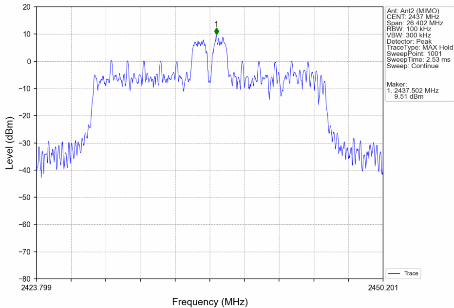
802.11ax(HEW20)_MCH_2437MHz_RU26_Mid_Ant2 (MIMO)_NTNV
