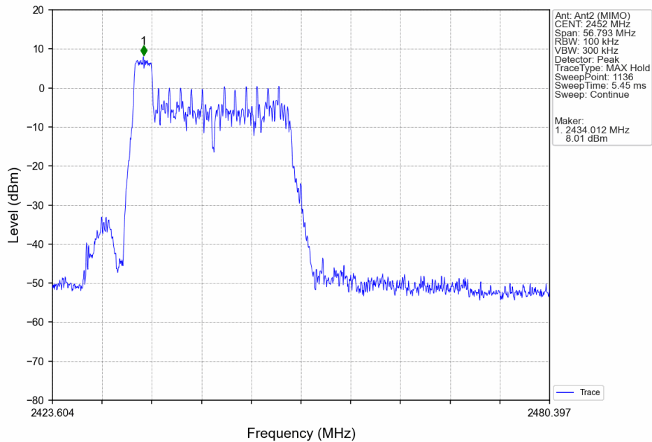
802.11ax(HEW40)_HCH_2452MHz_RU26_Left_Ant2 (MIMO)_NTNV
