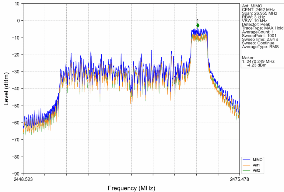
802.11ax(HEW20)_HCH_2462MHz_RU242_Left_Ant1 (MIMO)_NTNV
