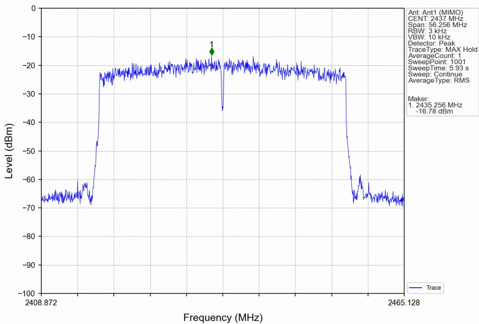
802.11ax(HEW40)_MCH_2437MHz_RU484_Left_Ant1 (MIMO)_NTNV
