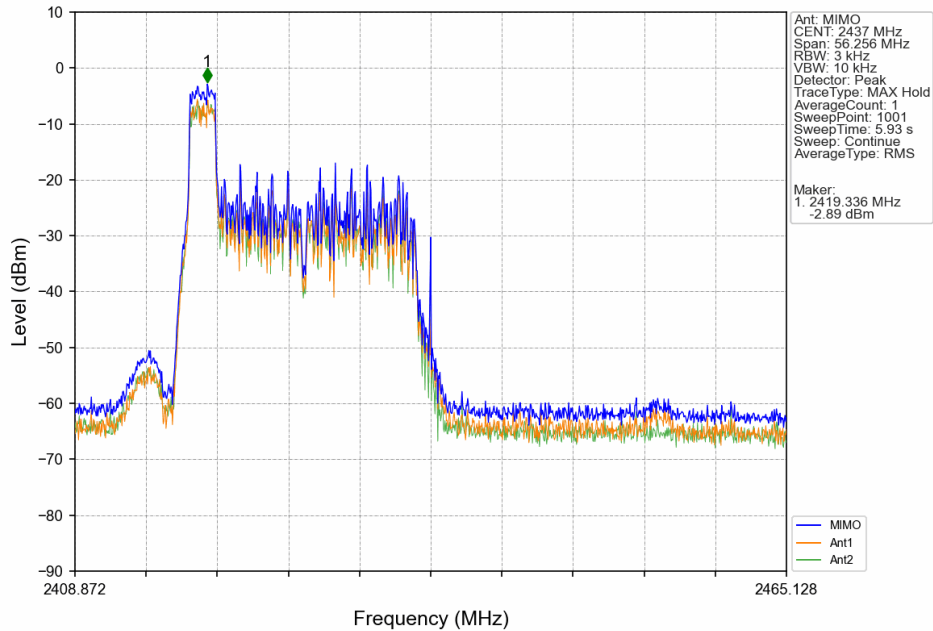
802.11ax(HEW40)_MCH_2437MHz_RU484_Left_Ant1 (MIMO)_NTNV
