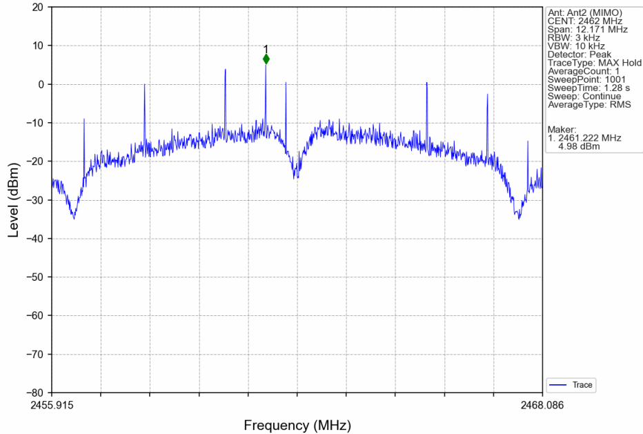
802.11g_HCH_2462MHz_MIMO_NTNV
