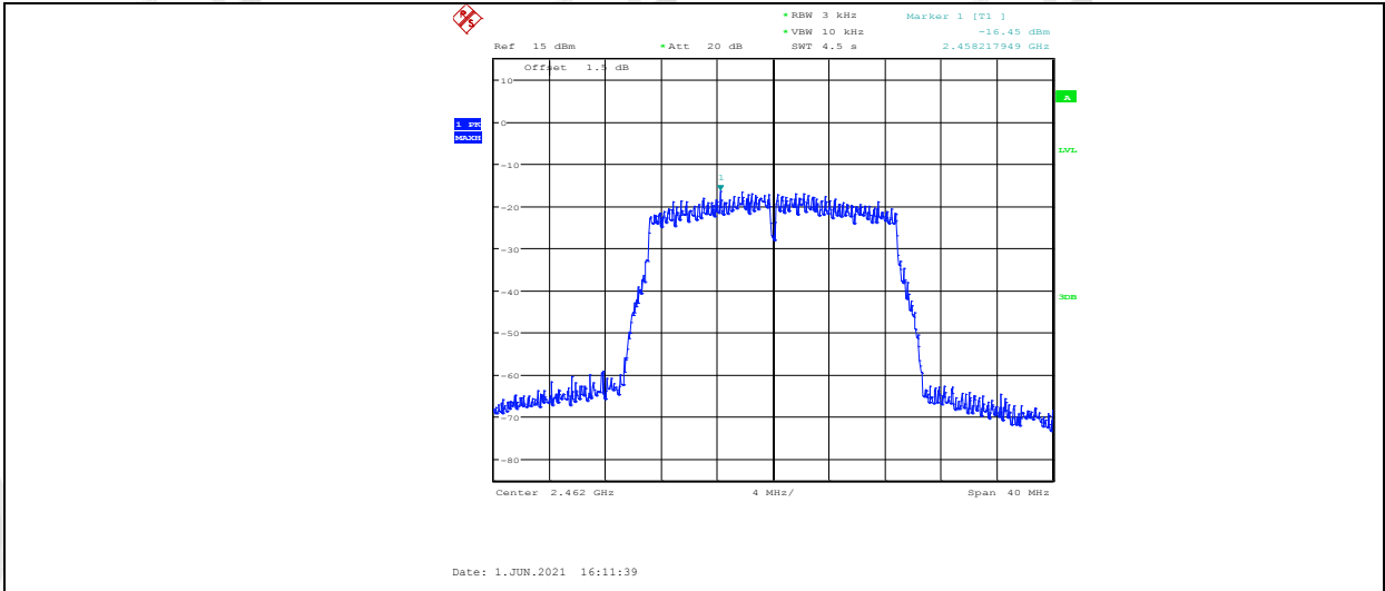
11N20MIMO_ANT2_2462
