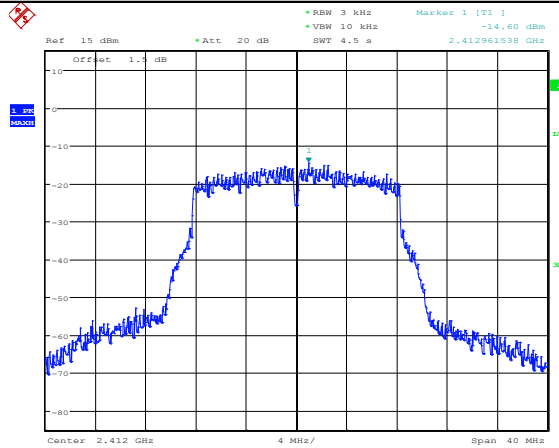
11G_ANT1_2412
