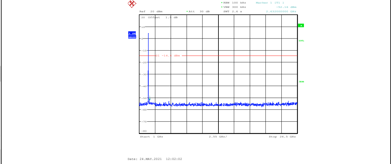
11N40MIMO_ANT1_2422_Ref
