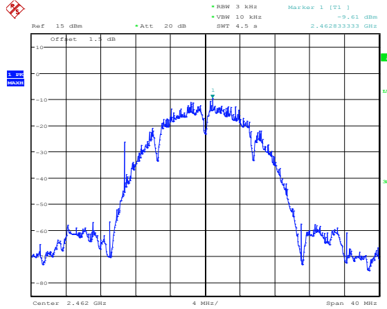
11B_ANT2_2462
