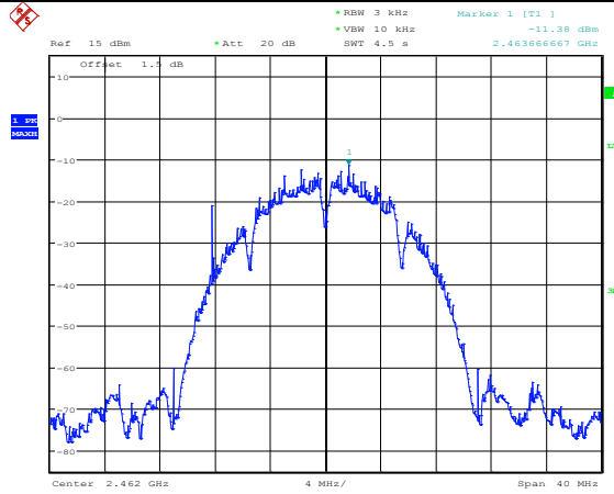
11B_ANT2_2462
