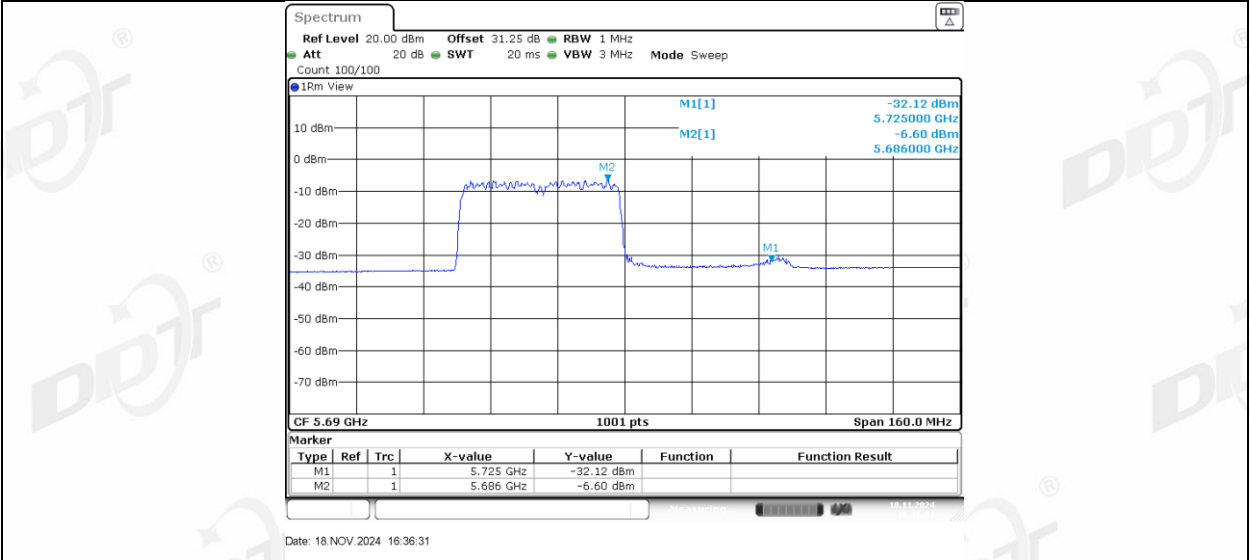
11AX80MIMO_Ant2_5690_UNII-2C_484Tone_RU66
