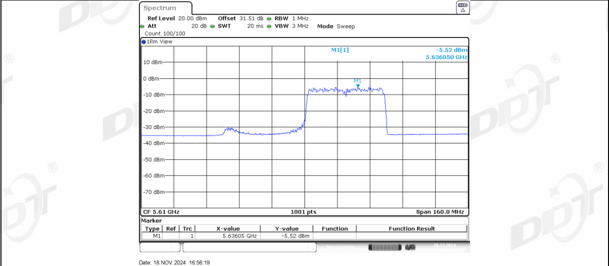
11AX80MIMO_Ant2_5610_484Tone_RU65
