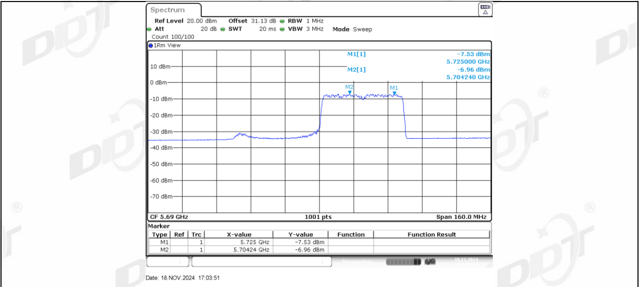
11AX80MIMO_Ant2_5690_UNII-2C_484Tone_RU65
