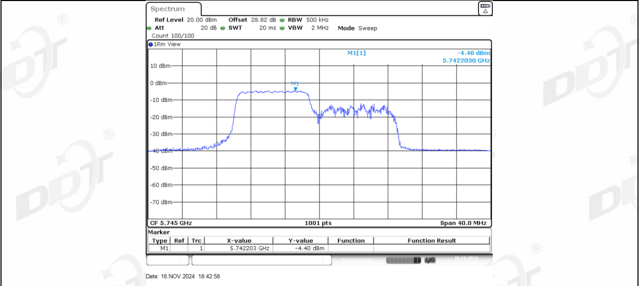
11AX20MIMO_Ant2_5745_106Tone_RU54
