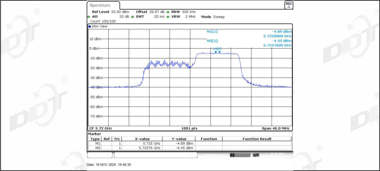
11AX20MIMO_Ant1_5745_26Tone_RU0
