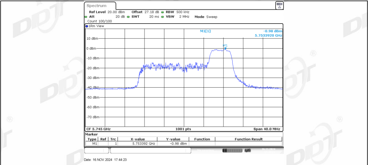
11AX20MIMO_Ant2_5745_106Tone_RU53
