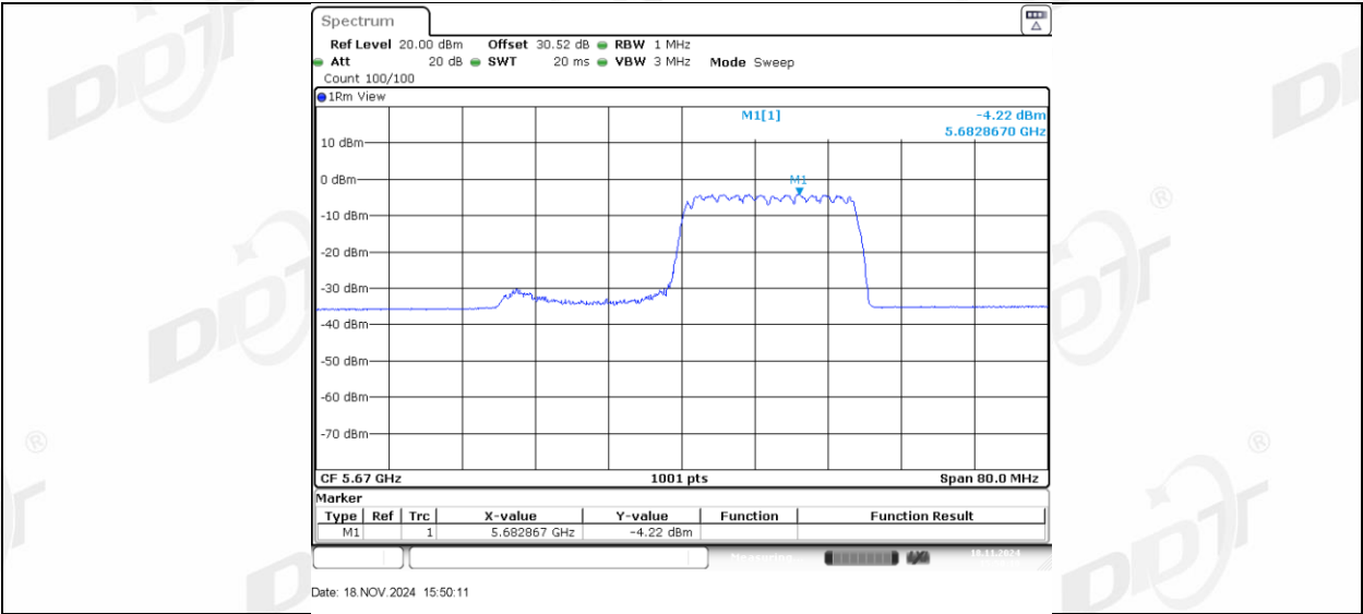
11AX40MIMO_Ant2_5670_242Tone_RU61
