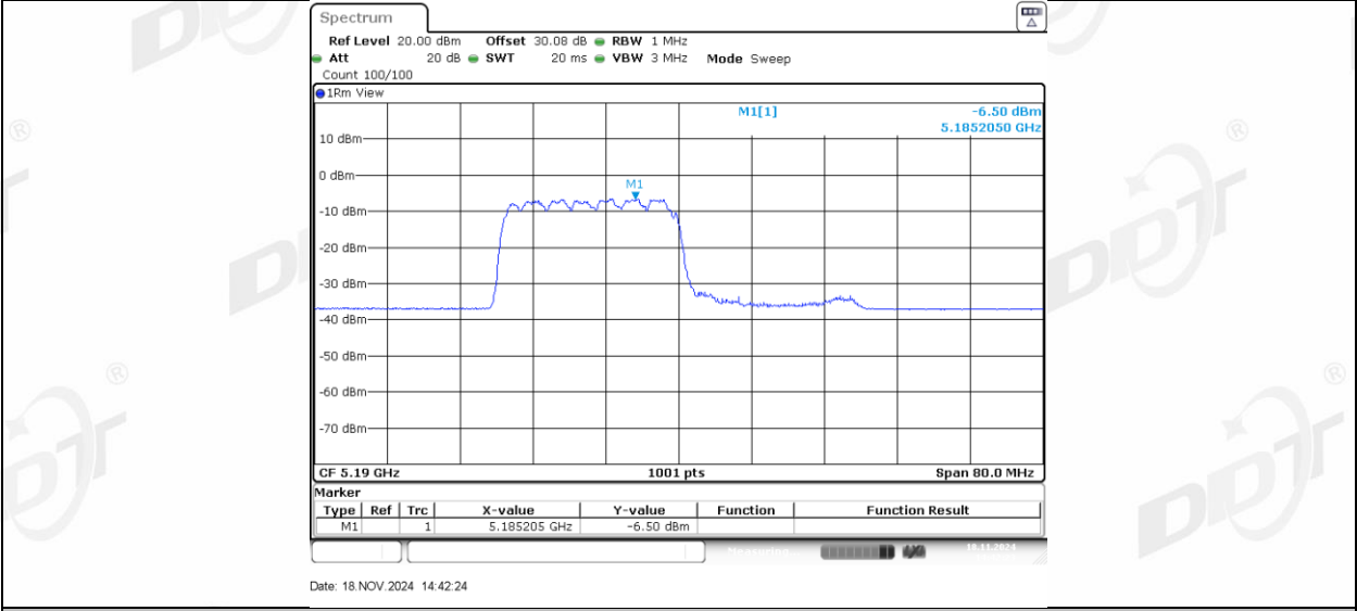
11AX40MIMO_Ant1_5190_242Tone_RU62
