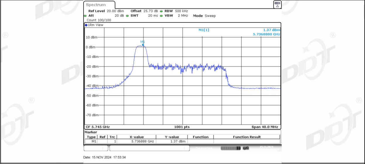
11AX20MIMO_Ant1_5745_26Tone_RU4
