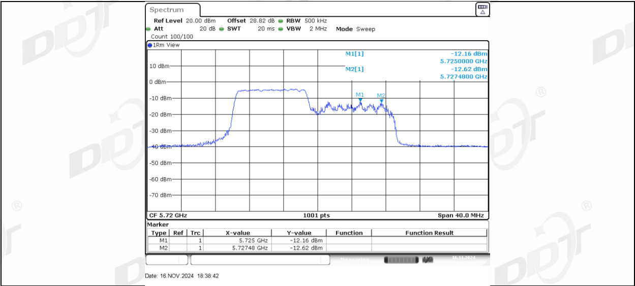
11AX20MIMO_Ant2_5720_UNII-3_106Tone_RU54
