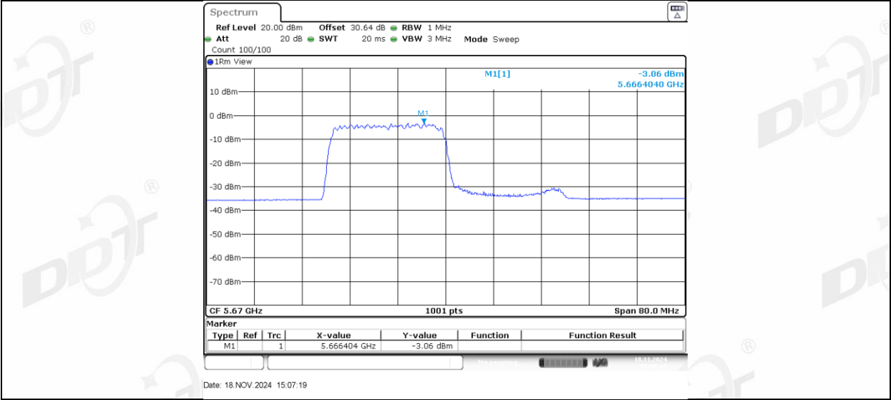
11AX40MIMO_Ant2_5670_242Tone_RU62
