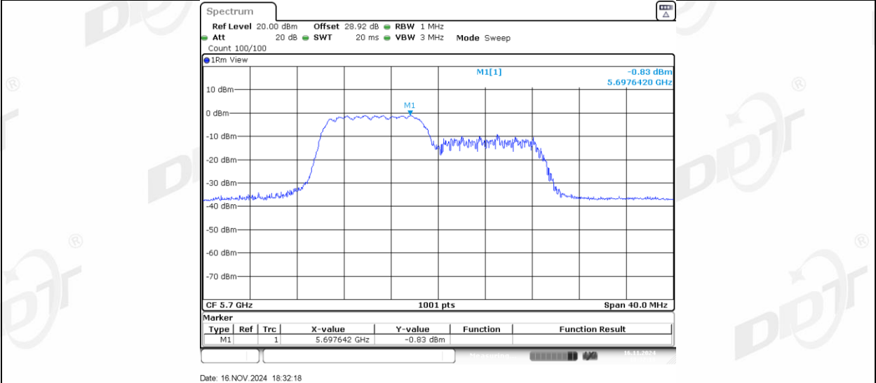
11AX20MIMO_Ant1_5700_106Tone_RU54
