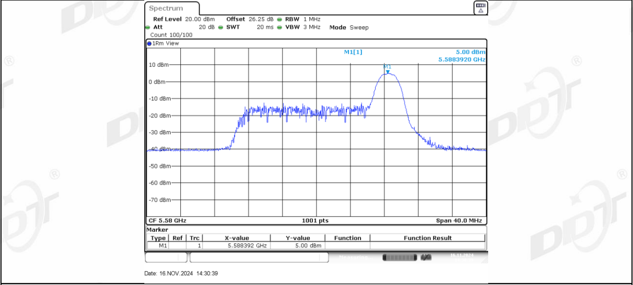
11AX20MIMO_Ant2_5580_52Tone_RU37
