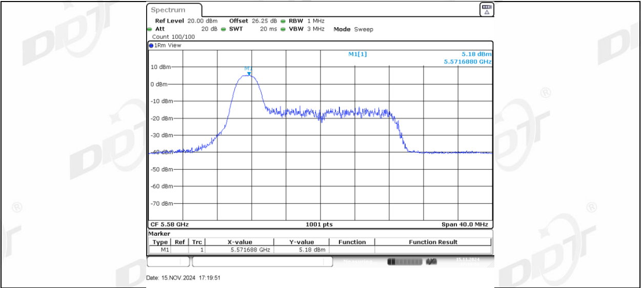
11AX20MIMO_Ant2_5580_26Tone_RU4
