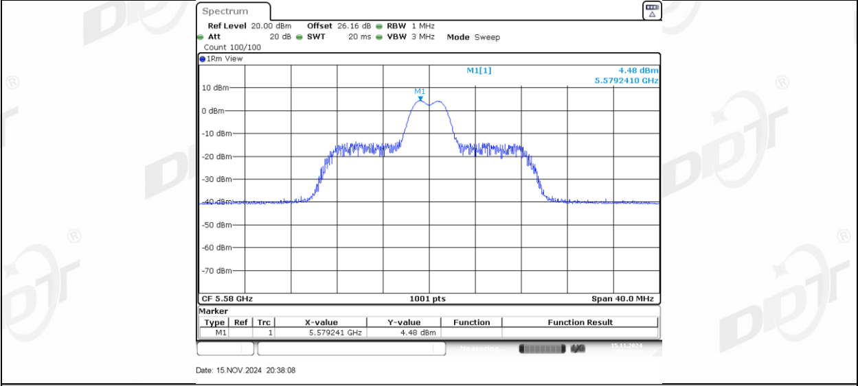
11AX20MIMO_Ant1_5580_26Tone_RU8
