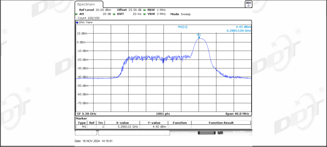
11AX20MIMO_Ant2_5280_52Tone_RU37
