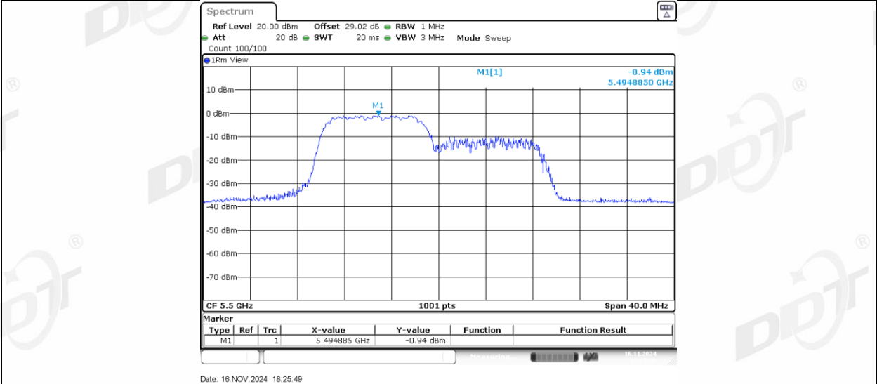
11AX20MIMO_Ant2_5500_106Tone_RU54
