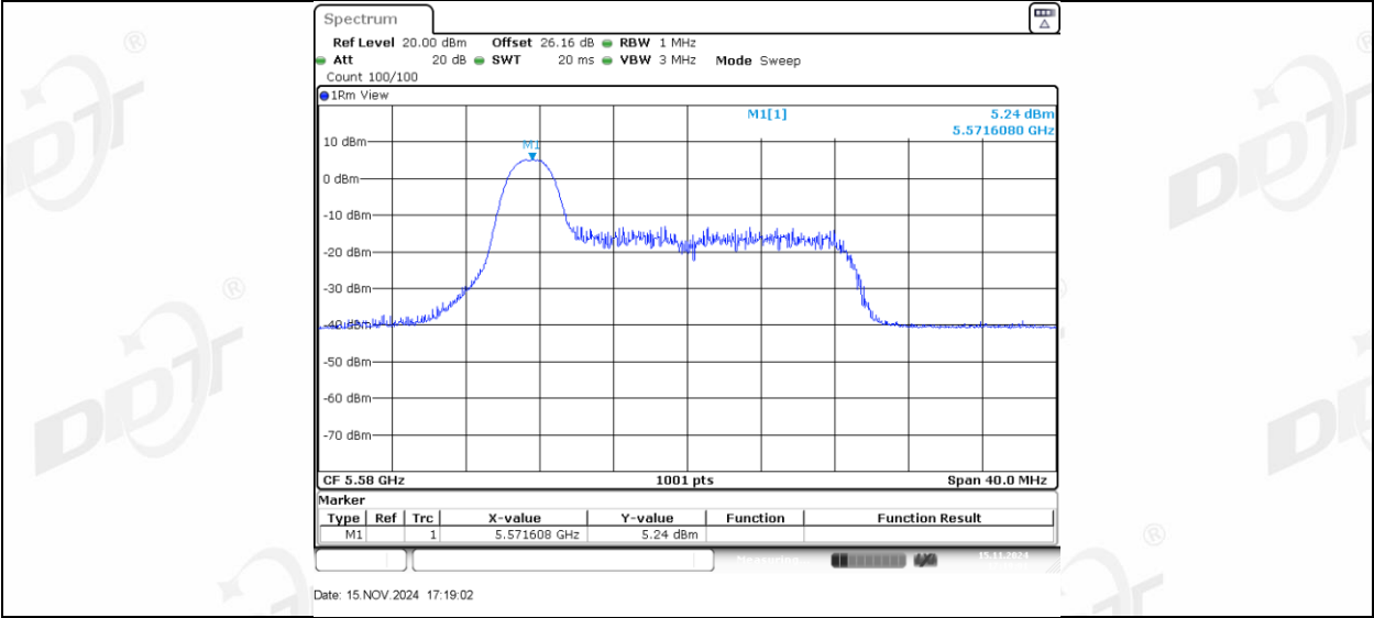
11AX20MIMO_Ant1_5580_26Tone_RU4
