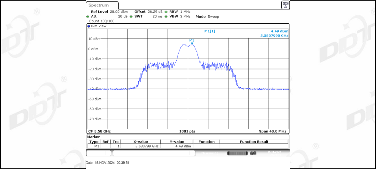
11AX20MIMO_Ant2_5580_26Tone_RU8
