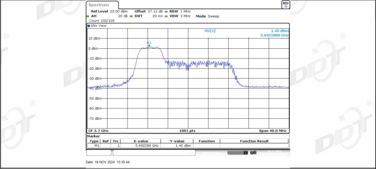
11AX20MIMO_Ant1_5700_52Tone_RU39
