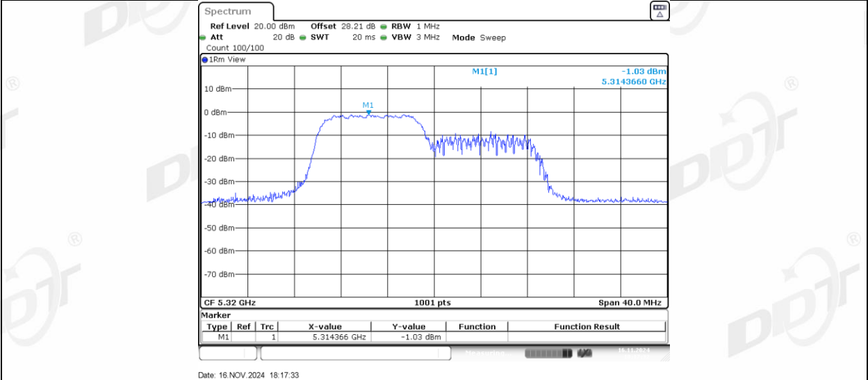
11AX20MIMO_Ant1_5320_106Tone_RU54
