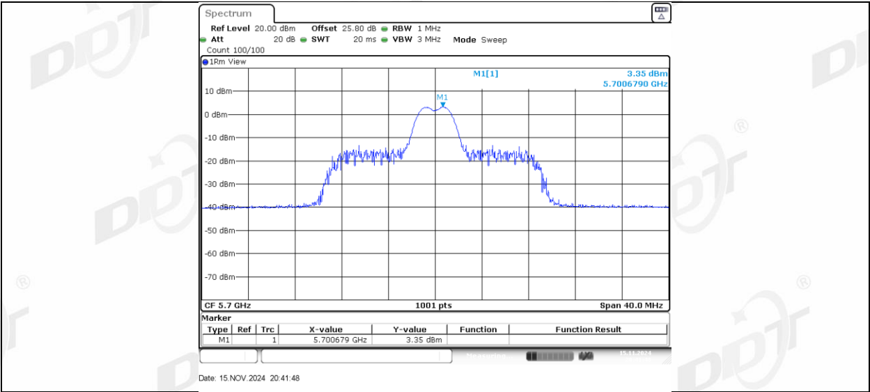
11AX20MIMO_Ant1_5700_26Tone_RU8
