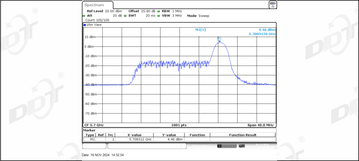
11AX20MIMO_Ant1_5700_52Tone_RU37
