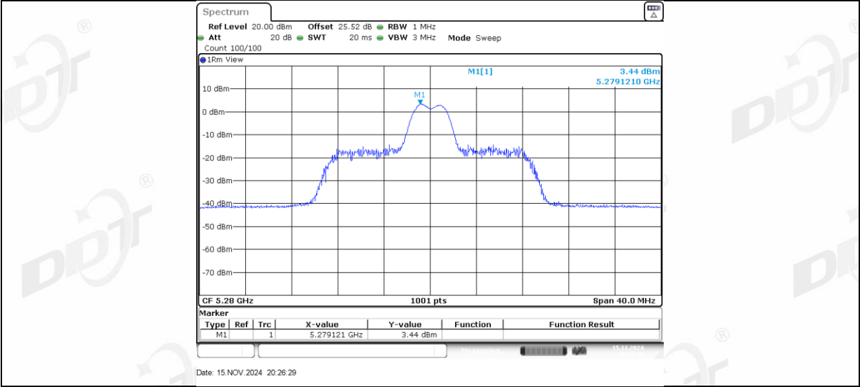
11AX20MIMO_Ant2_5280_26Tone_RU5
