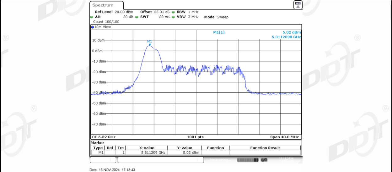
11AX20MIMO_Ant1_5320_26Tone_RU4
