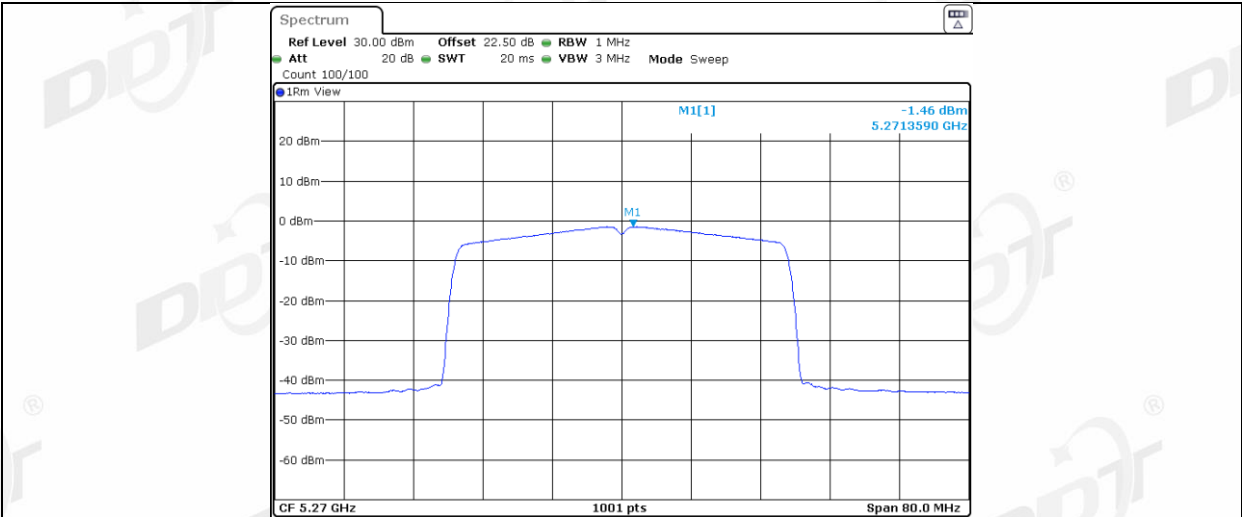
11AX40MIMO_Ant2_5270
