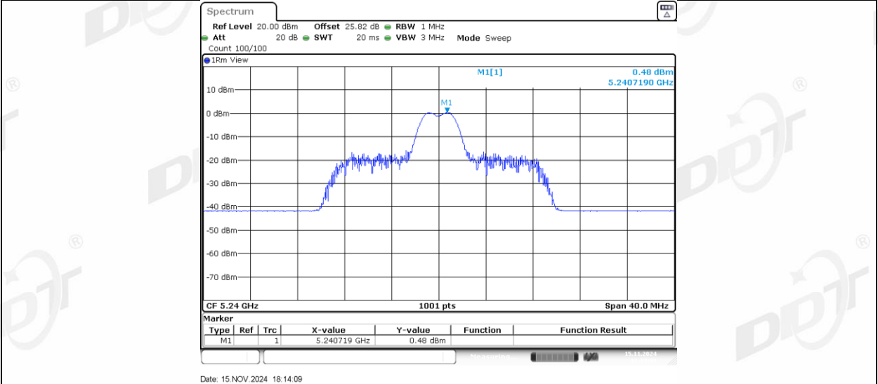
11AX20MIMO_Ant2_5240_26Tone_RU8
