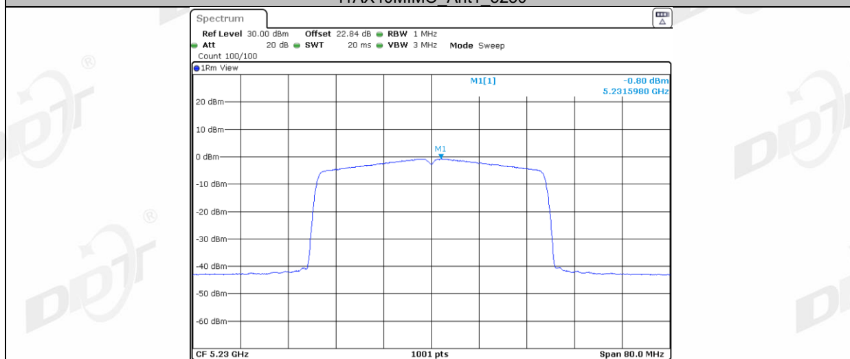
11AX40MIMO_Ant2_5230
