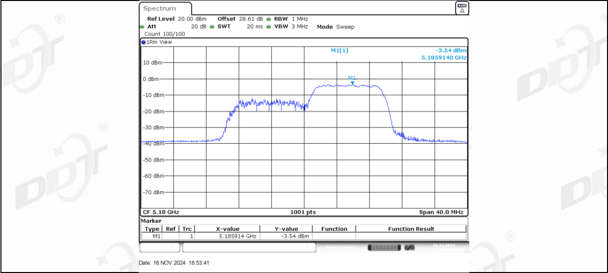
11AX20MIMO_Ant2_5180_26Tone_RU0
