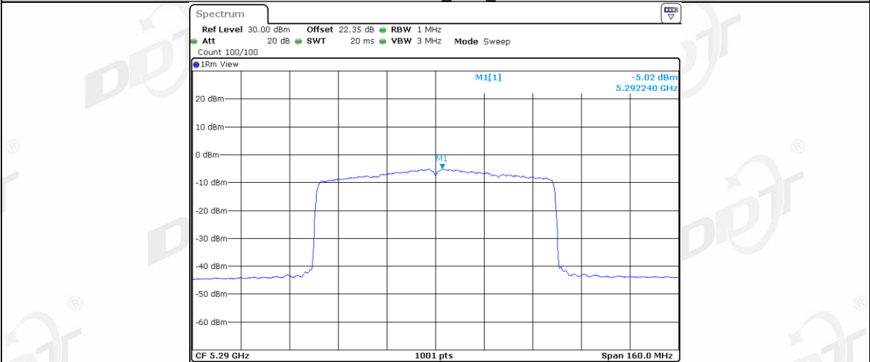
11AX80MIMO_Ant2_5290
