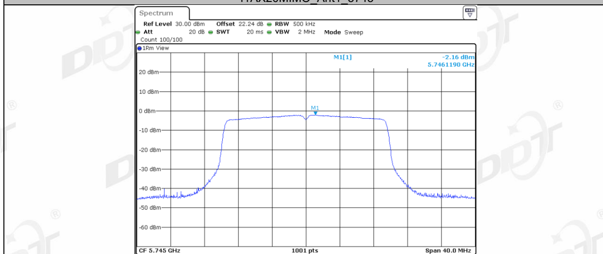
11AX20MIMO_Ant2_5745
