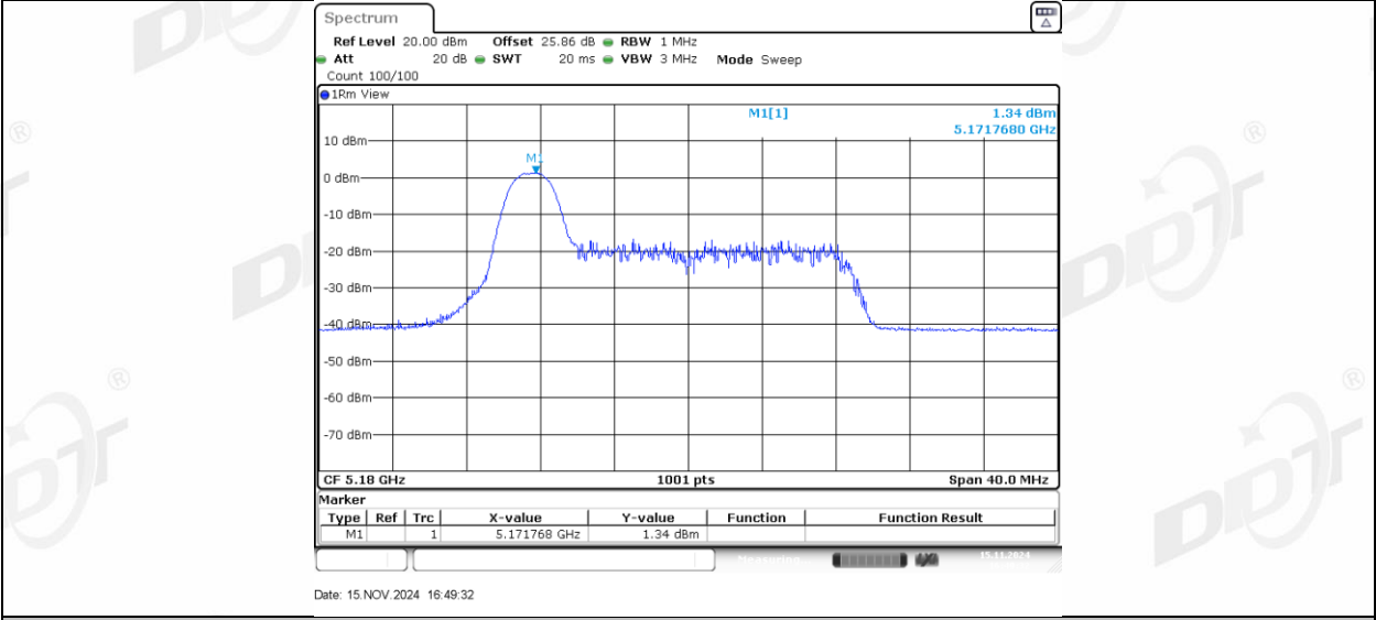
11AX20MIMO_Ant2_5180_26Tone_RU4
