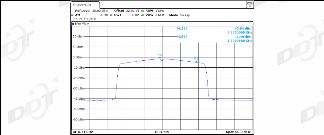
11AX40MIMO_Ant2_5710_UNII-2C
