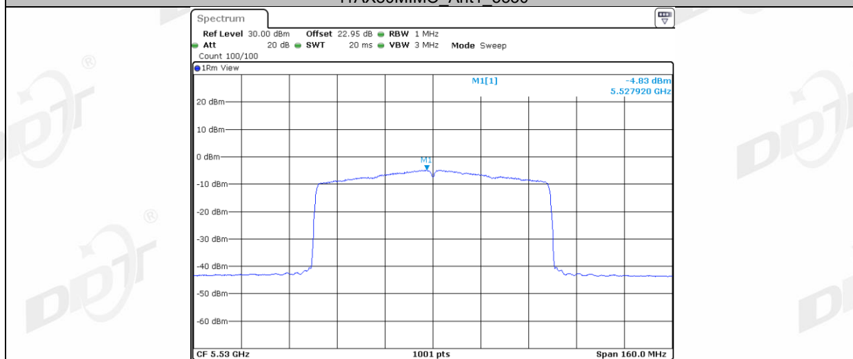
11AX80MIMO_Ant2_5530
