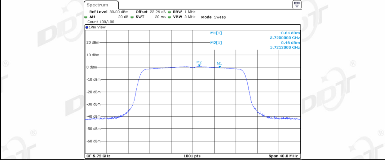
11AX20MIMO_Ant1_5720_UNII-3
