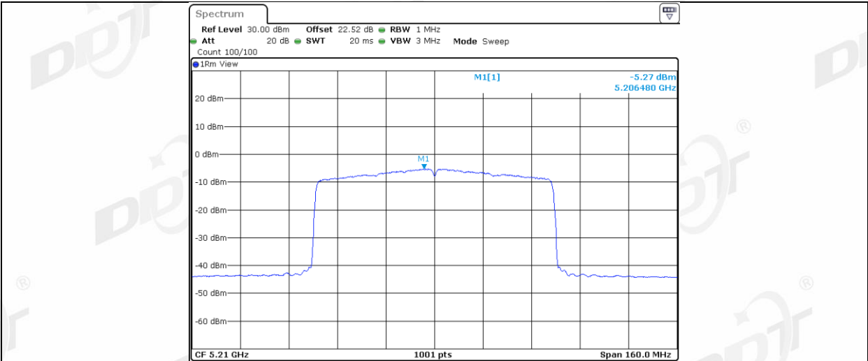
11AX80MIMO_Ant2_5210
