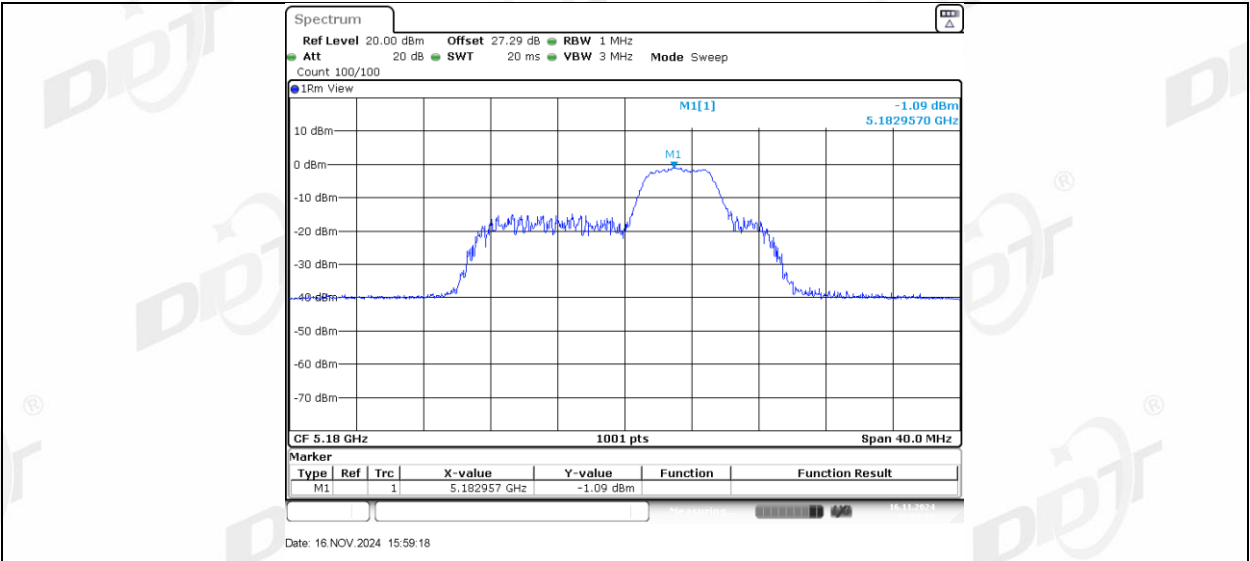
11AX20MIMO_Ant2_5180_52Tone_RU40
