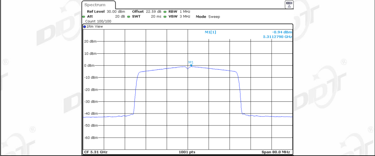
11AX40MIMO_Ant2_5310
