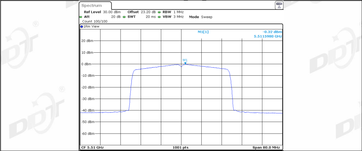
11AX40MIMO_Ant2_5510
