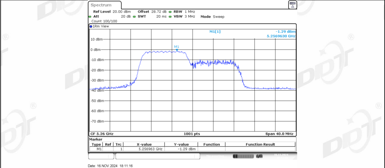
11AX20MIMO_Ant2_5260_106Tone_RU54
