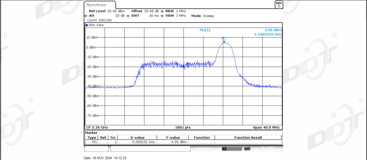
11AX20MIMO_Ant1_5260_52Tone_RU37
