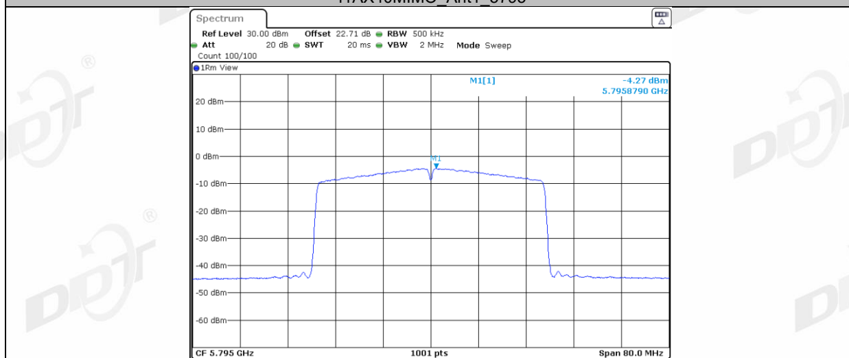
11AX40MIMO_Ant2_5795
