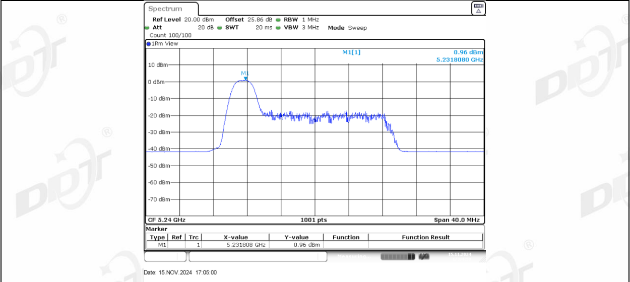
11AX20MIMO_Ant2_5240_26Tone_RU4
