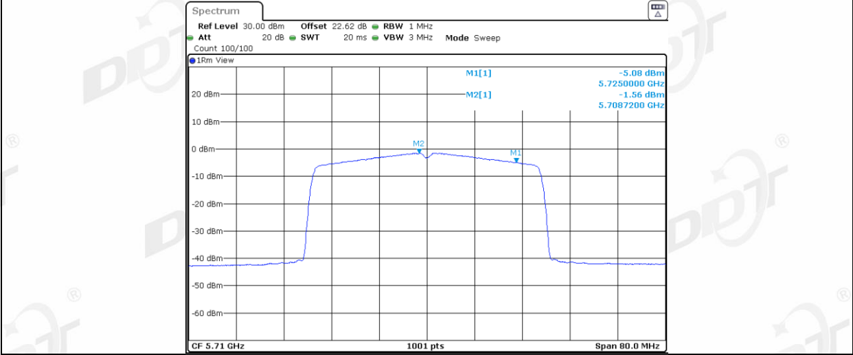
11AX40MIMO_Ant1_5710_UNII-3
