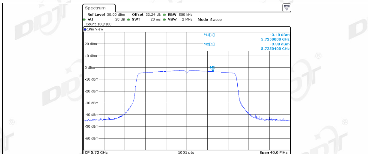
11AX20MIMO_Ant2_5720_UNII-3
