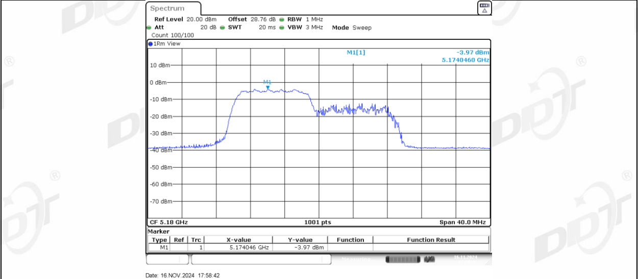
11AX20MIMO_Ant2_5180_106Tone_RU54
