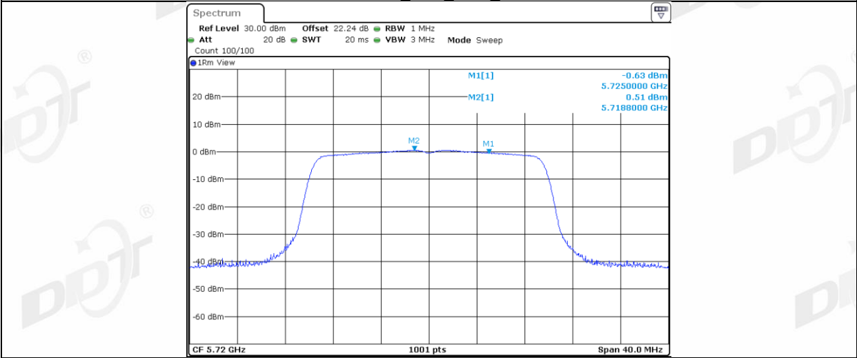
11AX20MIMO_Ant2_5720_UNII-2C
