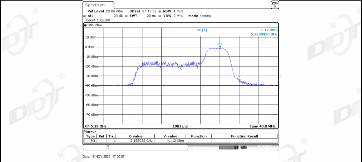
11AX20MIMO_Ant2_5180_106Tone_RU53
