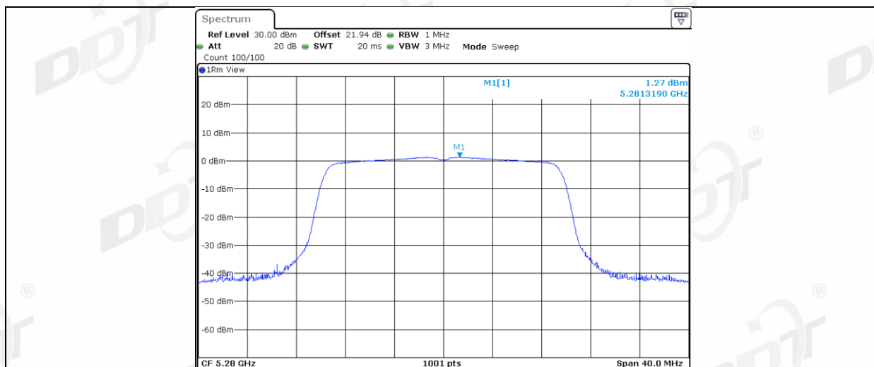
11AX20MIMO_Ant2_5280
