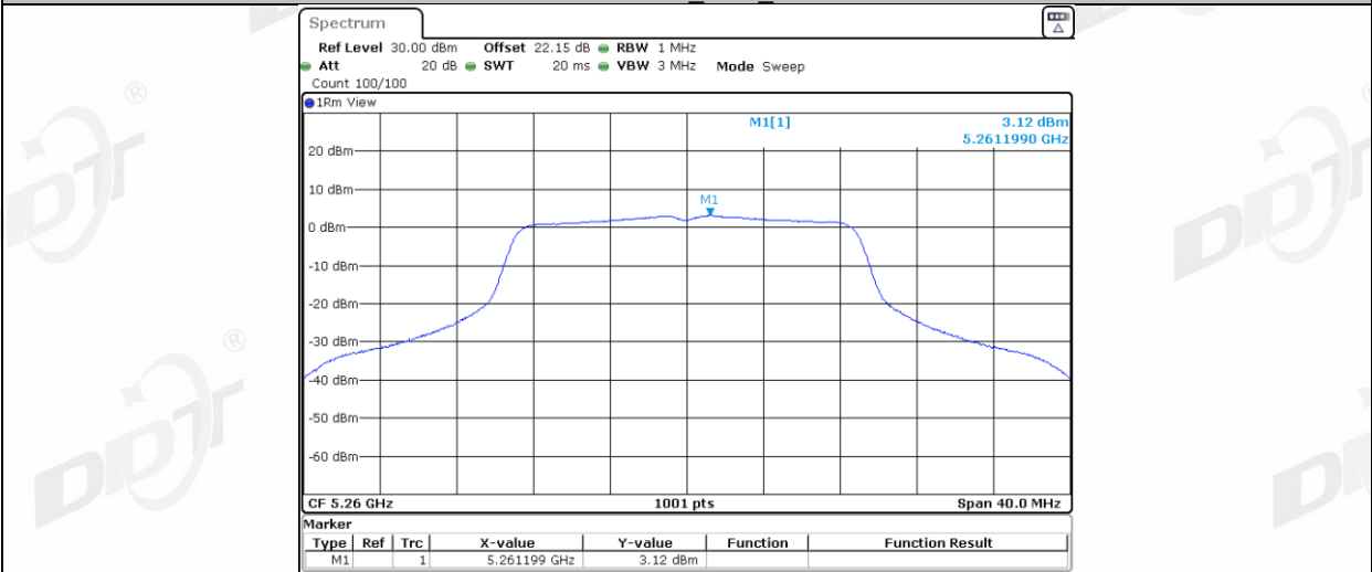
11N20MIMO_Ant2_5260
