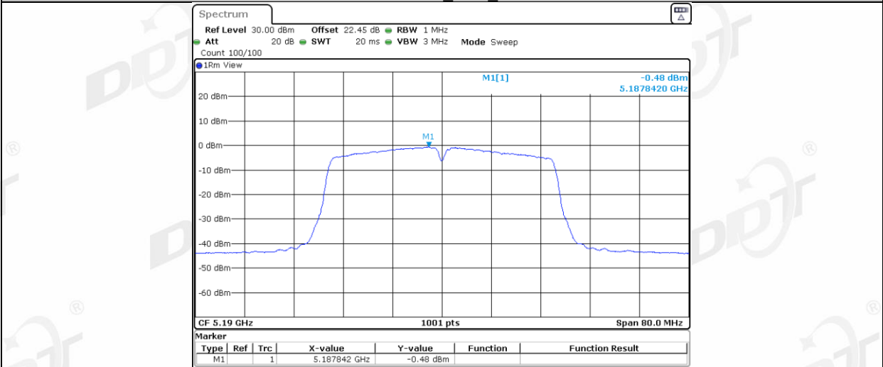
11N40MIMO_Ant2_5190
