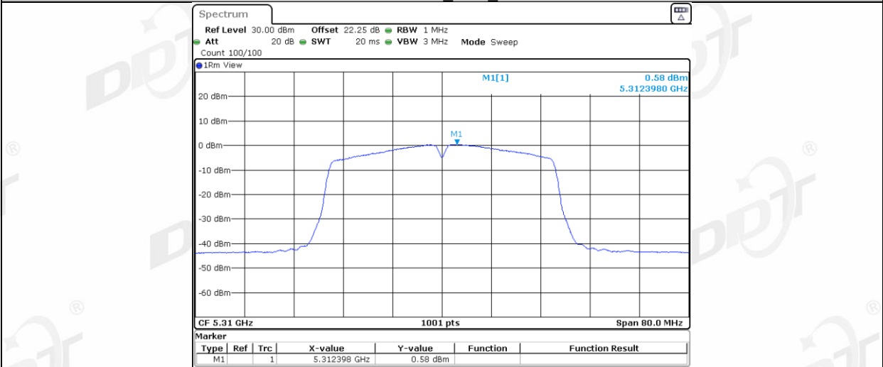
11N40MIMO_Ant2_5310
