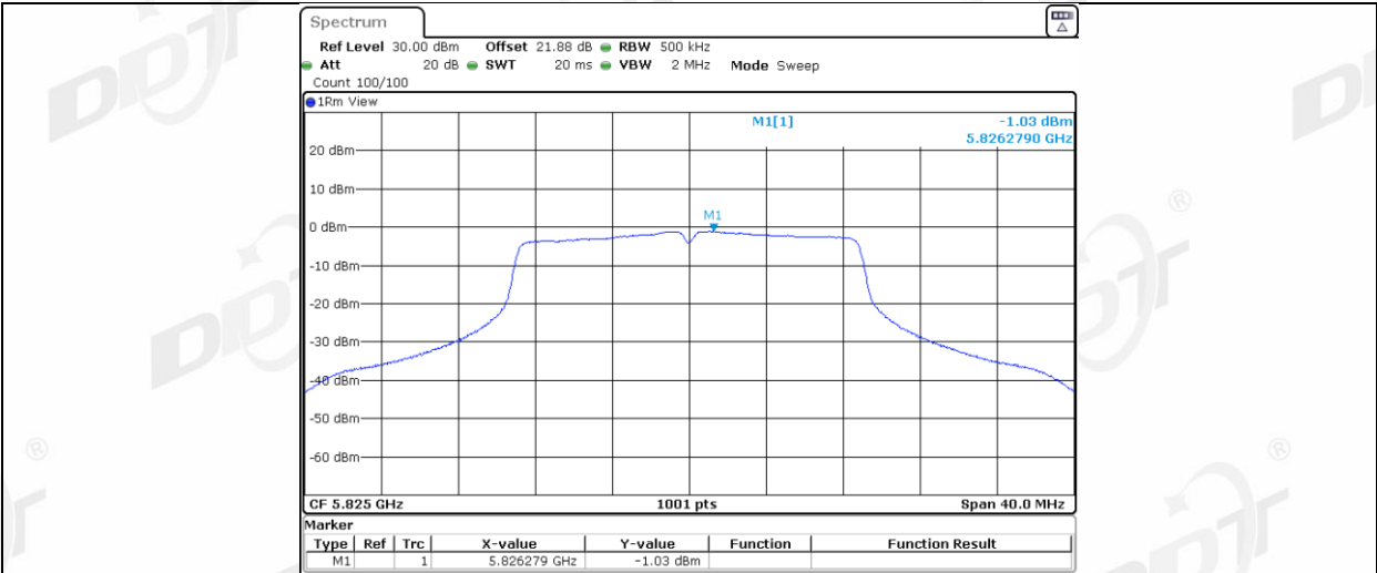
11N20MIMO_Ant2_5825
