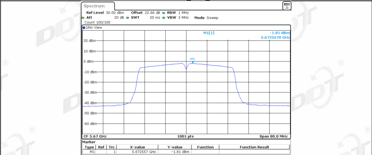
11N40MIMO_Ant2_5670
