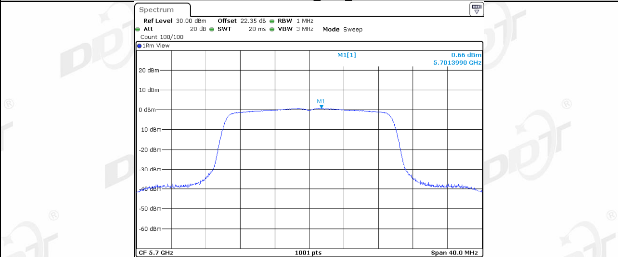
11AX20MIMO_Ant2_5700
