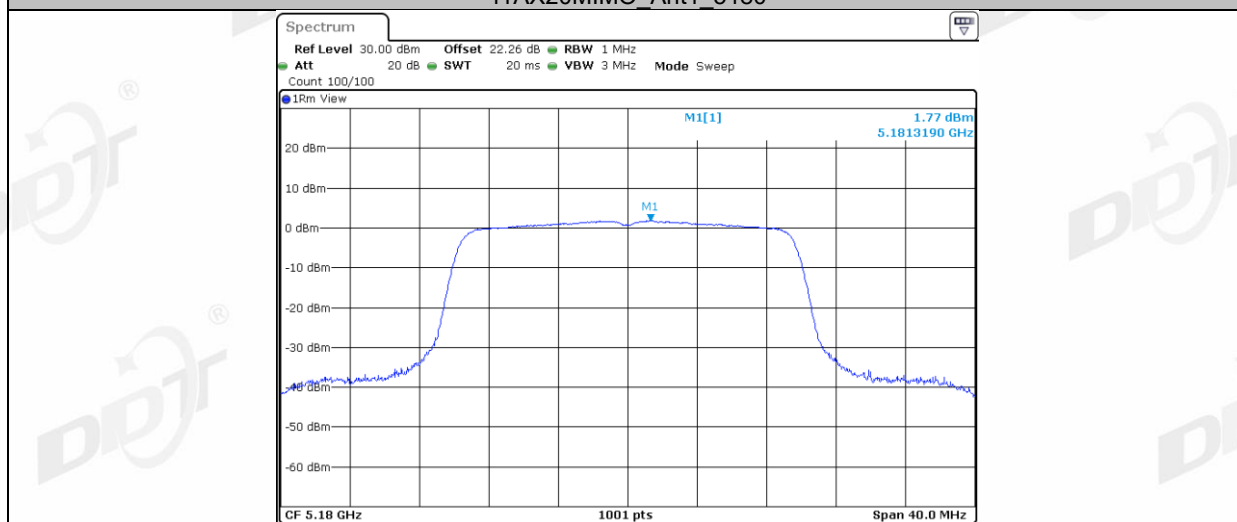
11AX20MIMO_Ant2_5180
