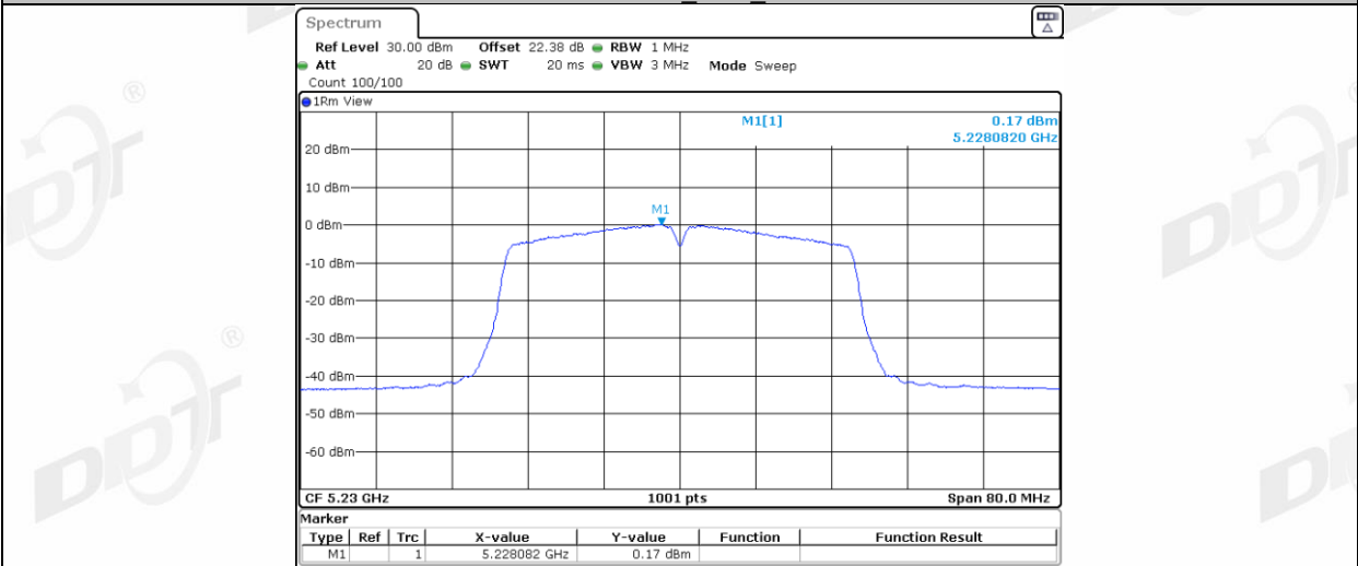
11N40MIMO_Ant2_5230
