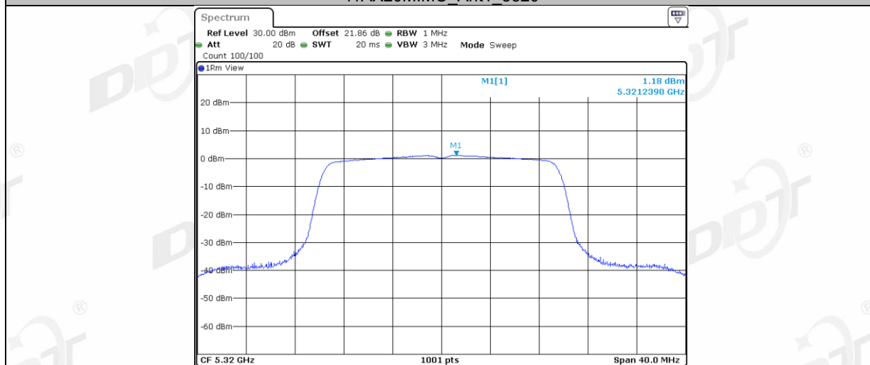
11AX20MIMO_Ant2_5320
