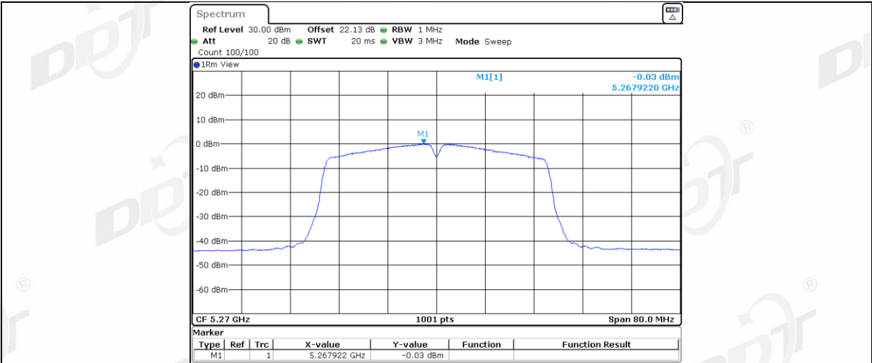
11N40MIMO_Ant2_5270
