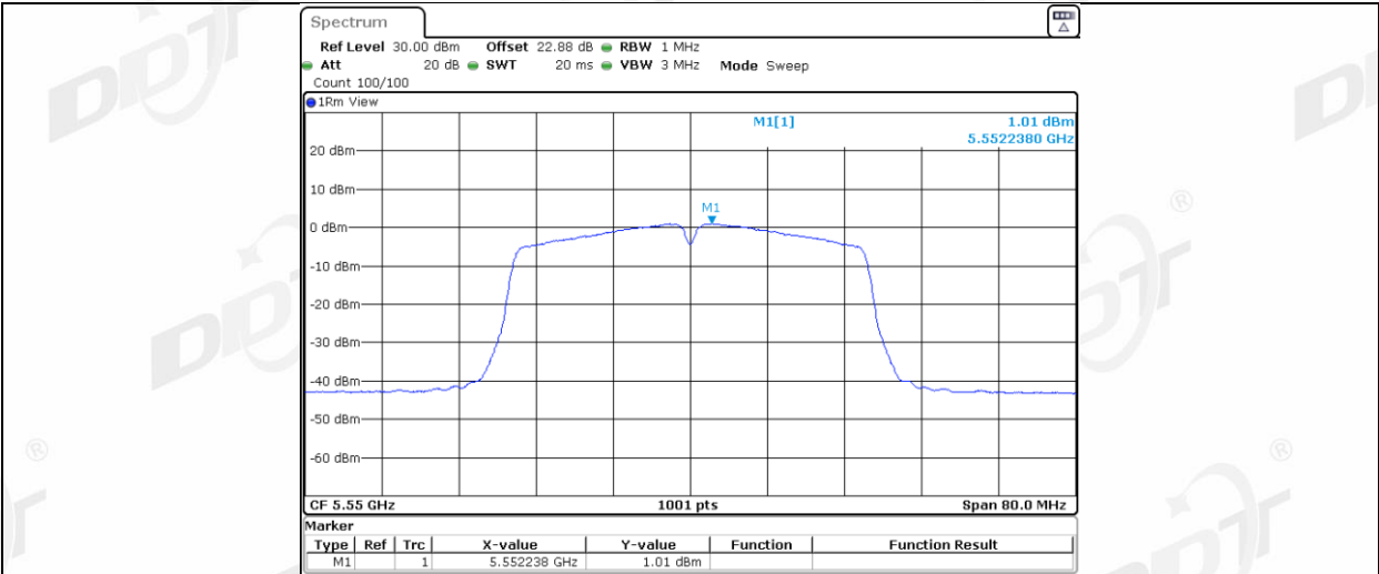
11N40MIMO_Ant2_5550
