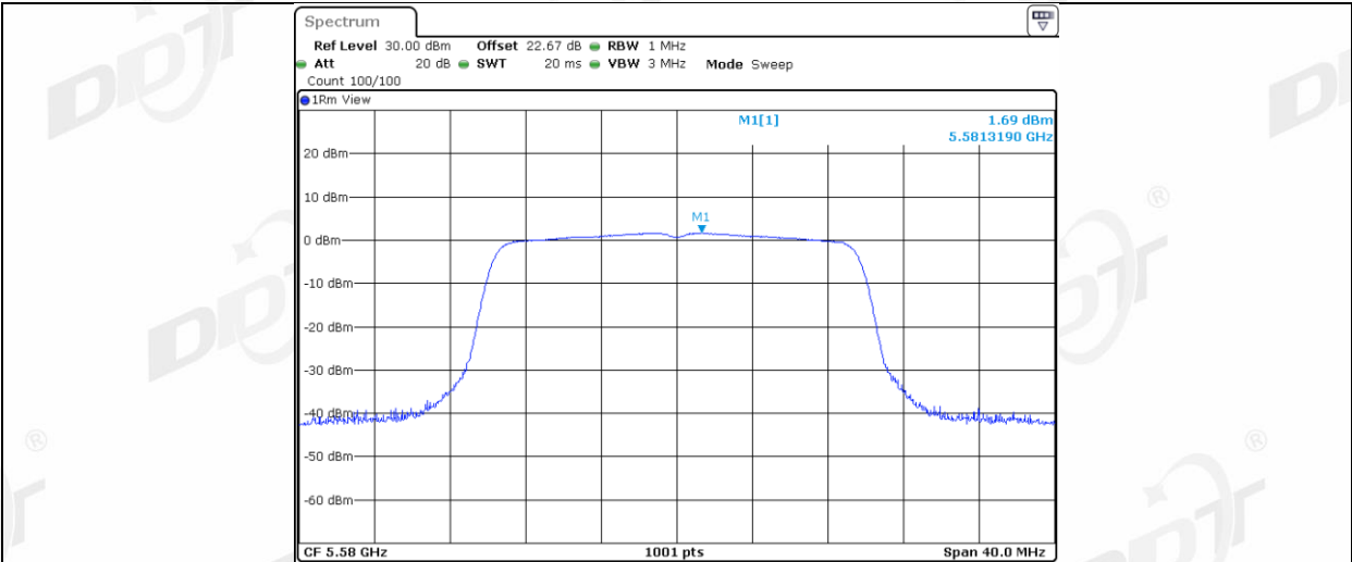
11AX20MIMO_Ant2_5580
