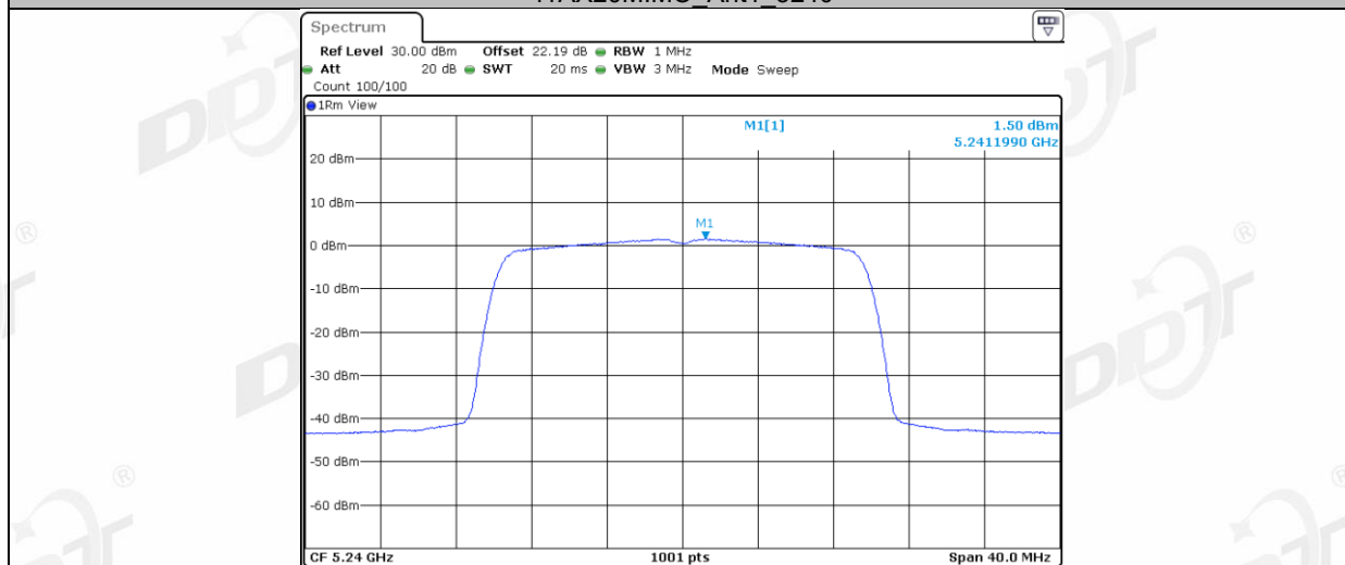
11AX20MIMO_Ant2_5240
