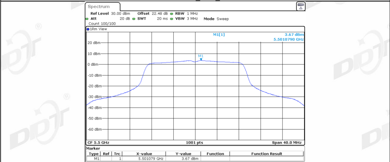
11N20MIMO_Ant2_5500
