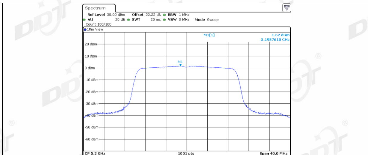
11AX20MIMO_Ant2_5200
