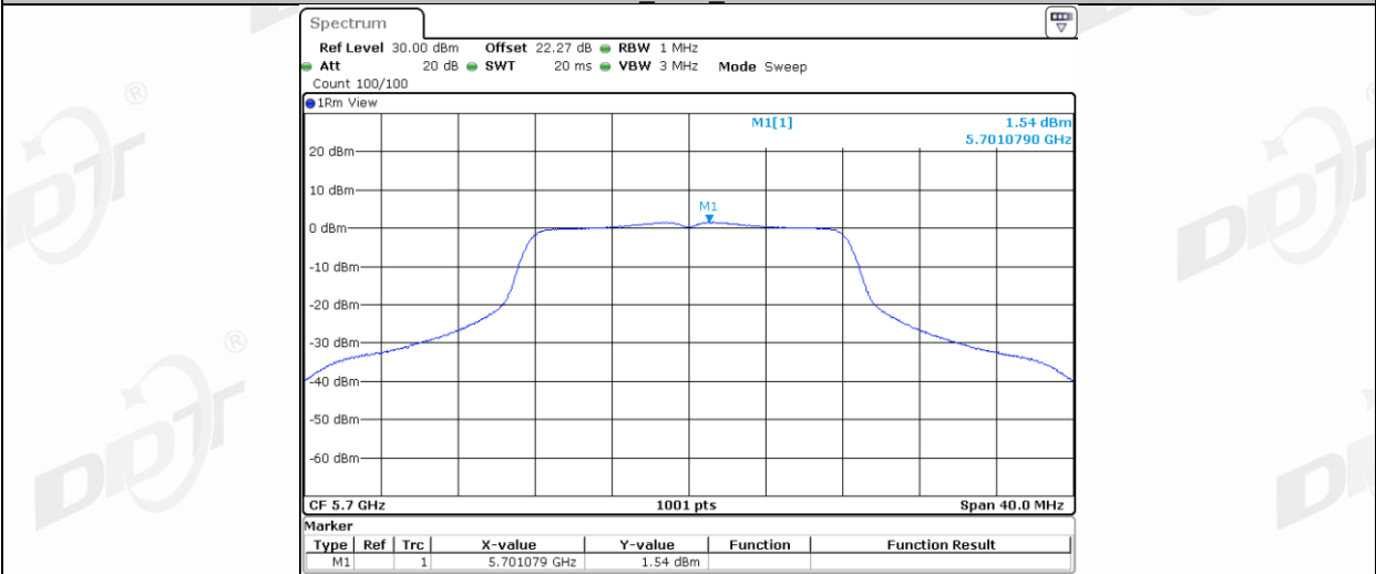
11A_Ant2_5700
