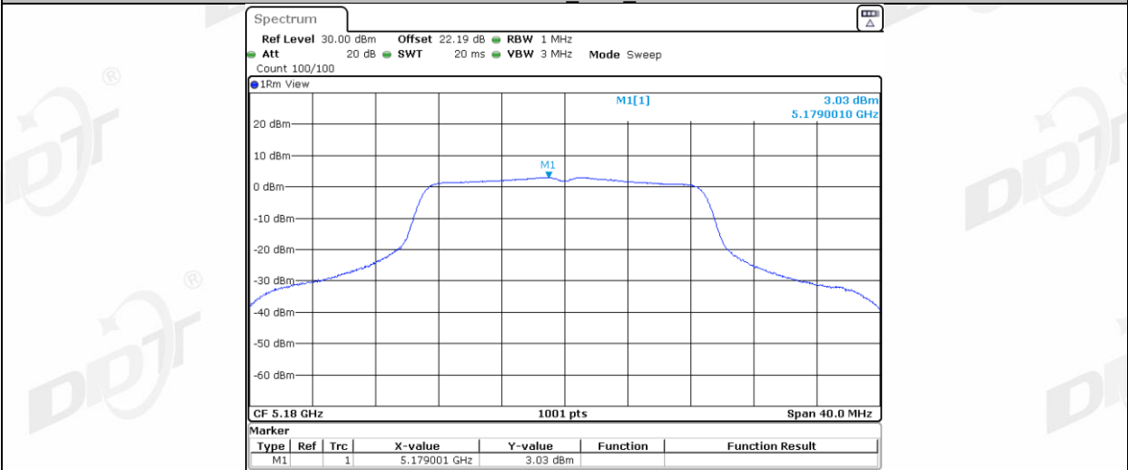
11N20MIMO_Ant2_5180
